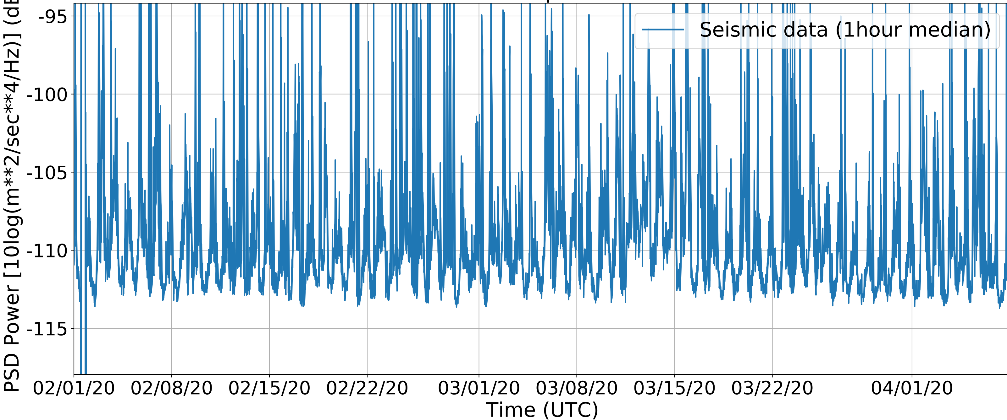
NP.1576.10.HNZ Bandpass filter: 5.0-20.0Hz
