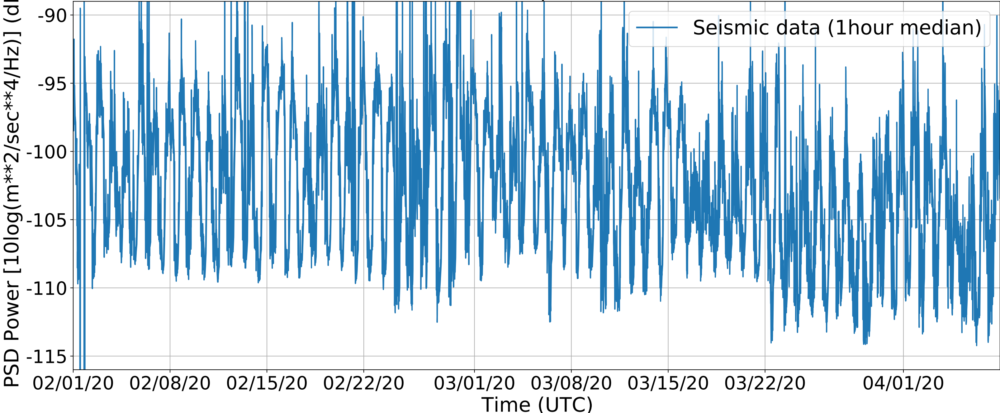
NP.1722.10.HNZ Bandpass filter: 5.0-20.0Hz
