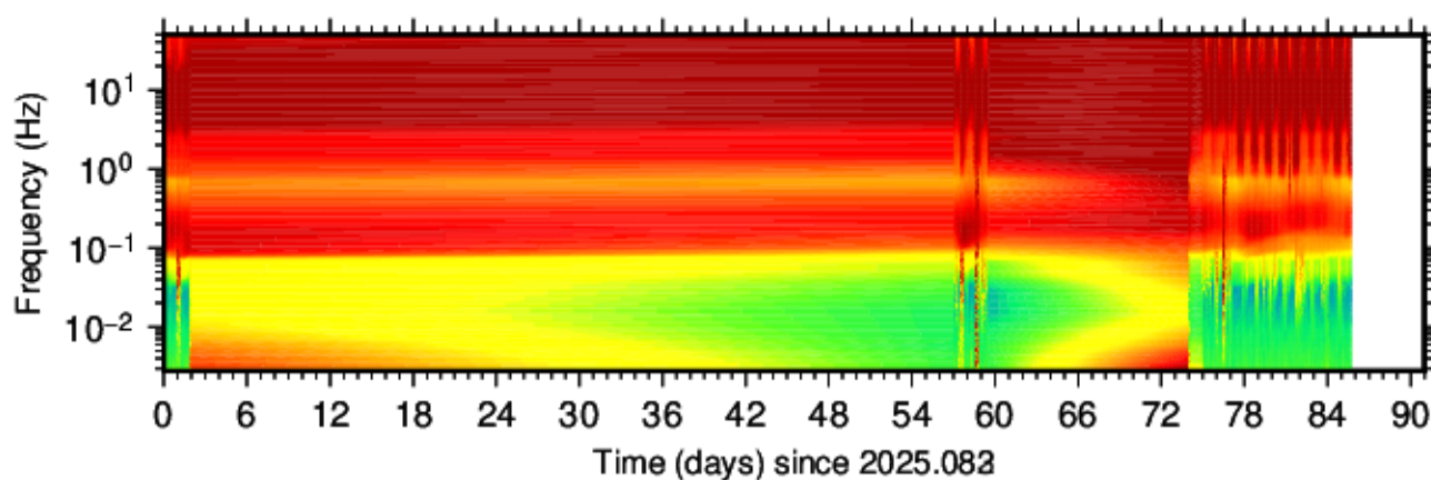
BK.BRIT.HHZ.00 (2025.083 - 2025.173)
