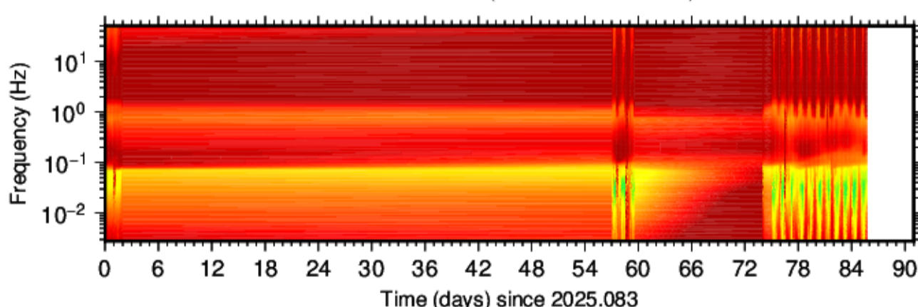
BK.BRIT.HHE.00 (2025.083 - 2025.173)
