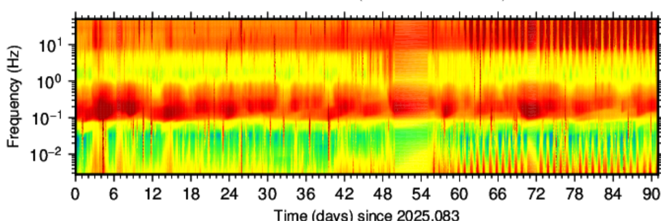
BK.GUMB.HHN.00 (2025.083 - 2025.173)
