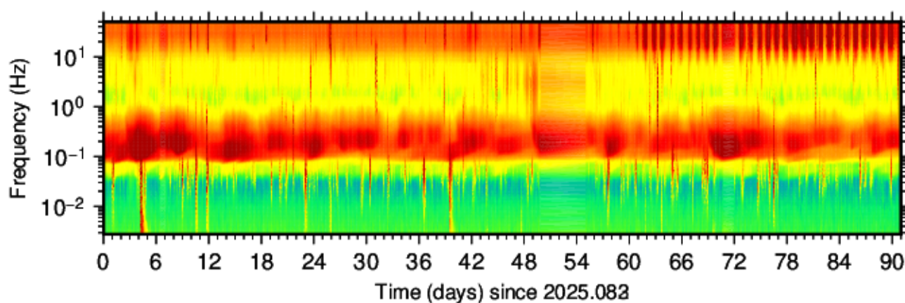
BK.GUMB.HHZ.00 (2025.083 - 2025.173)
