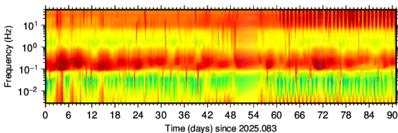
BK.GUMB.HHE.00 (2025.083 - 2025.173)
