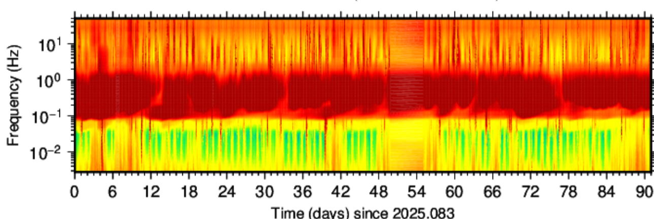
BK.HRCH.HHE.00 (2025.083 - 2025.173)
