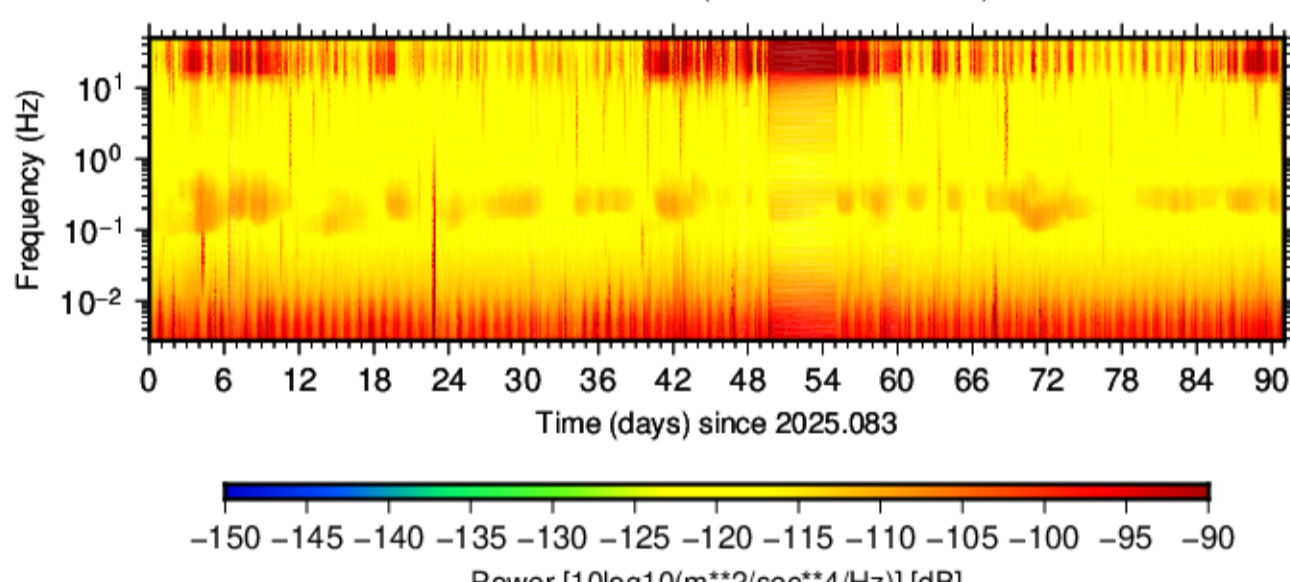
BK.PWOD.HNN.00 (2025.083 - 2025.173)
