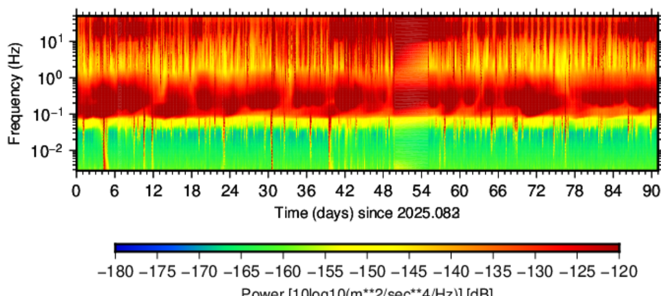
BK.PWOD.HHZ.00 (2025.083 - 2025.173)
