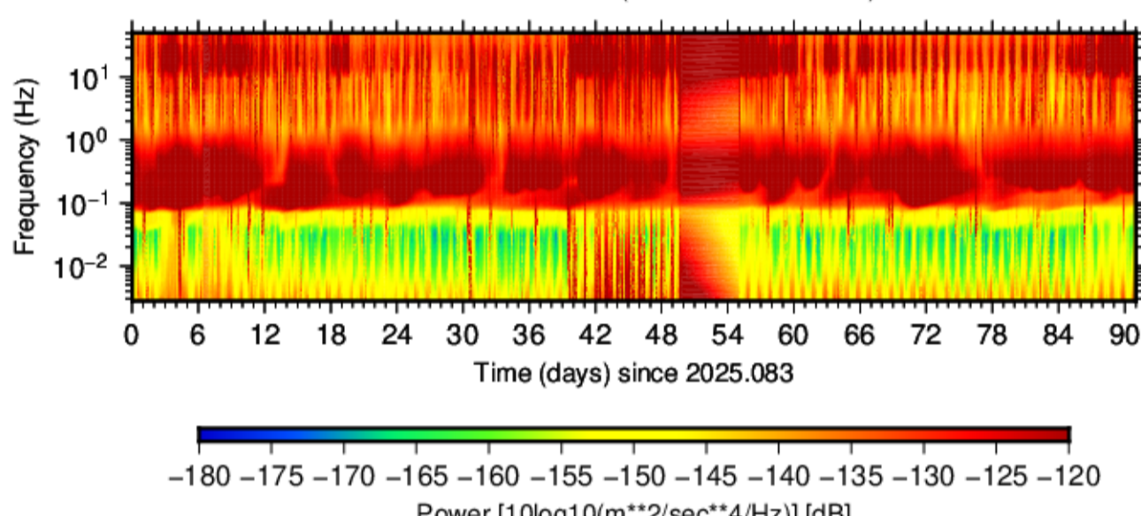
BK.PWOD.HHN.00 (2025.083 - 2025.173)
