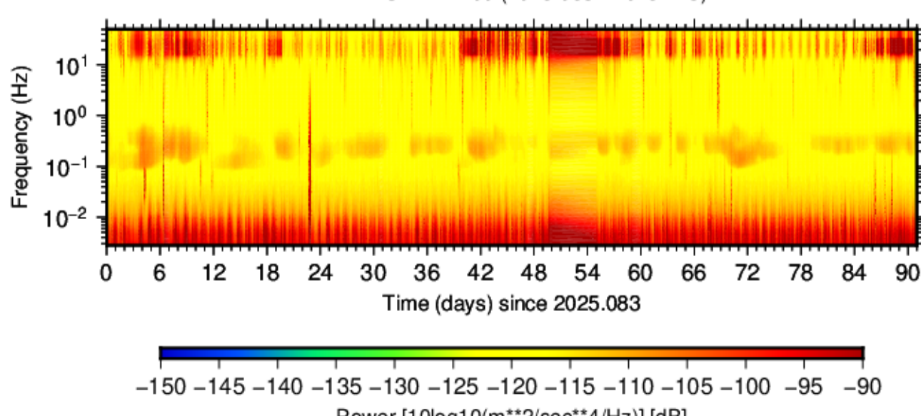
BK.PWOD.HNE.00 (2025.083 - 2025.173)
