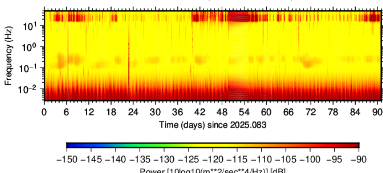
BK.PWOD.HNZ.00 (2025.083 - 2025.173)
