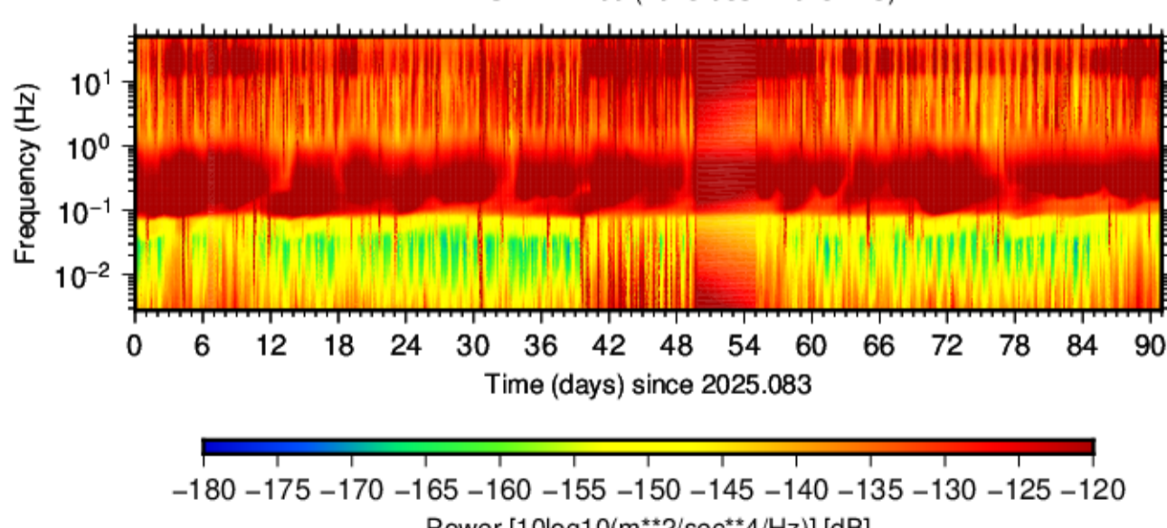
BK.PWOD.HHE.00 (2025.083 - 2025.173)
