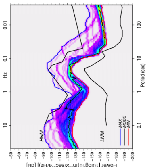
BK BAYL 00 HHZ 138 PSDs : 2025:250 - 2025:255
