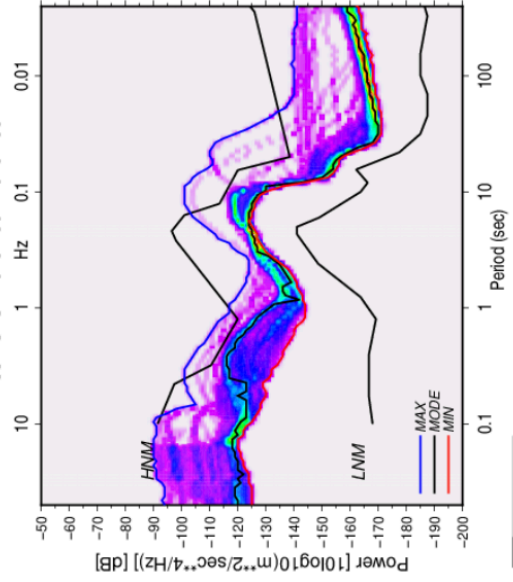
BK AVSP 00 HHZ 138 PSDs : 2025:250 - 2025:255
