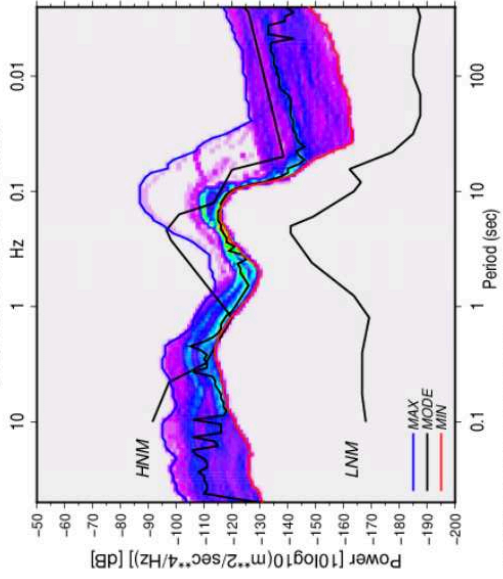
BK WHCL 00 HHE 138 PSDs : 2025:250 - 2025:255
