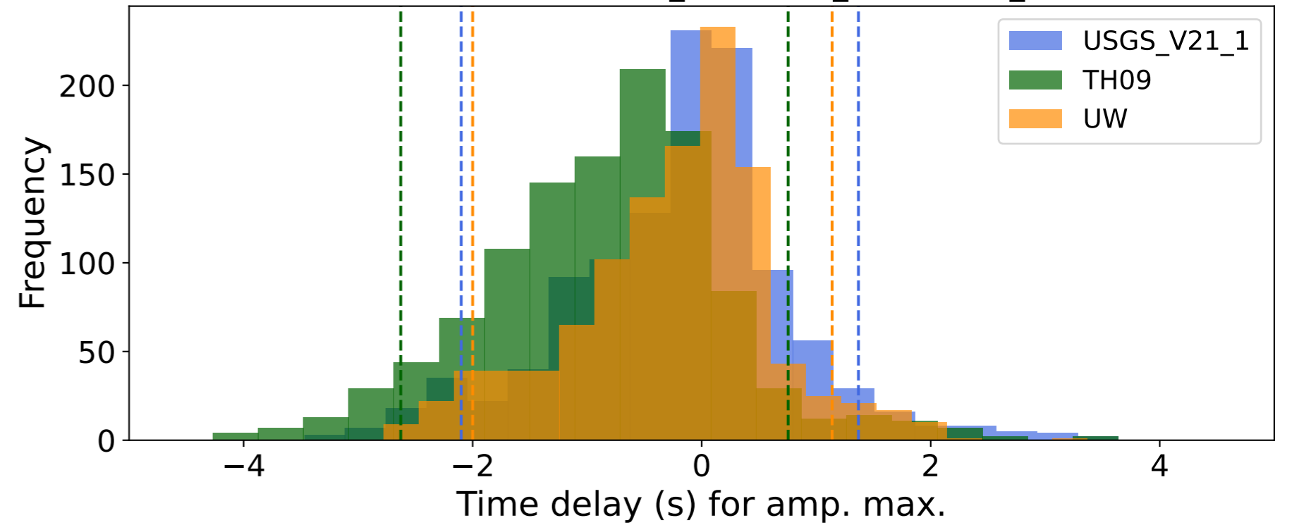
EventALL (0.16-0.5Hz) corr_tw:5s corr_com:T corr_min:0.8
