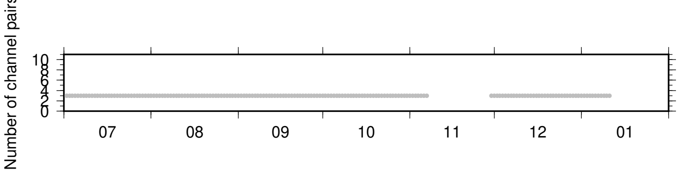
BK_PRDS_NC_KSM ZRT 0.10-0.90Hz 011
