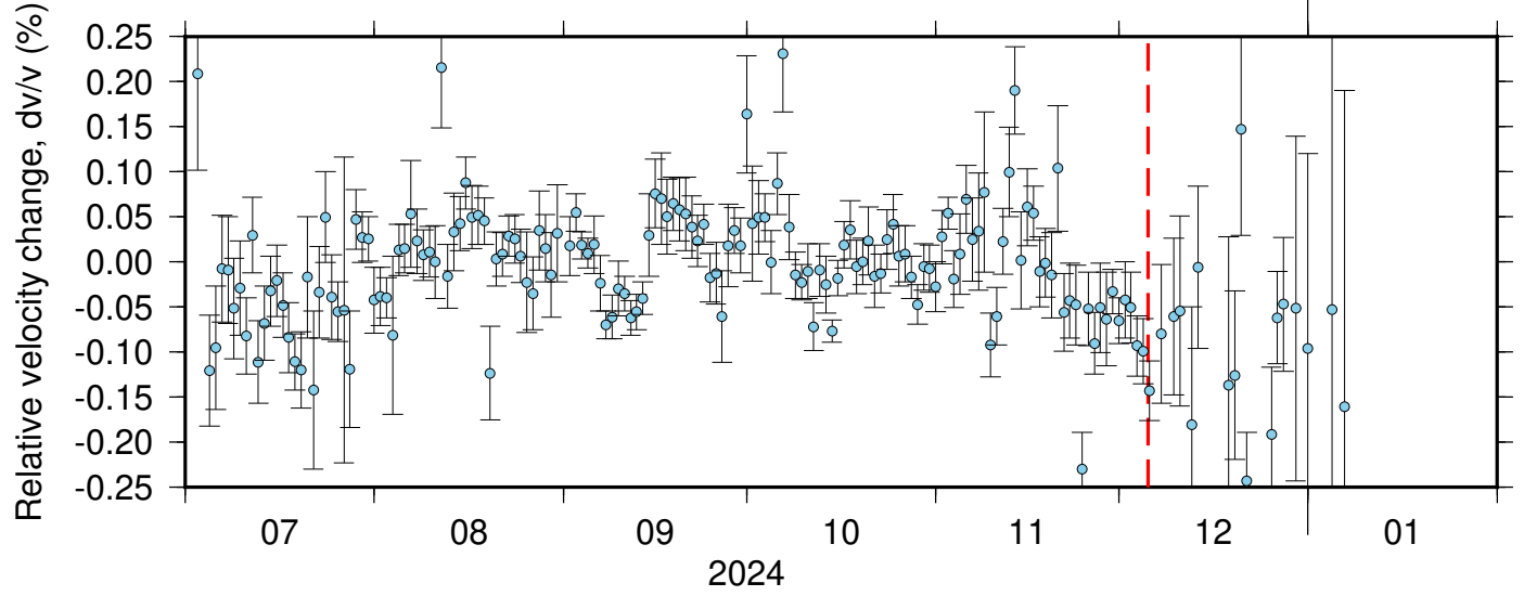
BK_PETL_BK_RBOW ZRT 0.10-0.90Hz 011
