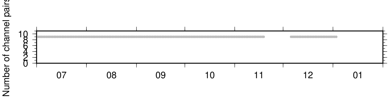
BK_GHOP_PB_B049 ZRT 0.10-0.90Hz 011
