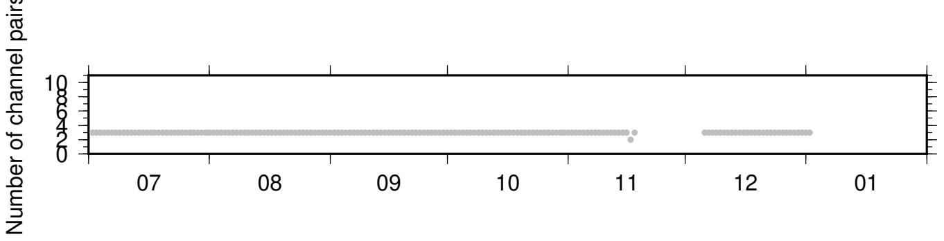
NC_KPR_PB_B049 ZRT 0.10-0.90Hz 011
