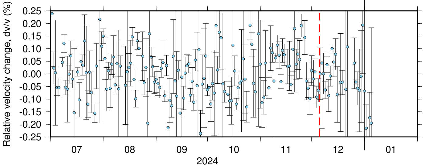
BK_HAYF_BK_WLKR ZRT 0.10-0.90Hz 011
