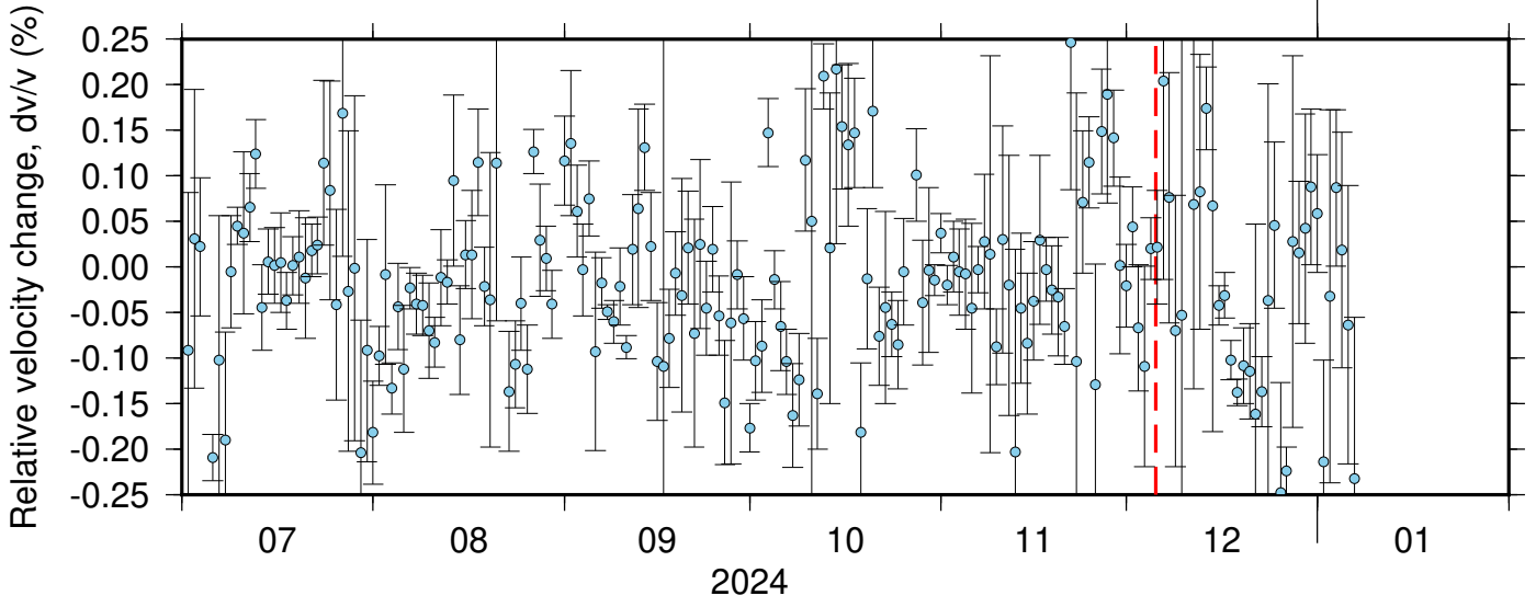
BK_HAYF_NC_KMR ZRT 0.10-0.90Hz 011
