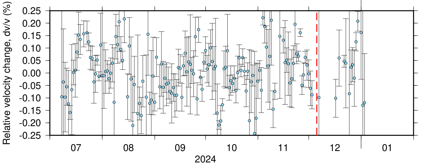
BK_RBOW_NC_KCR ZRT 0.10-0.90Hz 011
