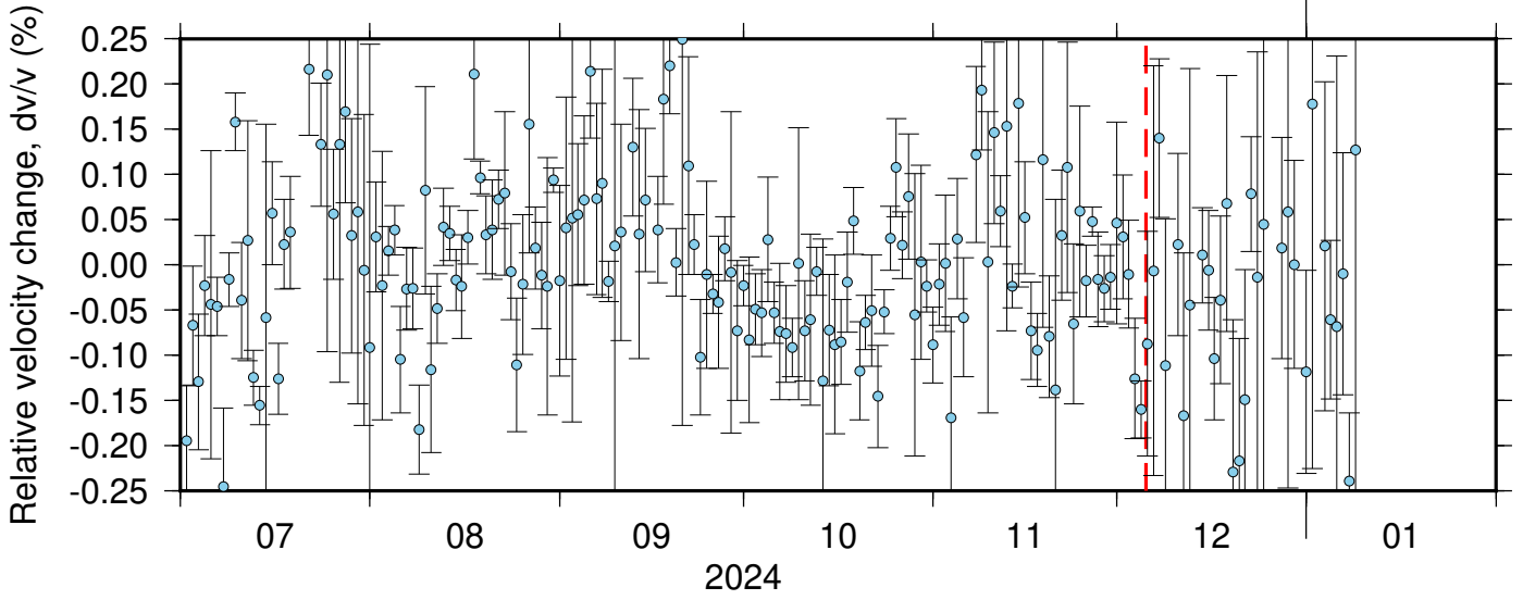
BK_HAYF_BK_SPRL ZRT 0.10-0.90Hz 011
