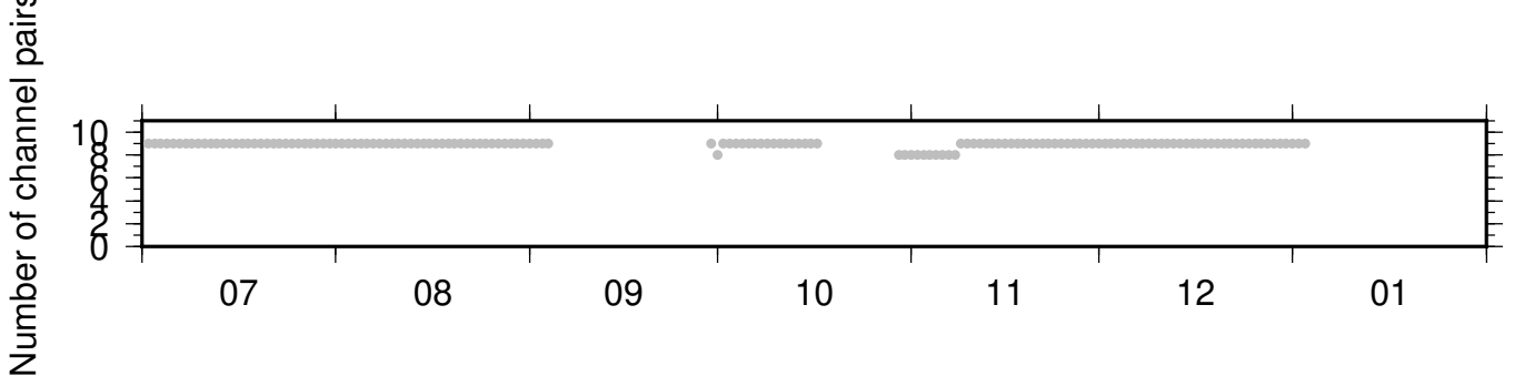
BK_RBOW_PB_B046 ZRT 0.10-0.90Hz 011
