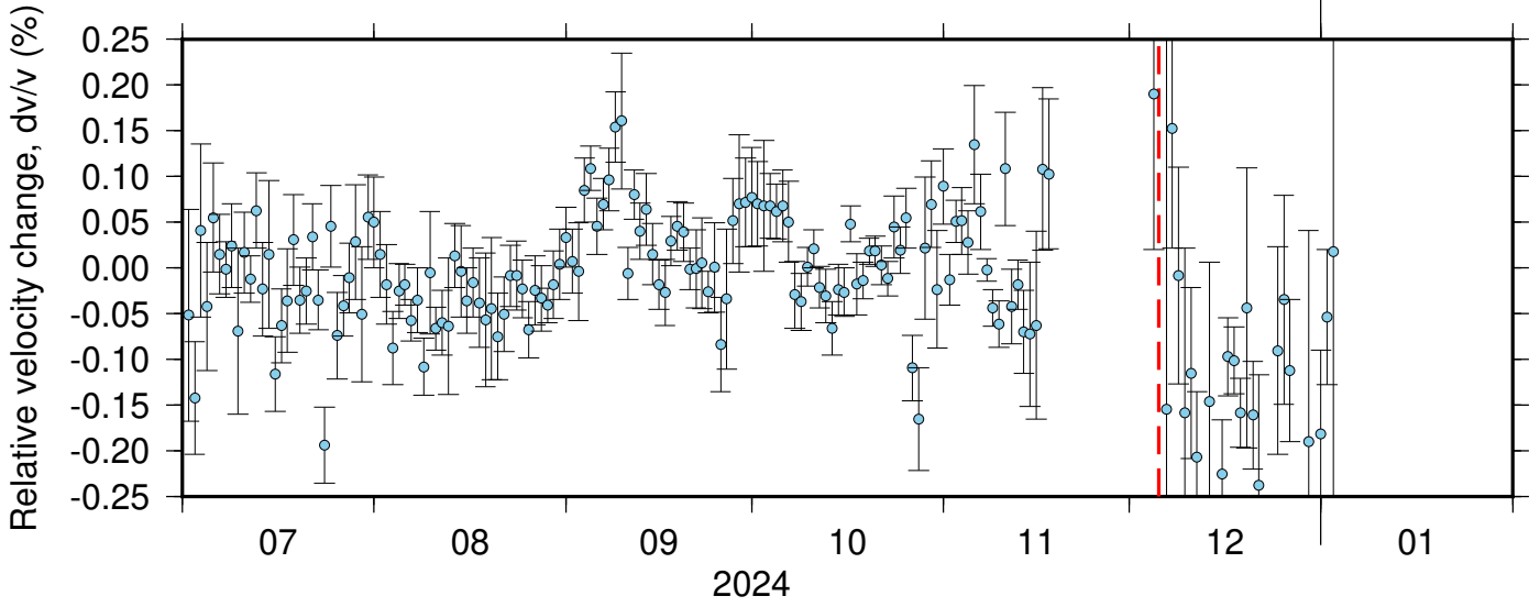
NC_KMPB_PB_B049 ZRT 0.10-0.90Hz 011
