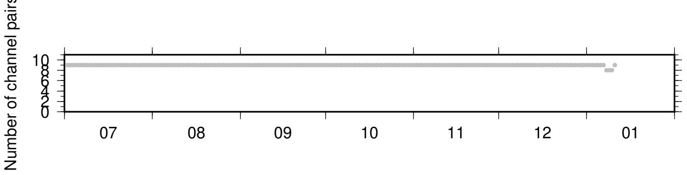
BK_PETL_BK_RBOW ZRT 0.10-0.90Hz 011
