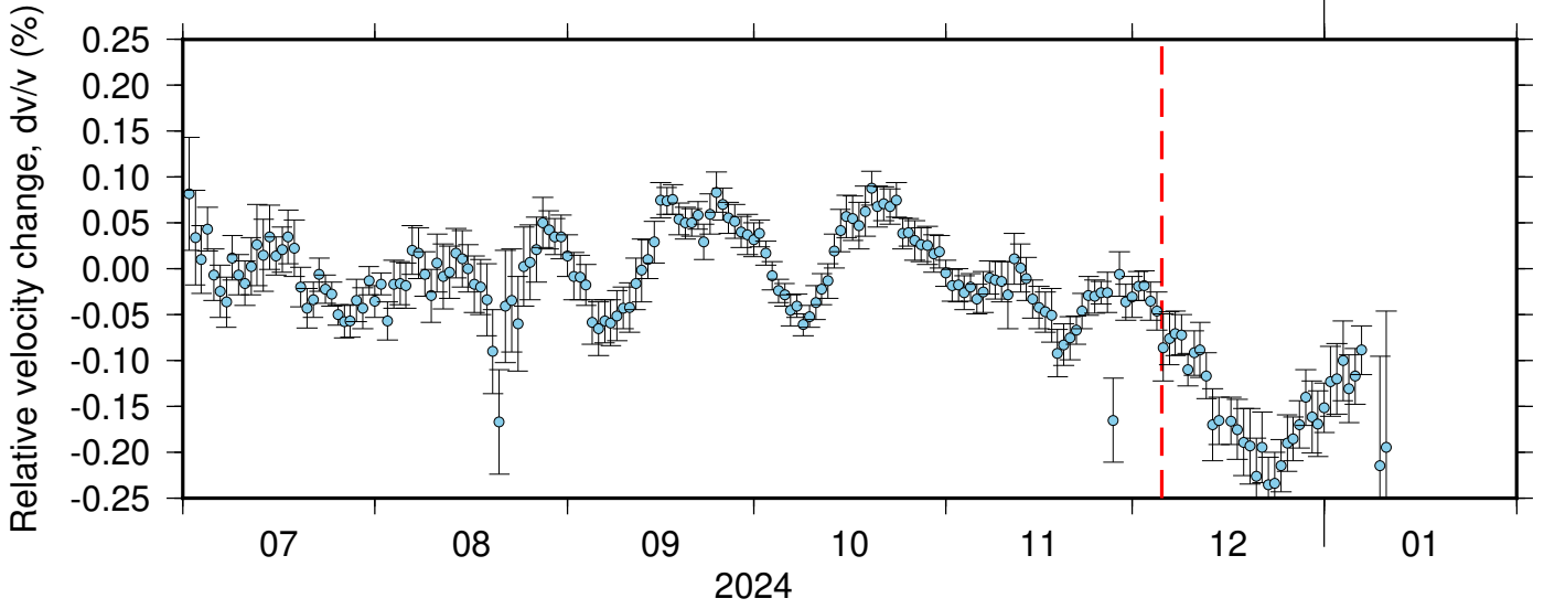
BK_GHOP_NC_KMPB ZRT 0.10-0.90Hz 011
