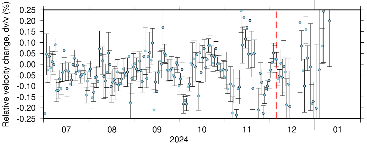
BK_RBOW_NC_KCT ZRT 0.10-0.90Hz 011
