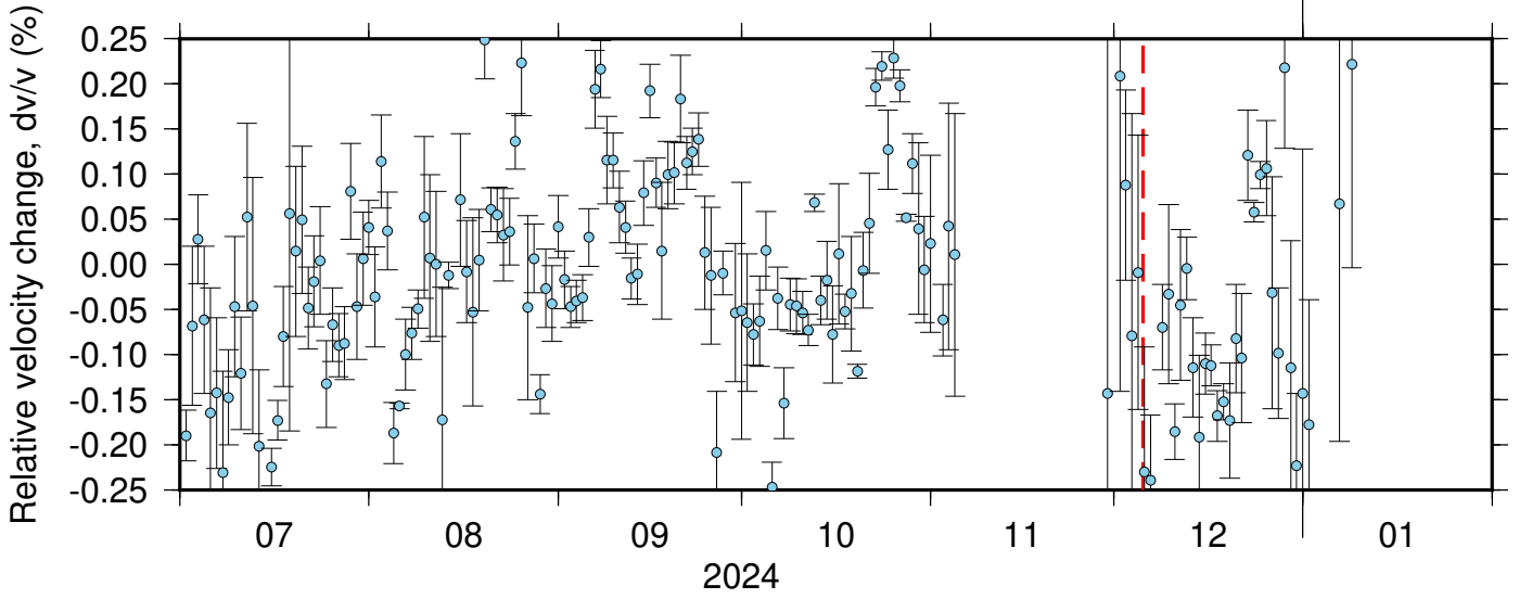
BK_GHOP_NC_KSM ZRT 0.10-0.90Hz 011
