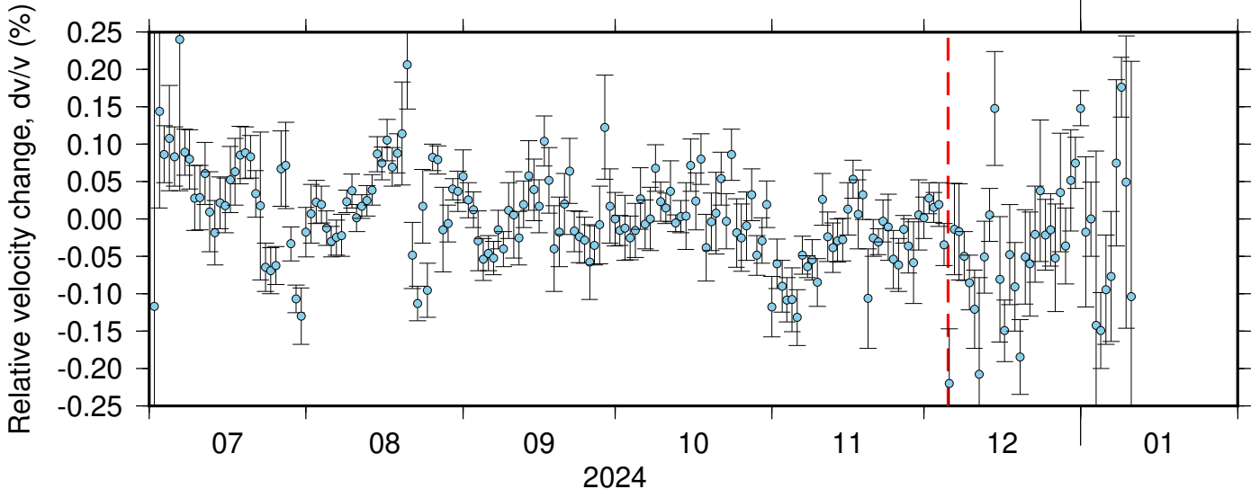
BK_PRDS_NC_KMR ZRT 0.10-0.90Hz 011
