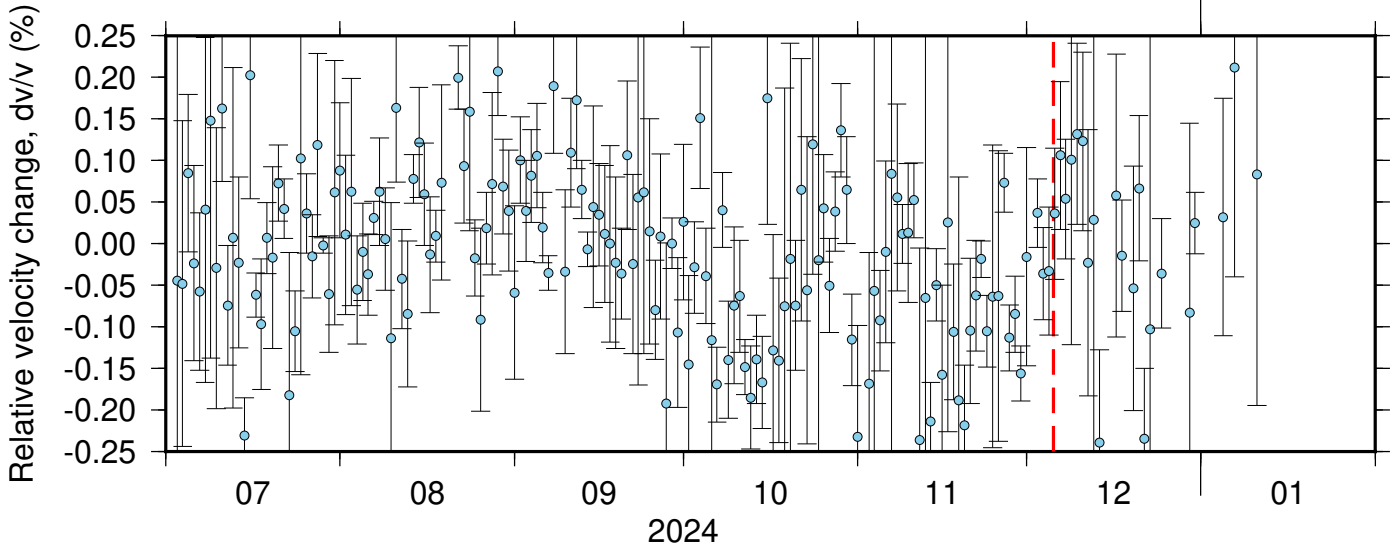
BK_PRDS_NC_KCT ZRT 0.10-0.90Hz 011
