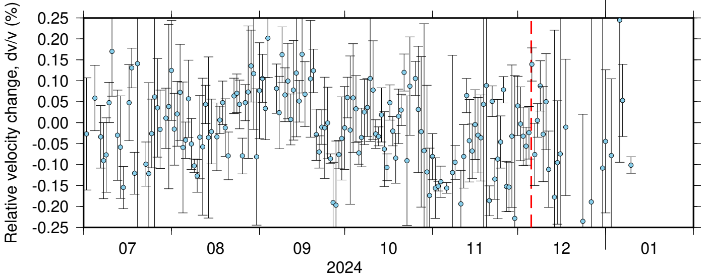
BK_JCC_NC_KMR ZRT 0.10-0.90Hz 011
