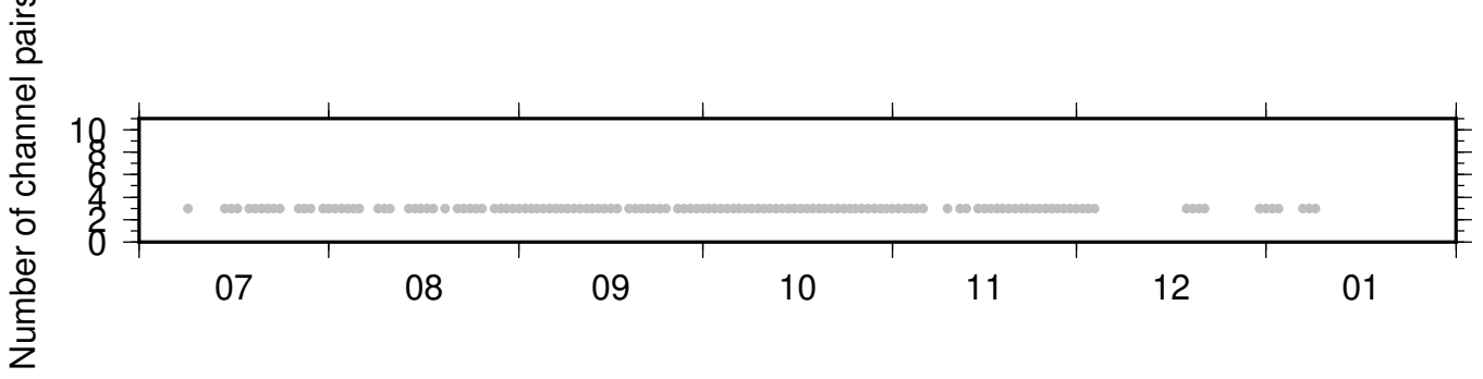
BK_JCC_NC_KCR ZRT 0.10-0.90Hz 011
