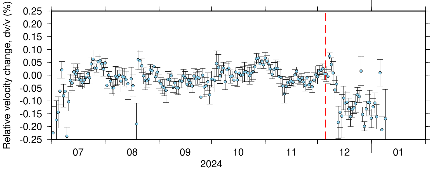
BK_GHOP_BK_PRDS ZRT 0.10-0.90Hz 011
