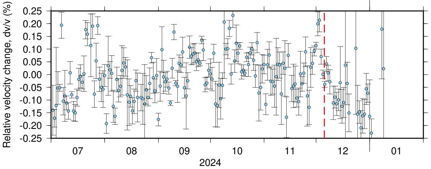
BK_SPRL_NC_KPR ZRT 0.10-0.90Hz 011
