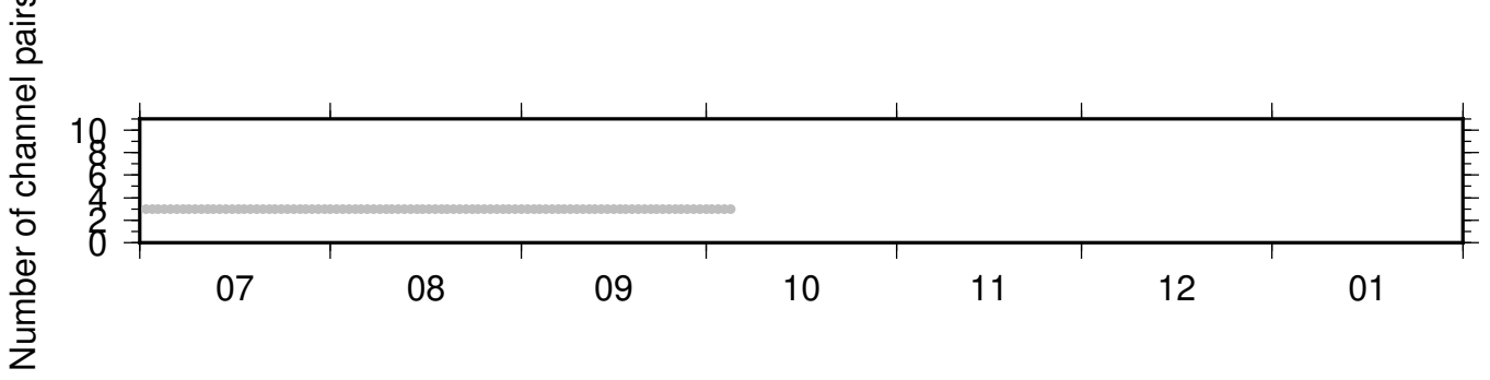
NC_KPR_PB_B932 ZRT 0.10-0.90Hz 011
