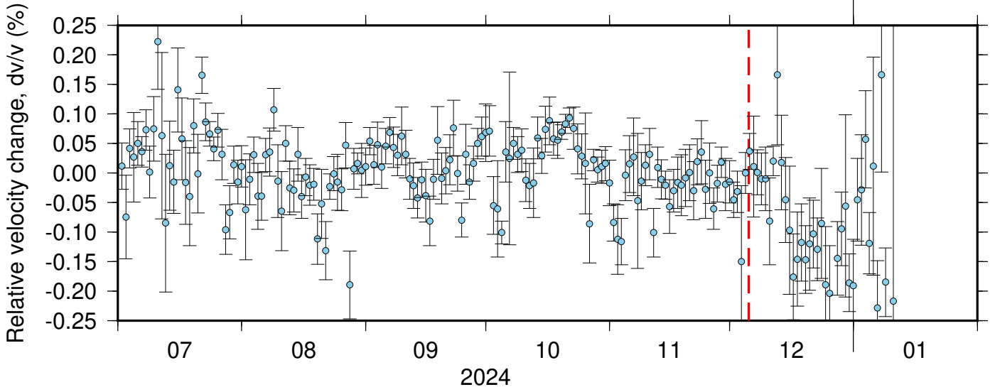
BK_PRDS_NC_KMPB ZRT 0.10-0.90Hz 011
