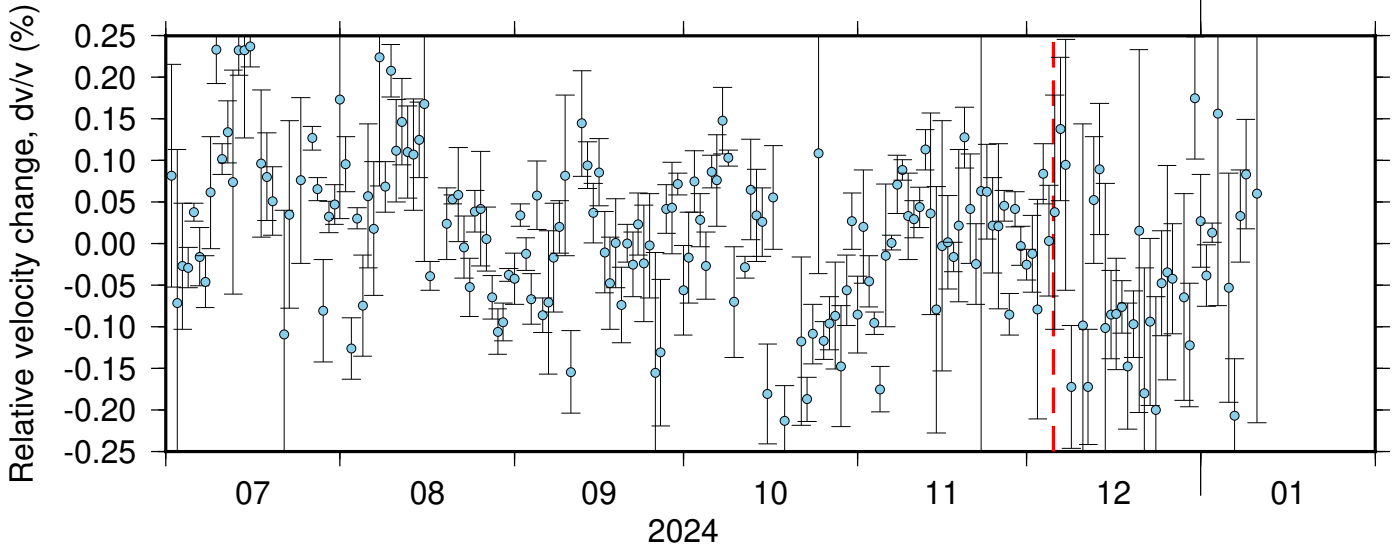
BK_BLAS_NC_KBU ZRT 0.10-0.90Hz 011
