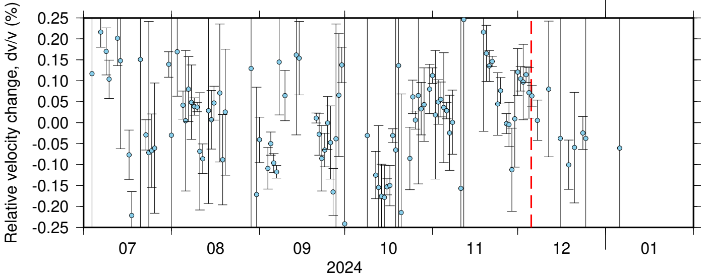
BK_HAYF_NC_KBU ZRT 0.10-0.90Hz 011
