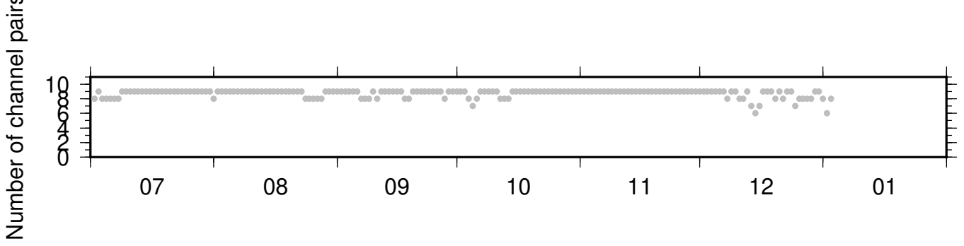
BK_GHOP_PB_B934 ZRT 0.10-0.90Hz 011
