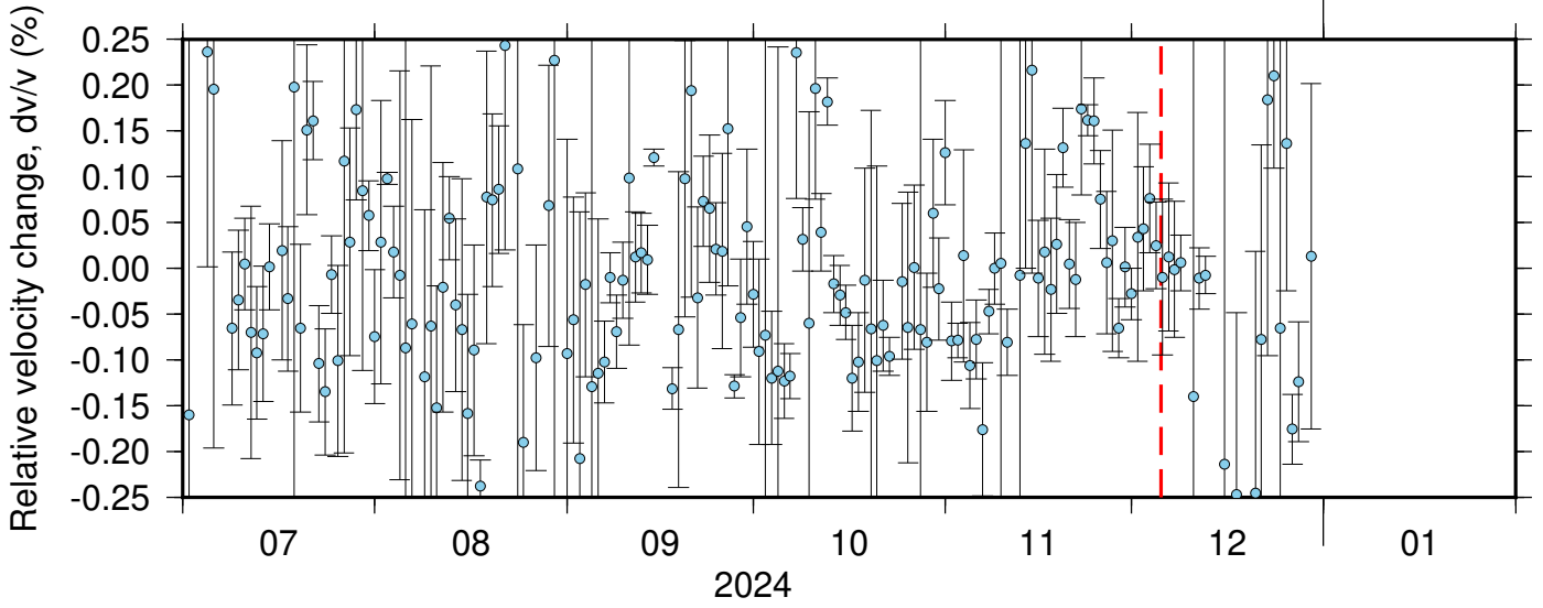
BK_RBOW_PB_B934 ZRT 0.10-0.90Hz 011
