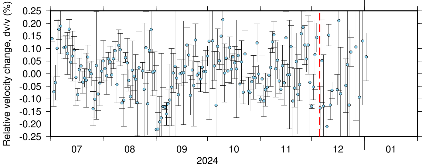
BK_GHOP_PB_B934 ZRT 0.10-0.90Hz 011
