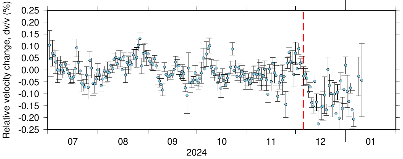
BK_GHOP_BK_SPRL ZRT 0.10-0.90Hz 011
