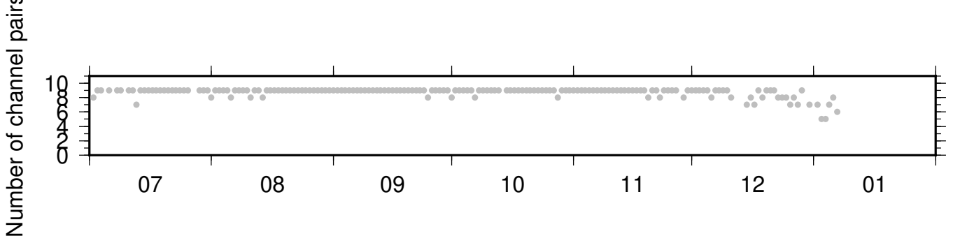
BK_HAYF_BK_PETL ZRT 0.10-0.90Hz 011
