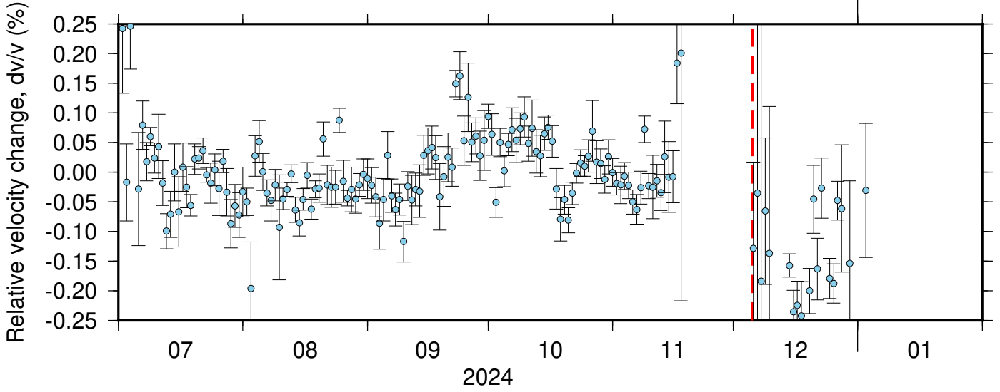
BK_PRDS_PB_B049 ZRT 0.10-0.90Hz 011
