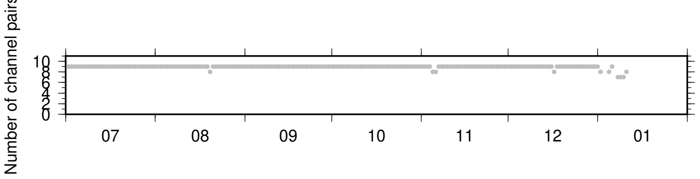
BK_PETL_BK_SPRL ZRT 0.10-0.90Hz 011
