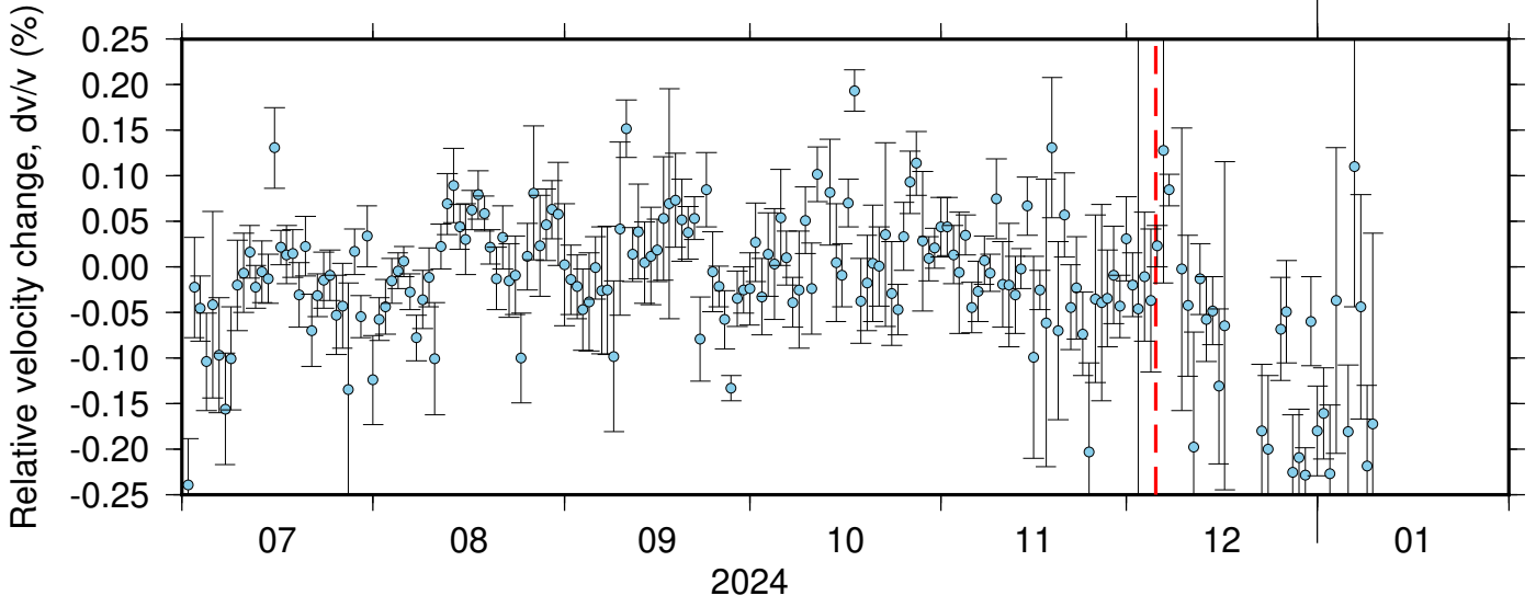
BK_RBOW_BK_SPRL ZRT 0.10-0.90Hz 011
