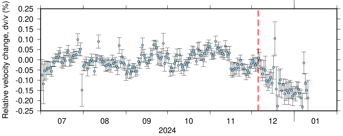
BK_GHOP_NC_KMR ZRT 0.10-0.90Hz 011
