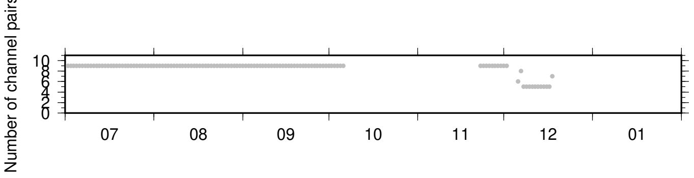
BK_RBOW_PB_B932 ZRT 0.10-0.90Hz 011
