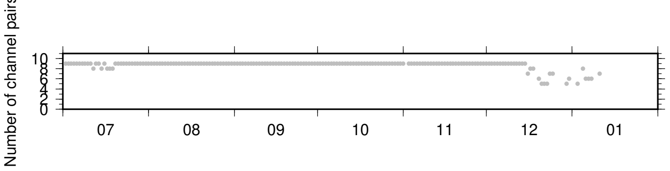
BK_PRDS_NC_KCT ZRT 0.10-0.90Hz 011
