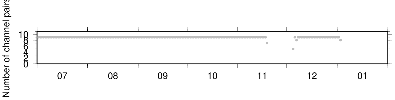
NC_KMPB_PB_B049 ZRT 0.10-0.90Hz 011
