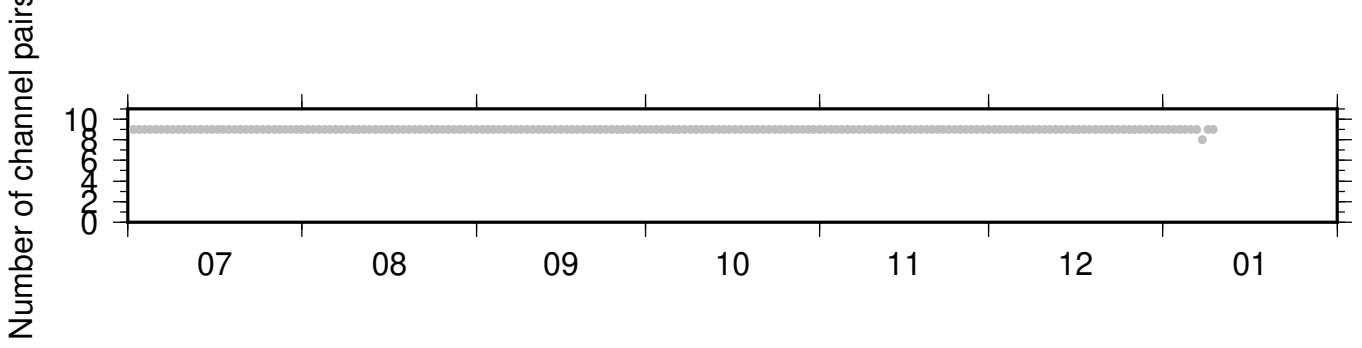
BK_HAYF_NC_KMR ZRT 0.10-0.90Hz 011
