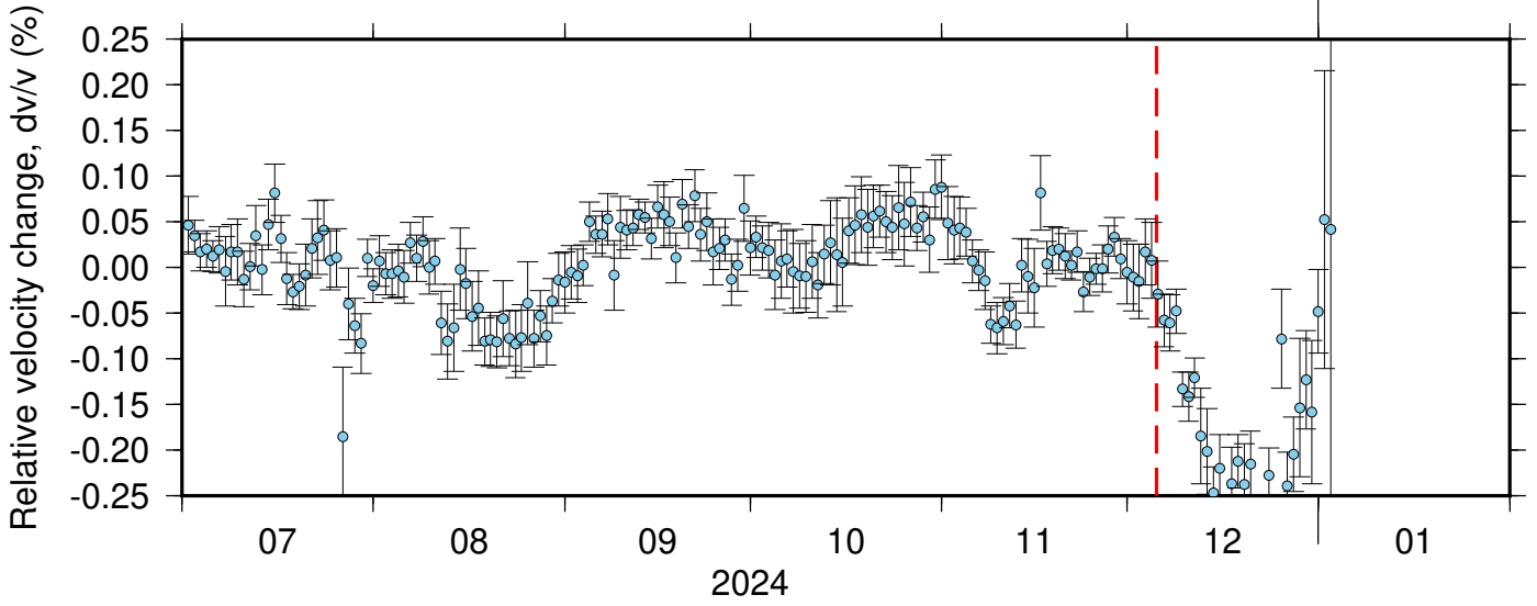
NC_KMPB_PB_B047 ZRT 0.10-0.90Hz 011
