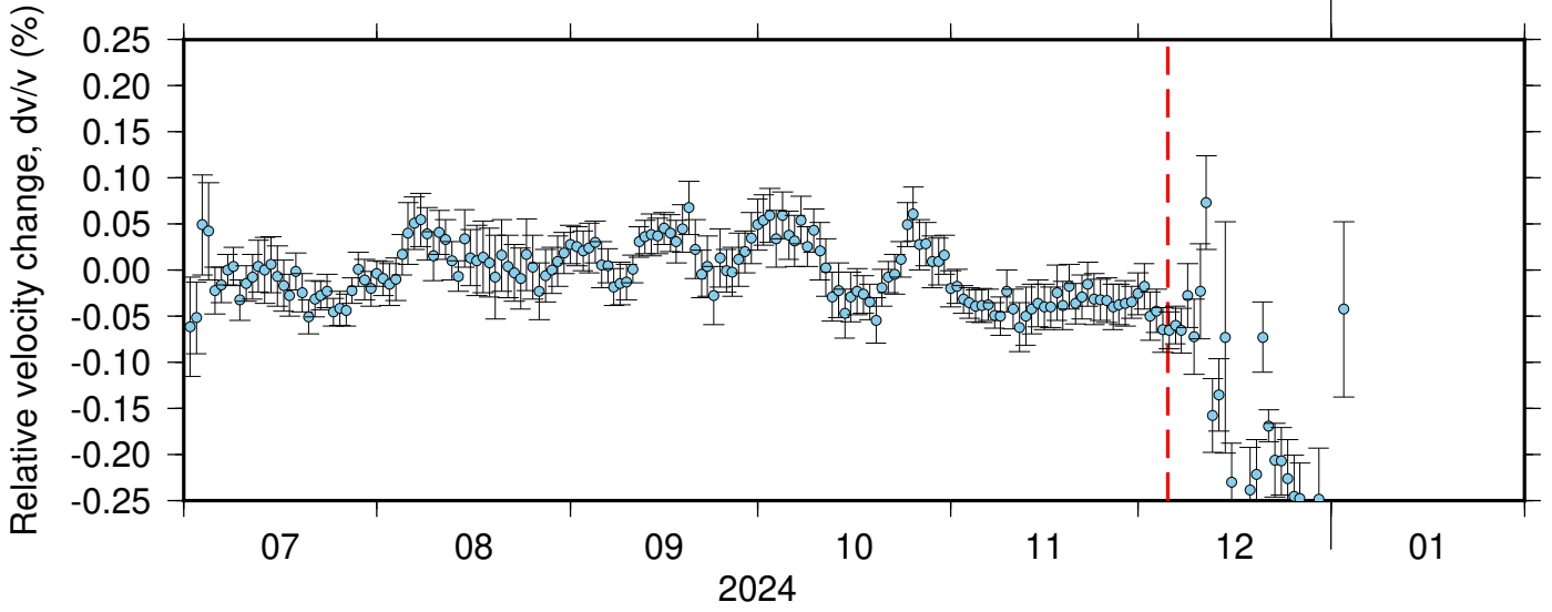
BK_RBOW_PB_B047 ZRT 0.10-0.90Hz 011
