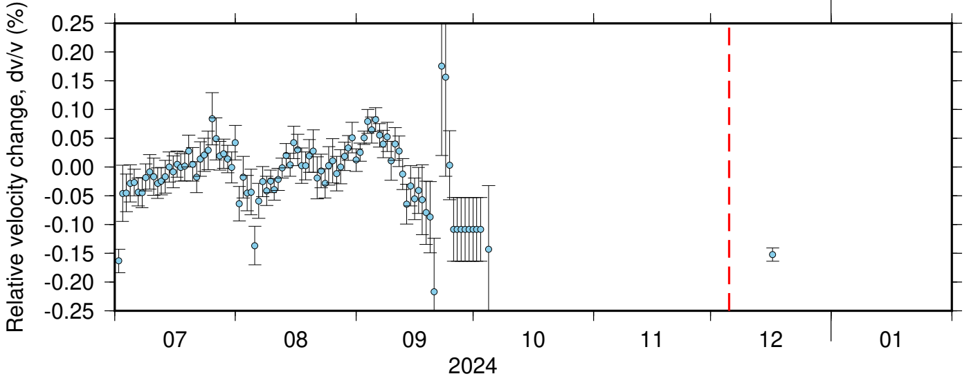
BK_RBOW_PB_B932 ZRT 0.10-0.90Hz 011
