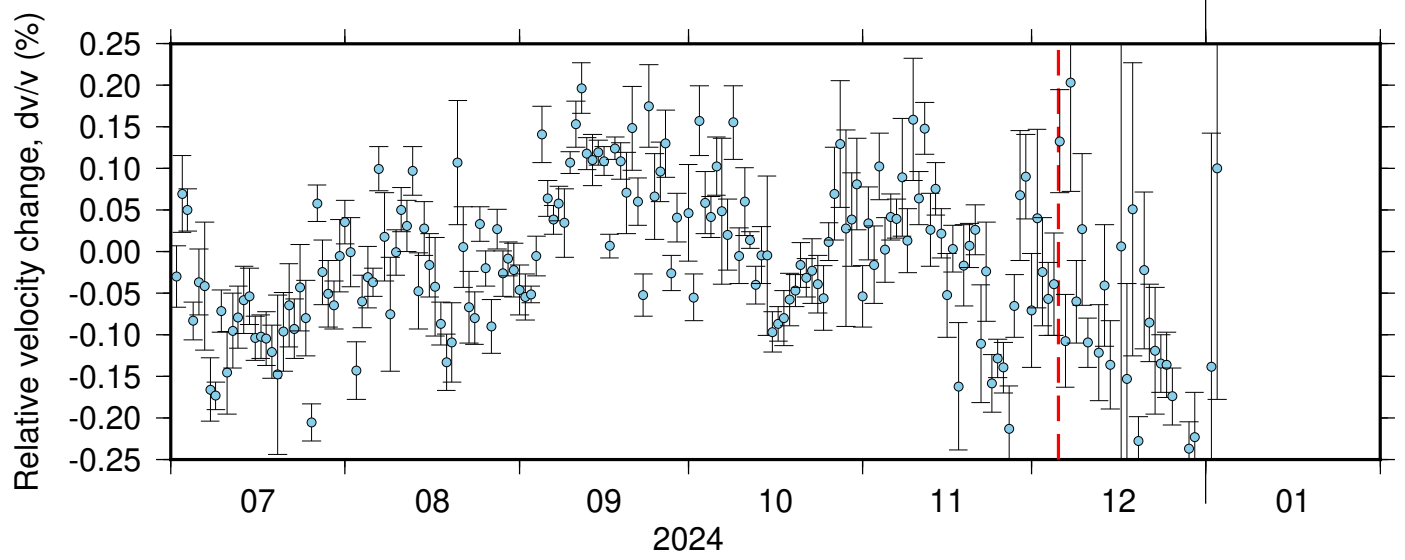
NC_KPR_PB_B047 ZRT 0.10-0.90Hz 011
