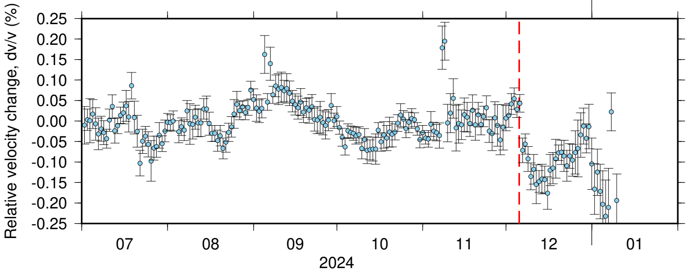
BK_BLAS_NC_KMR ZRT 0.10-0.90Hz 011
