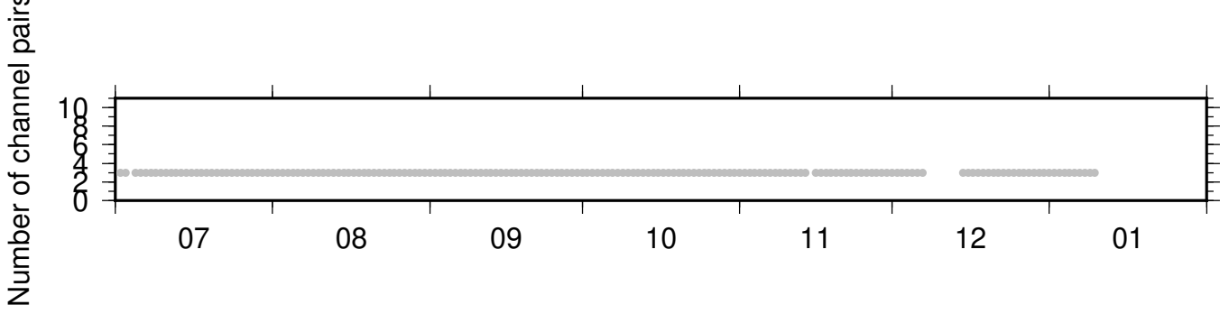
BK_RBOW_NC_KCR ZRT 0.10-0.90Hz 011
