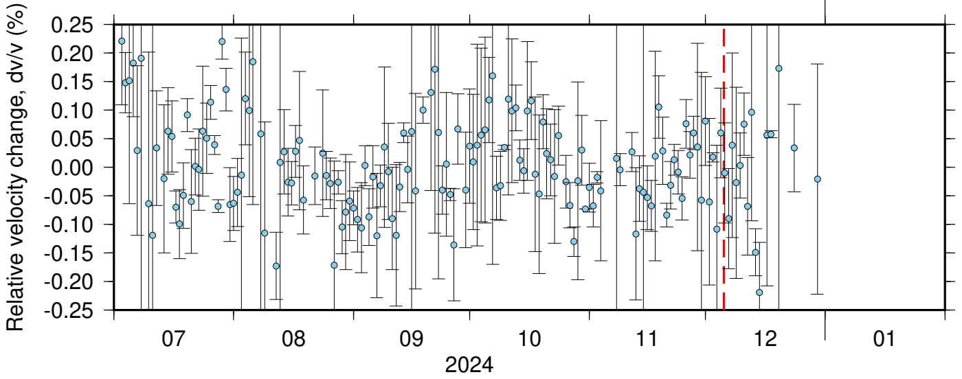
NC_KMPB_PB_B934 ZRT 0.10-0.90Hz 011
