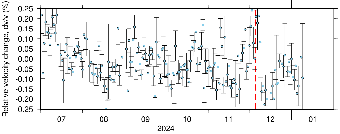
BK_RBOW_NC_KBU ZRT 0.10-0.90Hz 011
