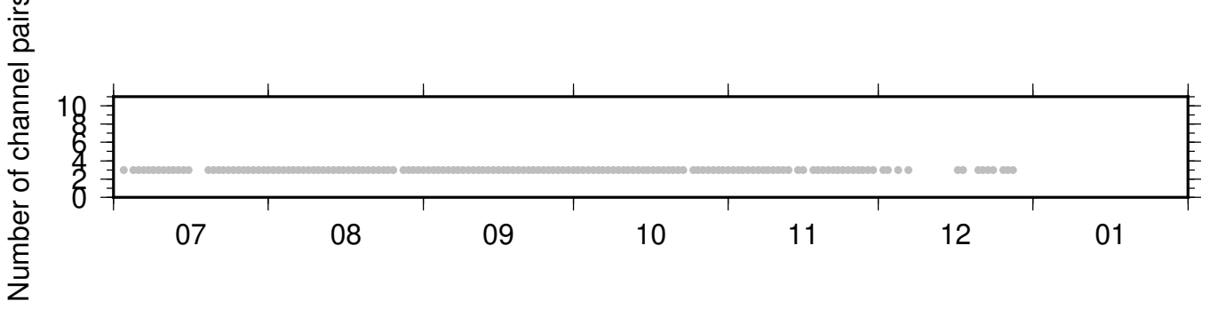
BK_PRDS_NC_KCR ZRT 0.10-0.90Hz 011
