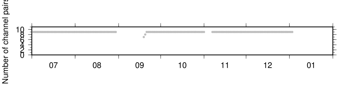
NC_KMPB_PB_B045 ZRT 0.10-0.90Hz 011
