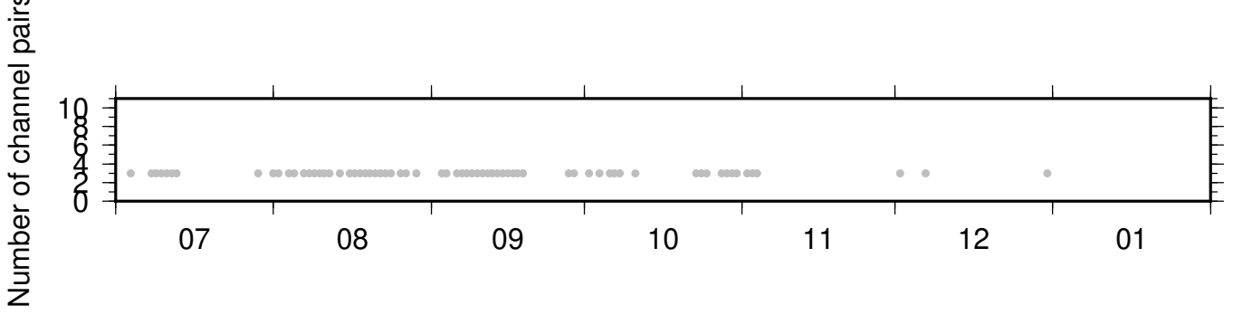
BK_JCC_NC_KSM ZRT 0.10-0.90Hz 011
