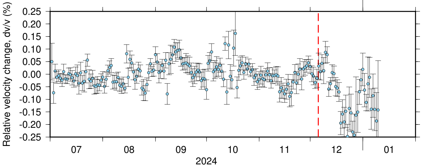
BK_BRIC_NC_KMR ZRT 0.10-0.90Hz 011
