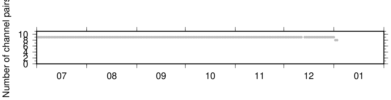
BK_GHOP_PB_B935 ZRT 0.10-0.90Hz 011
