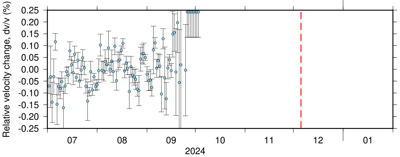
NC_KPR_PB_B932 ZRT 0.10-0.90Hz 011
