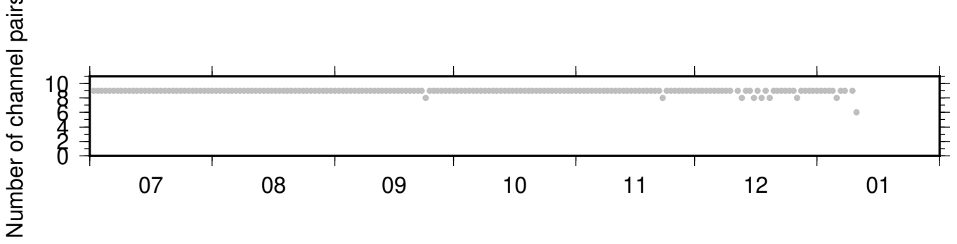
BK_GHOP_BK_HAYF ZRT 0.10-0.90Hz 011
