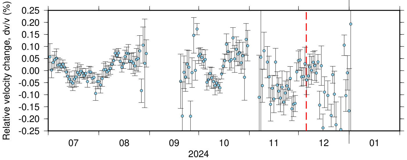
NC_KMPB_PB_B045 ZRT 0.10-0.90Hz 011
