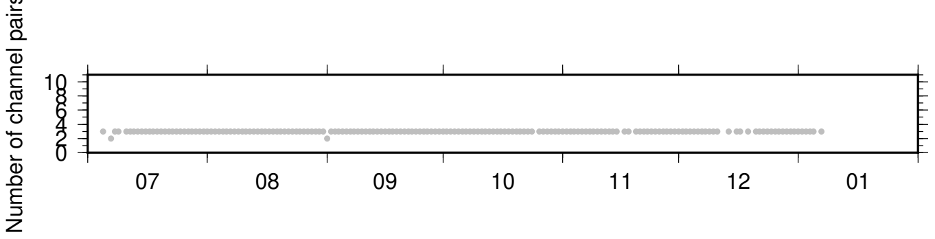
BK_SPRL_NC_KCR ZRT 0.10-0.90Hz 011
