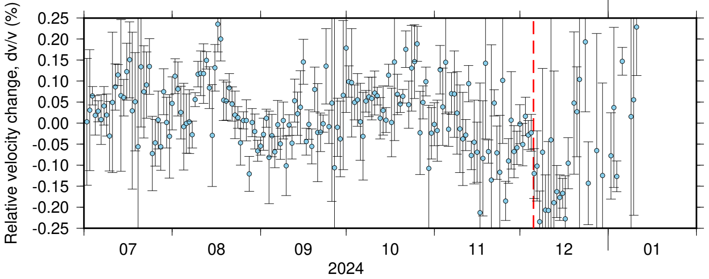
BK_BLAS_NC_KMPB ZRT 0.10-0.90Hz 011
