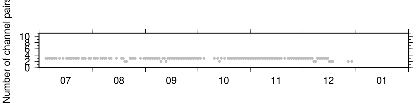
NC_KPR_PB_B934 ZRT 0.10-0.90Hz 011
