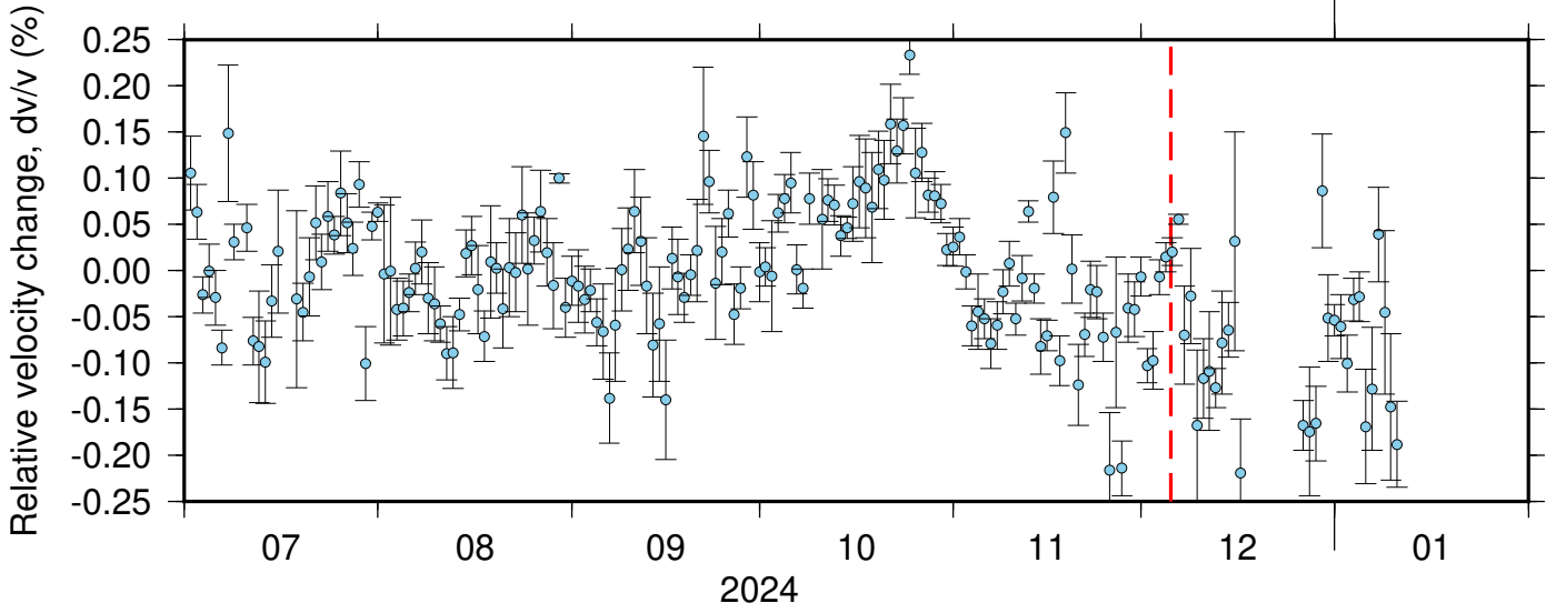
BK_GHOP_NC_KPR ZRT 0.10-0.90Hz 011
