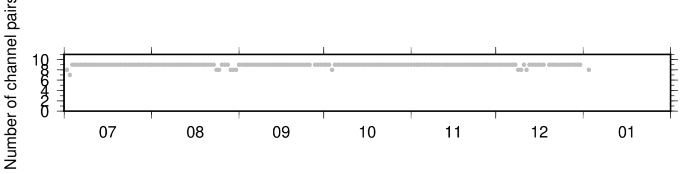
BK_RBOW_PB_B935 ZRT 0.10-0.90Hz 011
