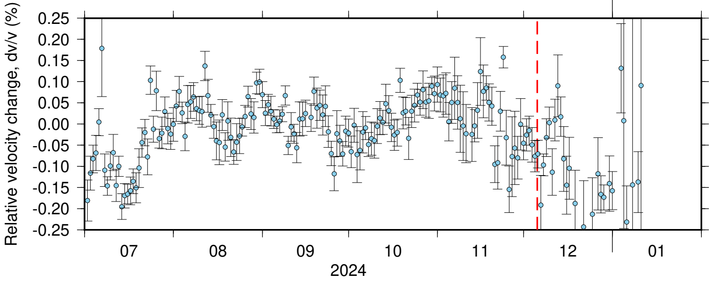
BK_RBOW_BK_WLKR ZRT 0.10-0.90Hz 011
