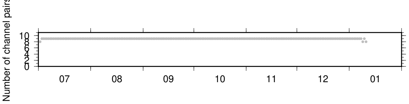
BK_BLAS_NC_KMPB ZRT 0.10-0.90Hz 011
