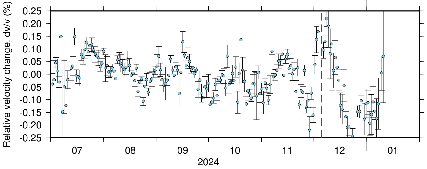
BK_GHOP_NC_KBU ZRT 0.10-0.90Hz 011
