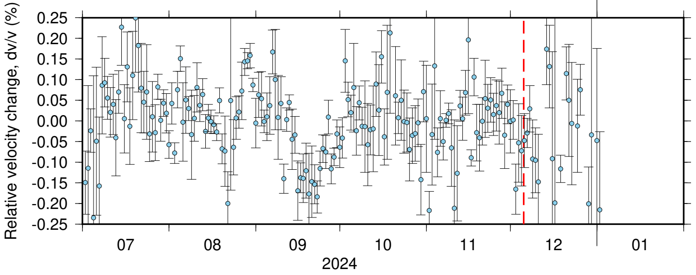
BK_GHOP_PB_B935 ZRT 0.10-0.90Hz 011
