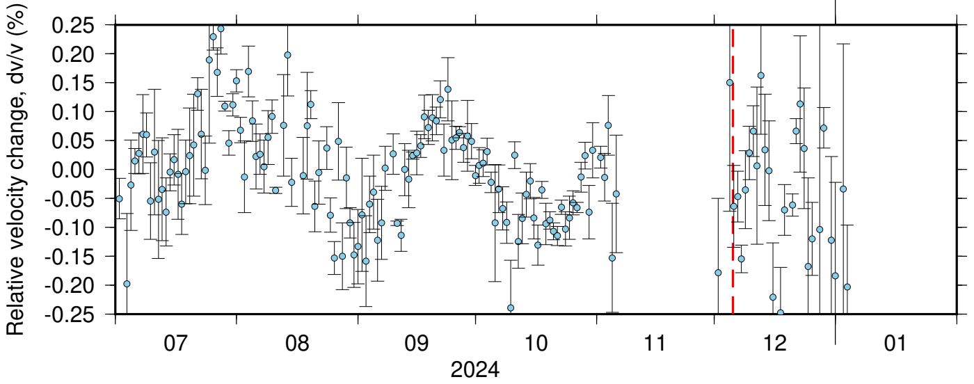
BK_RBOW_NC_KSM ZRT 0.10-0.90Hz 011
