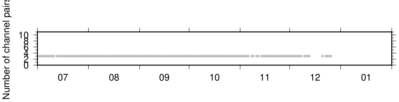
BK_PETL_NC_KBU ZRT 0.10-0.90Hz 011
