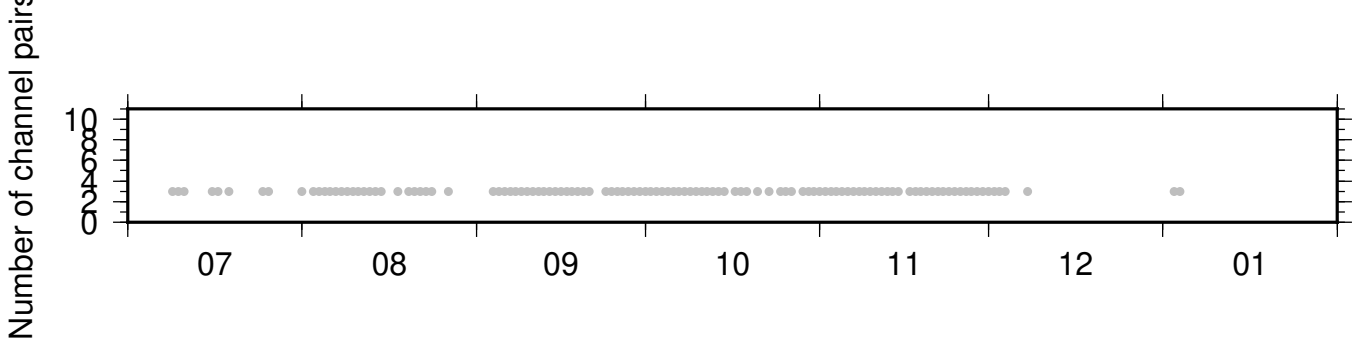
BK_PETL_NC_KCR ZRT 0.10-0.90Hz 011
