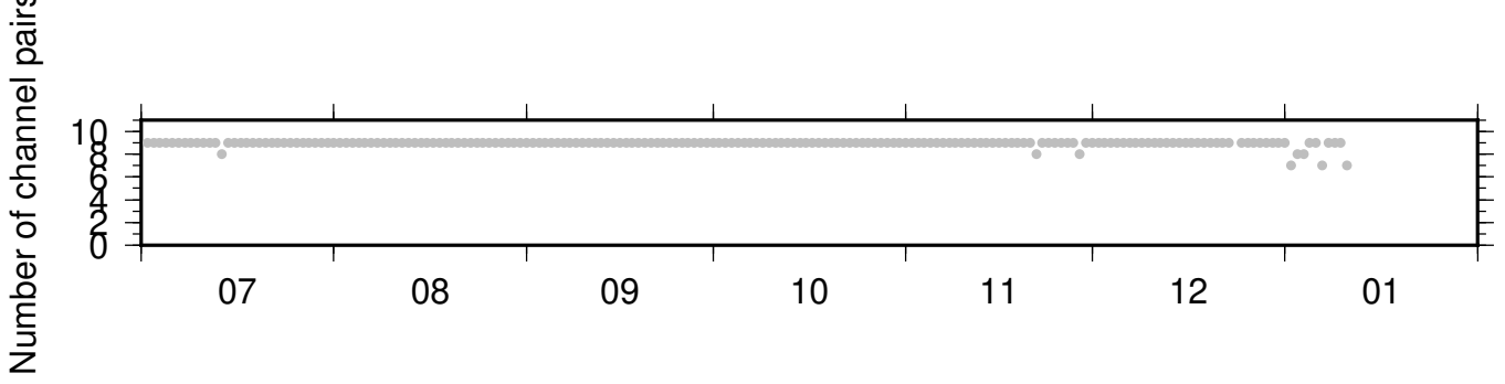
BK_PETL_NC_KMR ZRT 0.10-0.90Hz 011
