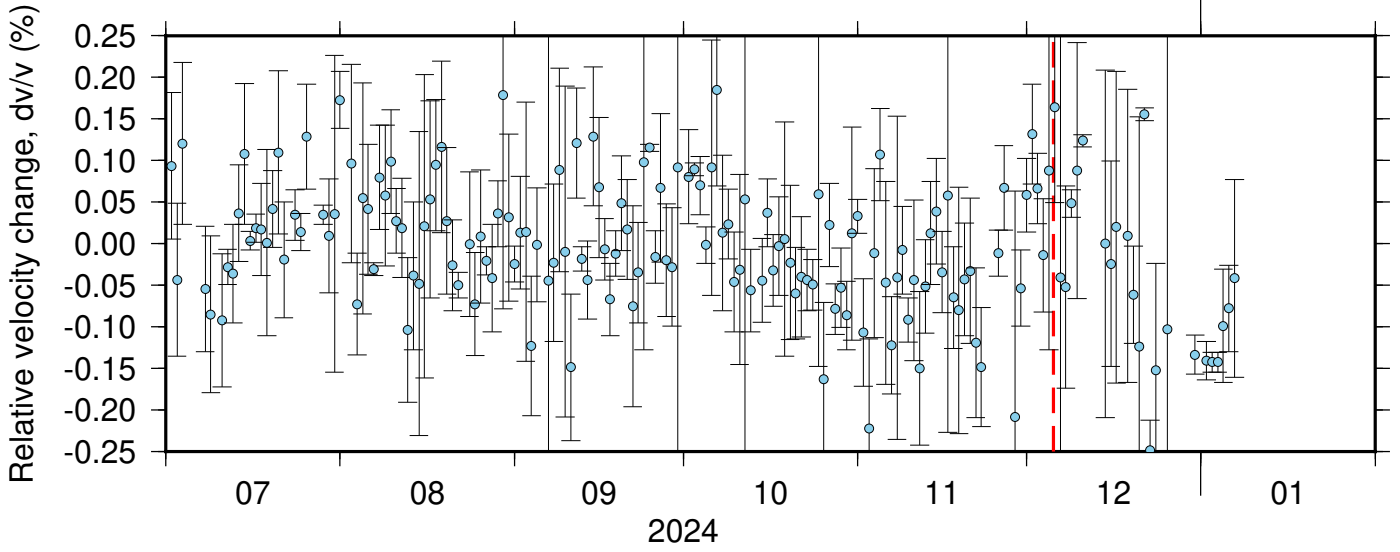
BK_HAYF_BK_PETL ZRT 0.10-0.90Hz 011
