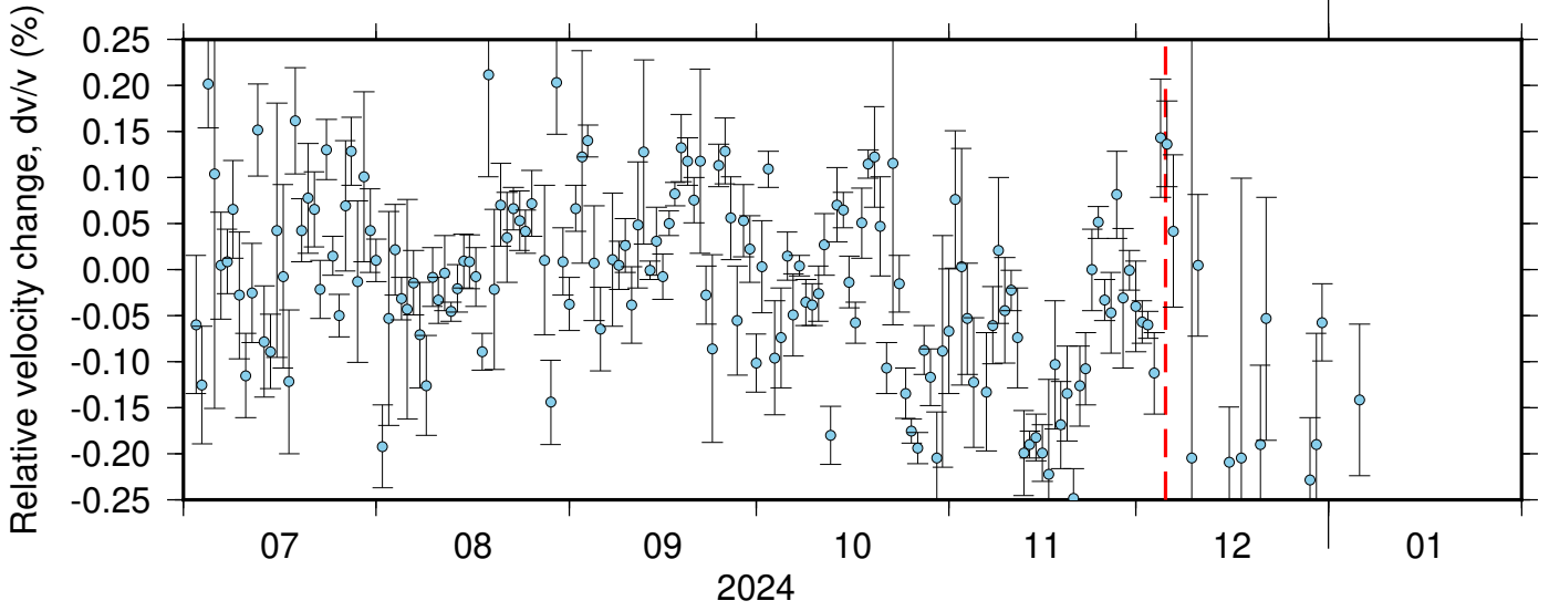
BK_GHOP_NC_KCR ZRT 0.10-0.90Hz 011
