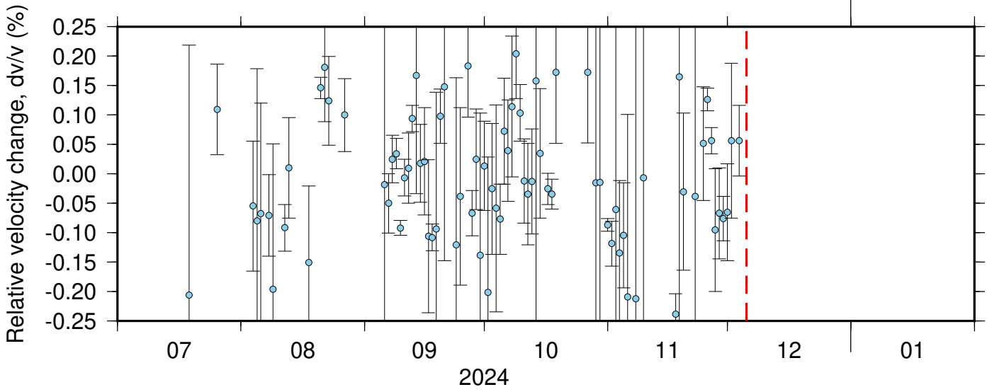
BK_PETL_NC_KCR ZRT 0.10-0.90Hz 011
