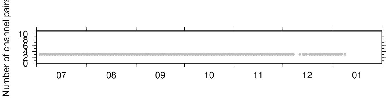
NC_KCR_NC_KMPB ZRT 0.10-0.90Hz 011
