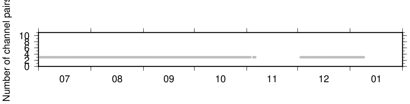
BK_SPRL_NC_KSM ZRT 0.10-0.90Hz 011
