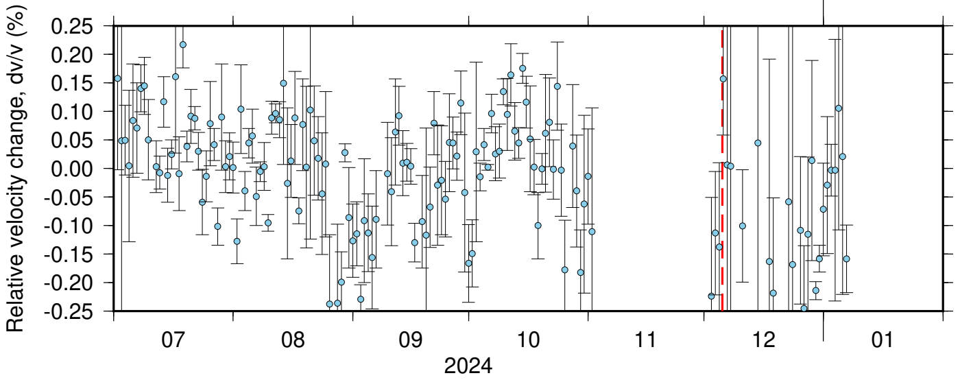
BK_SPRL_NC_KSM ZRT 0.10-0.90Hz 011
