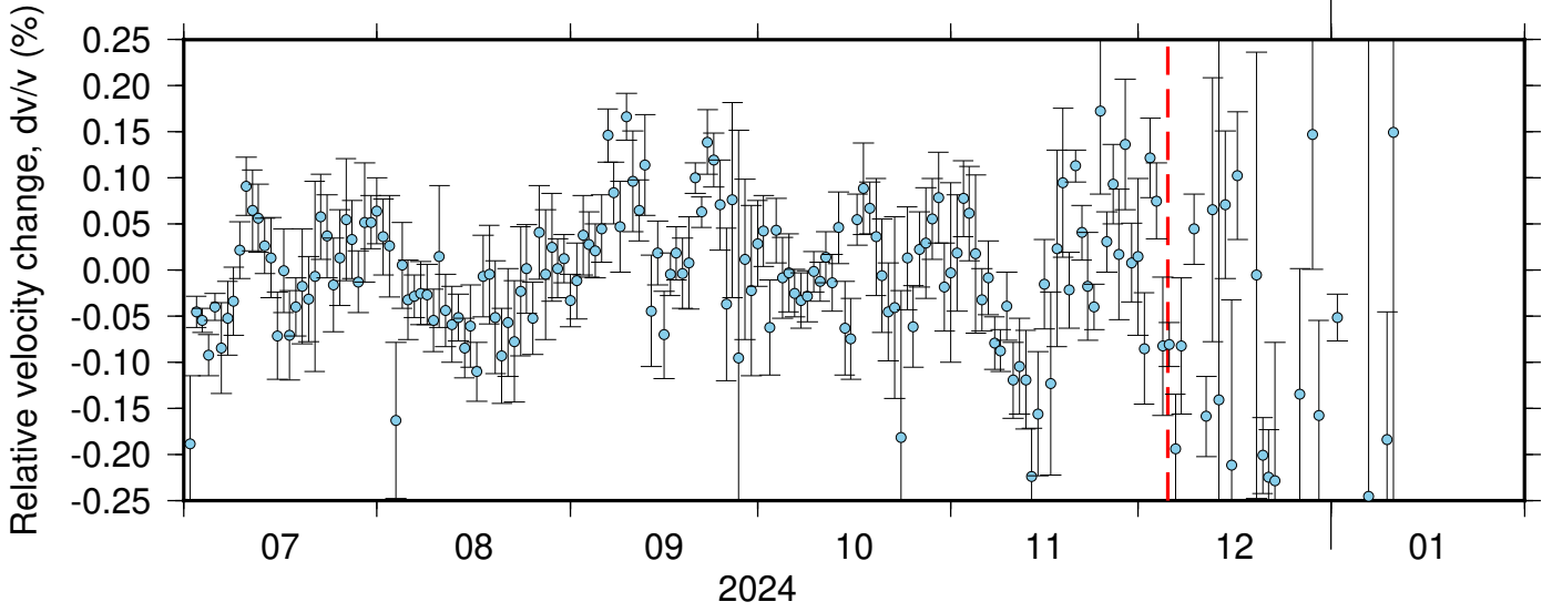
BK_GHOP_NC_KCT ZRT 0.10-0.90Hz 011
