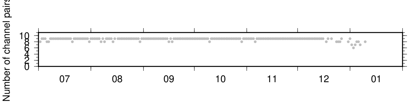
BK_JCC_NC_KMR ZRT 0.10-0.90Hz 011
