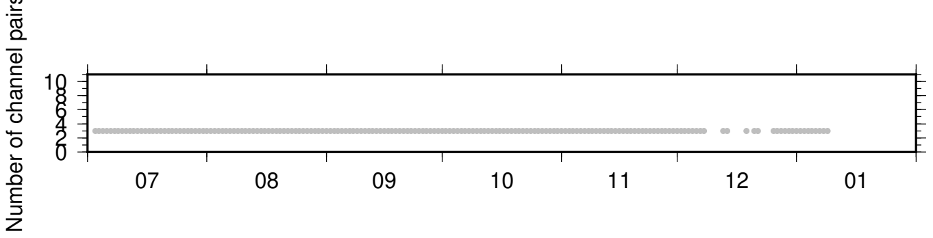
BK_BLAS_NC_KCR ZRT 0.10-0.90Hz 011
