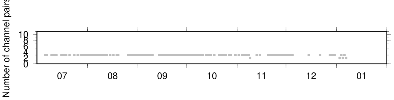
BK_HAYF_NC_KCR ZRT 0.10-0.90Hz 011
