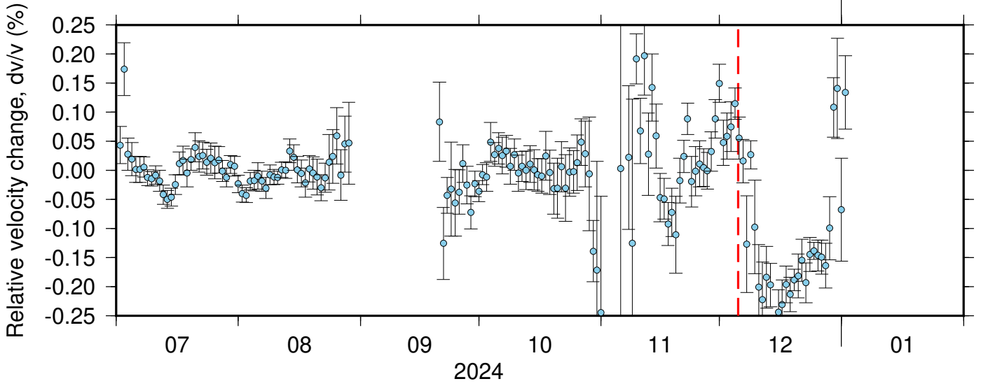
BK_GHOP_PB_B045 ZRT 0.10-0.90Hz 011
