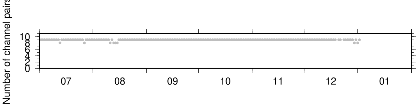
NC_KMPB_PB_B935 ZRT 0.10-0.90Hz 011
