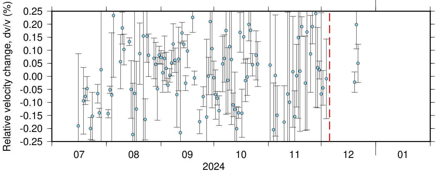
BK_JCC_NC_KCR ZRT 0.10-0.90Hz 011
