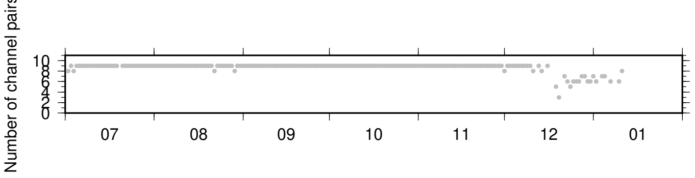
NC_KCT_NC_KMR ZRT 0.10-0.90Hz 011
