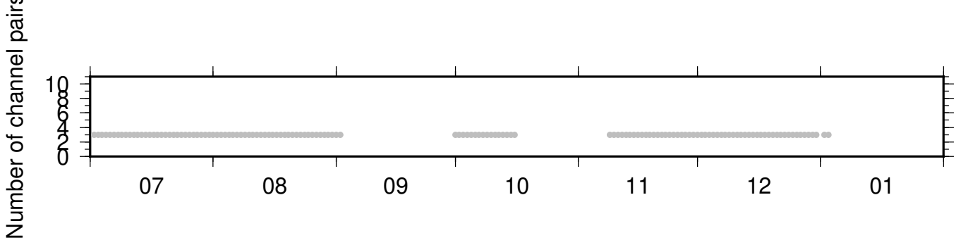
NC_KPR_PB_B046 ZRT 0.10-0.90Hz 011
