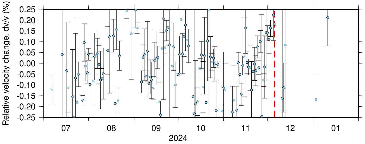
BK_BRIC_NC_KCR ZRT 0.10-0.90Hz 011
