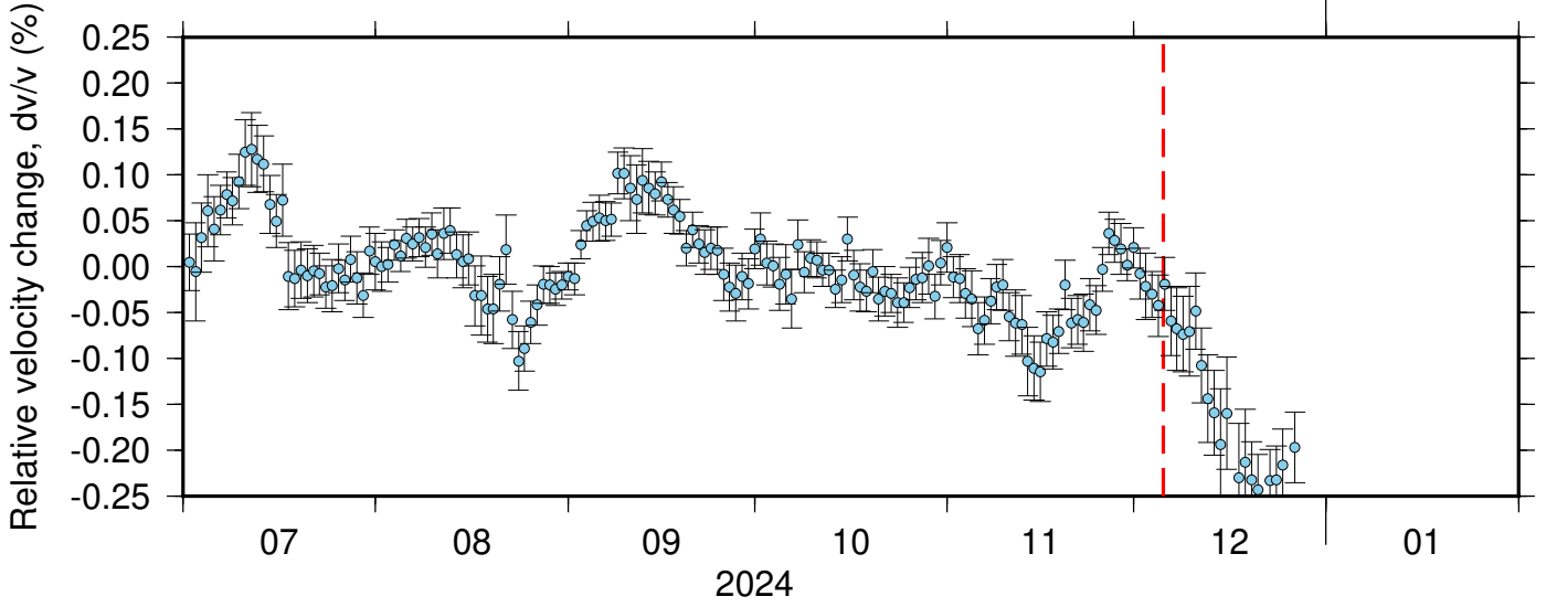
BK_RBOW_NC_KMPB ZRT 0.10-0.90Hz 011
