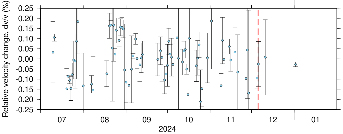
BK_JCC_NC_KBU ZRT 0.10-0.90Hz 011
