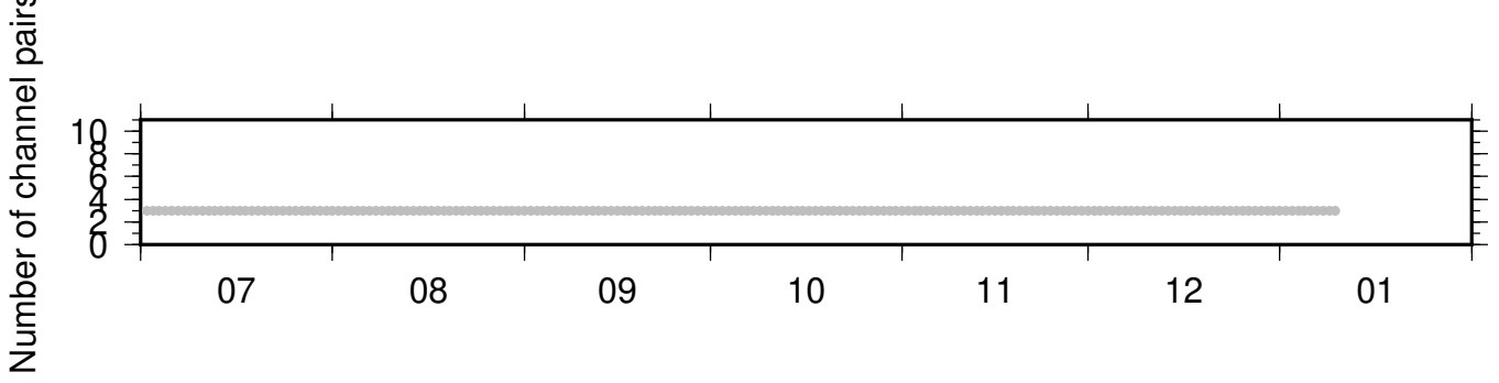
BK_SPRL_NC_KPR ZRT 0.10-0.90Hz 011
