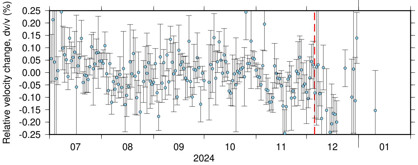
BK_PETL_BK_SPRL ZRT 0.10-0.90Hz 011
