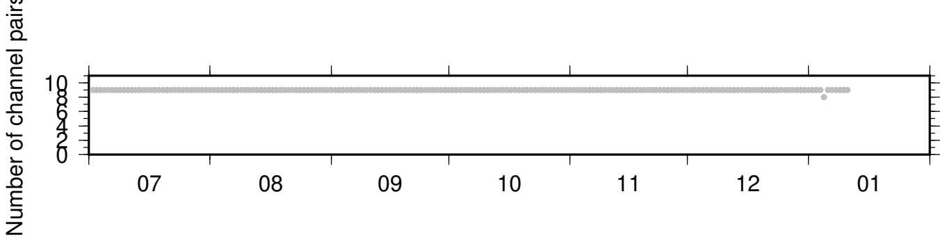
BK_PETL_NC_KMPB ZRT 0.10-0.90Hz 011
