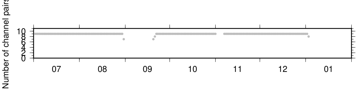
BK_RBOW_PB_B045 ZRT 0.10-0.90Hz 011
