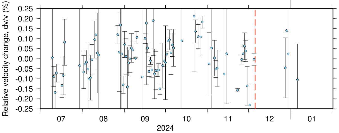
BK_HAYF_NC_KCR ZRT 0.10-0.90Hz 011
