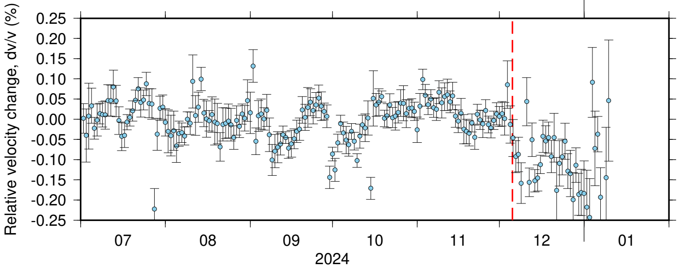
BK_SPRL_NC_KMR ZRT 0.10-0.90Hz 011
