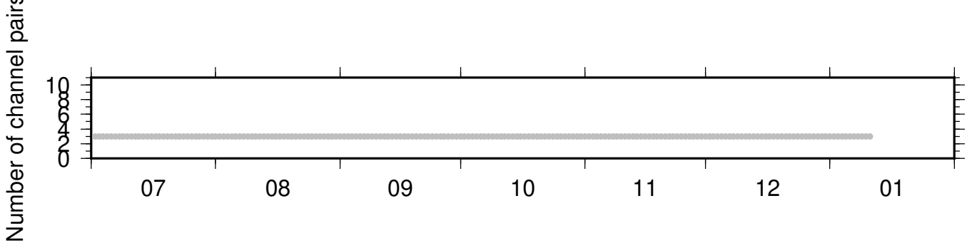
BK_BRIC_NC_KBU ZRT 0.10-0.90Hz 011
