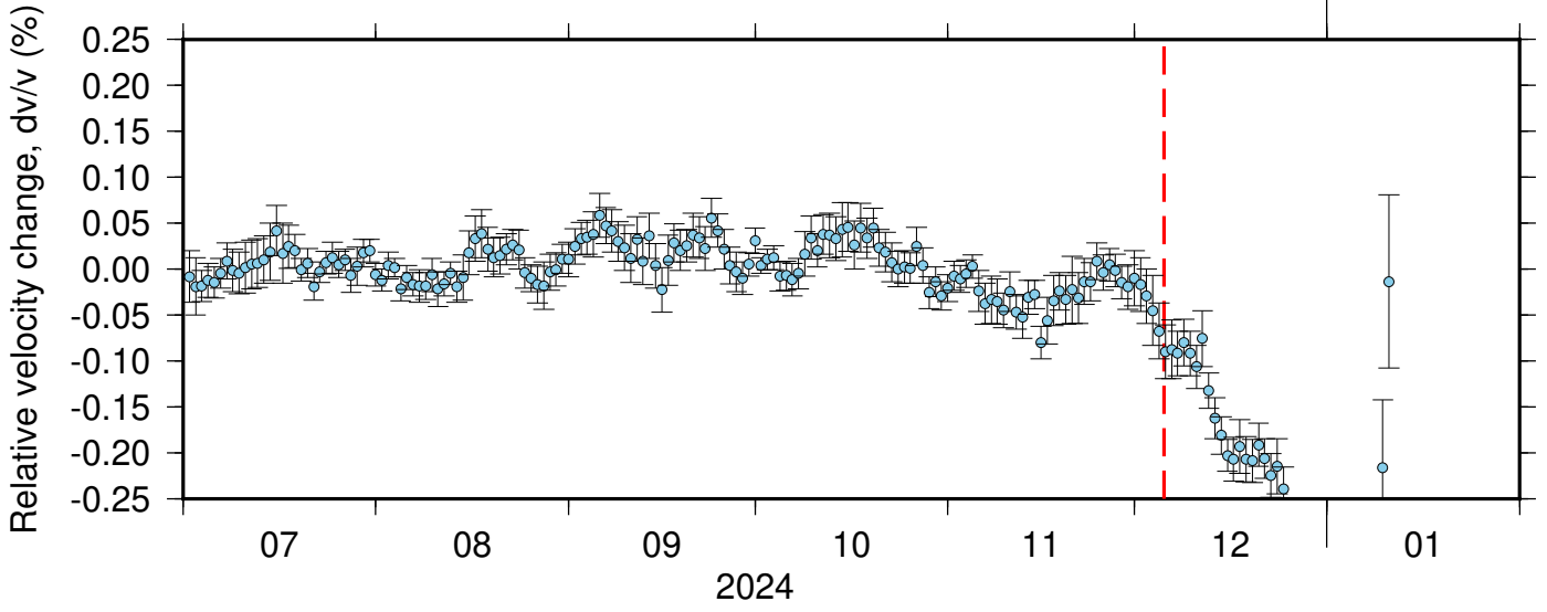
BK_PRDS_BK_SPRL ZRT 0.10-0.90Hz 011
