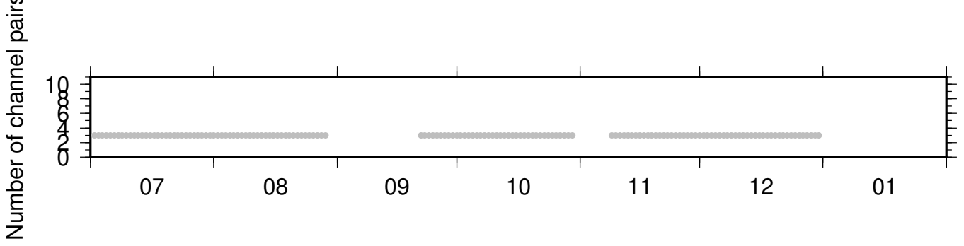
NC_KPR_PB_B045 ZRT 0.10-0.90Hz 011
