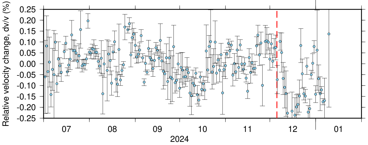
BK_BRIC_NC_KBU ZRT 0.10-0.90Hz 011
