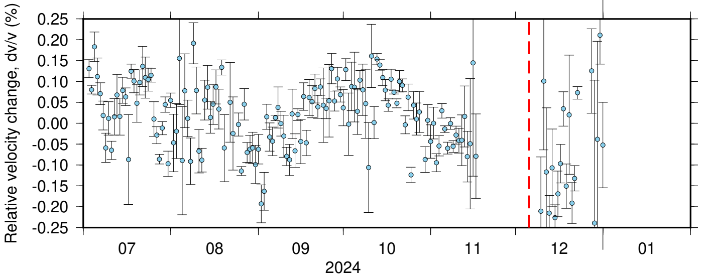
NC_KPR_PB_B049 ZRT 0.10-0.90Hz 011
