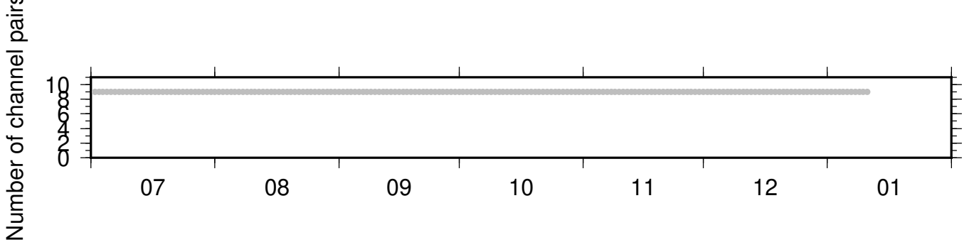
BK_GHOP_BK_PRDS ZRT 0.10-0.90Hz 011
