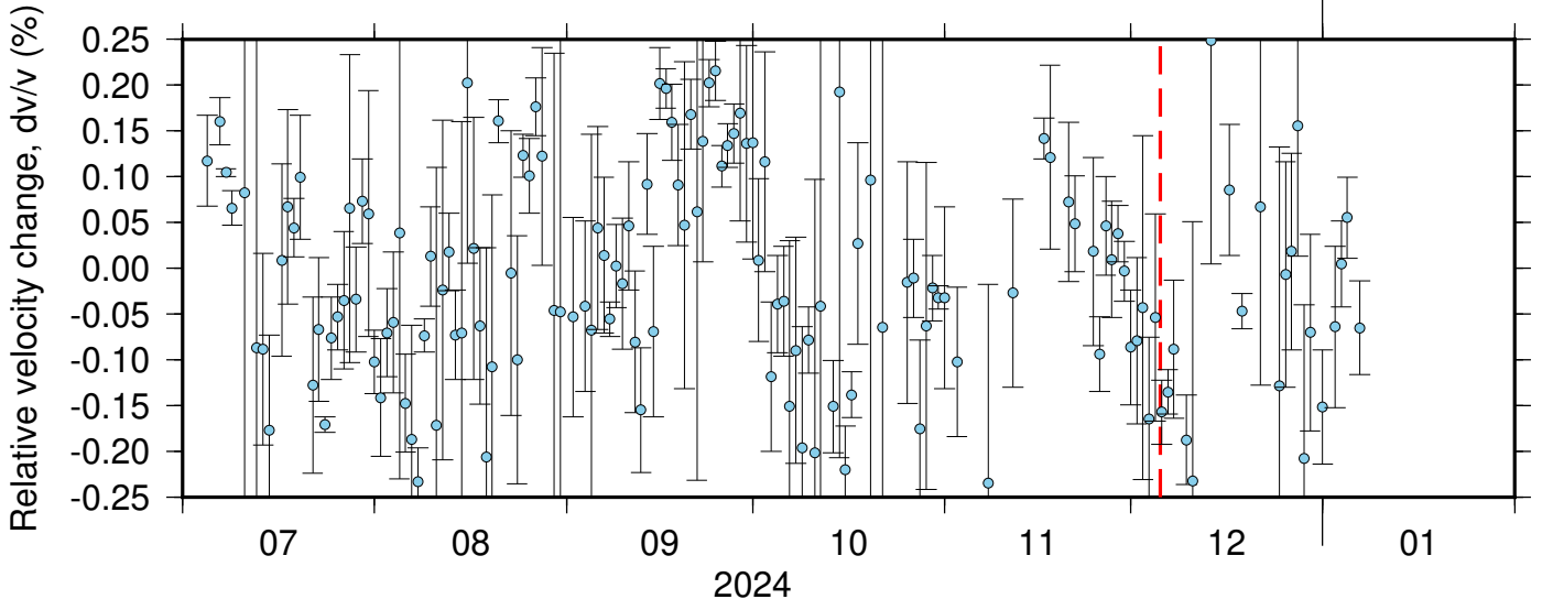
BK_SPRL_NC_KCR ZRT 0.10-0.90Hz 011
