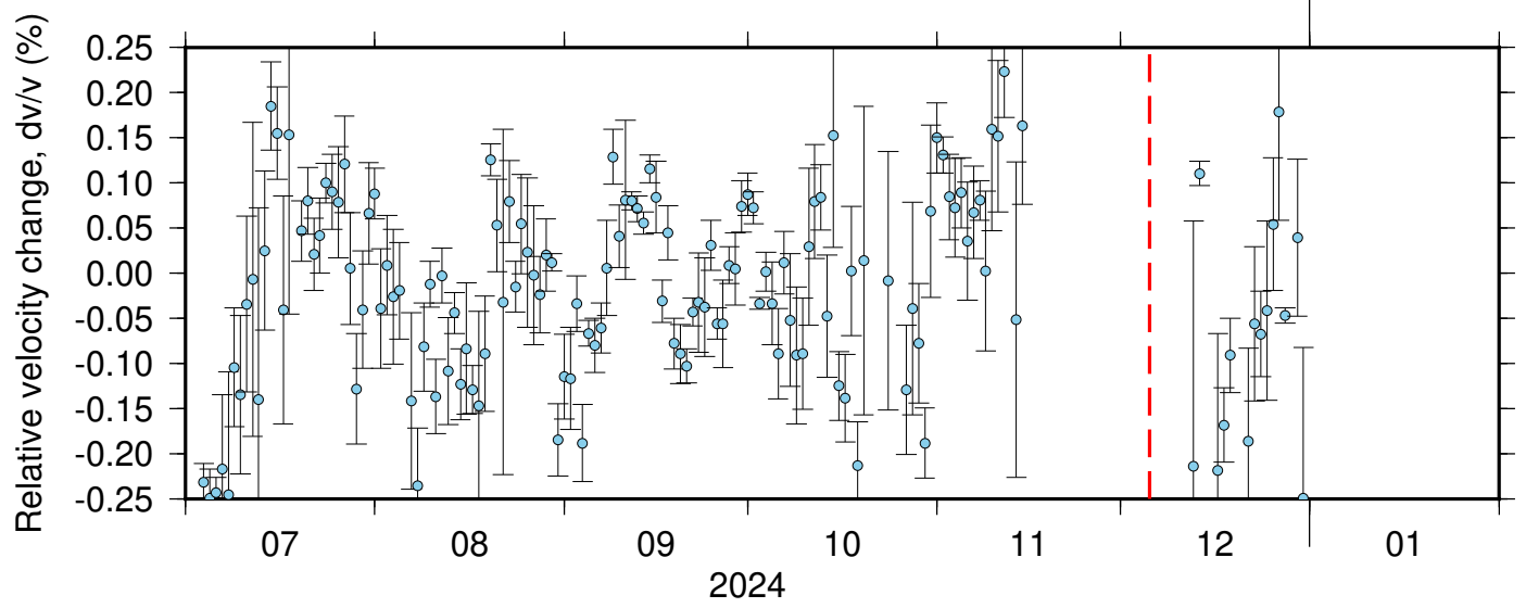
NC_KCR_PB_B049 ZRT 0.10-0.90Hz 011
