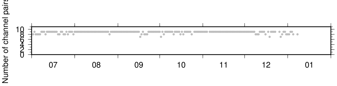
BK_HAYF_BK_WLKR ZRT 0.10-0.90Hz 011
