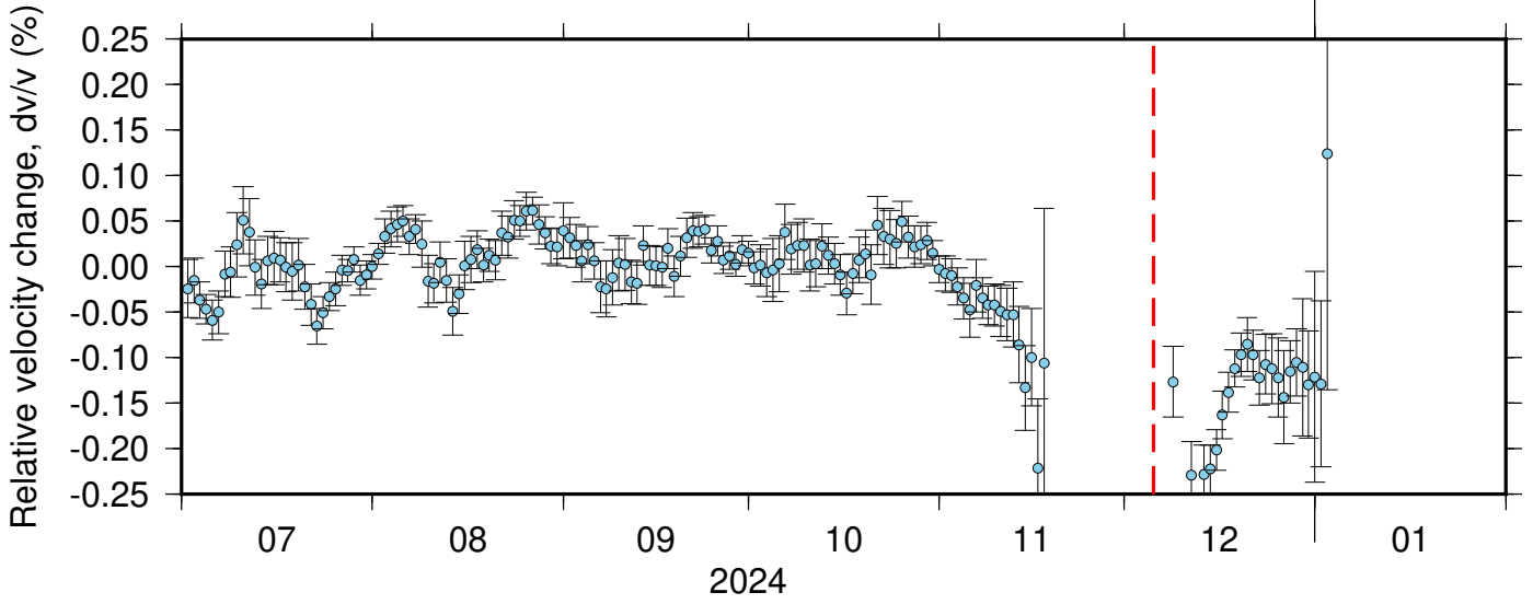
BK_GHOP_PB_B049 ZRT 0.10-0.90Hz 011
