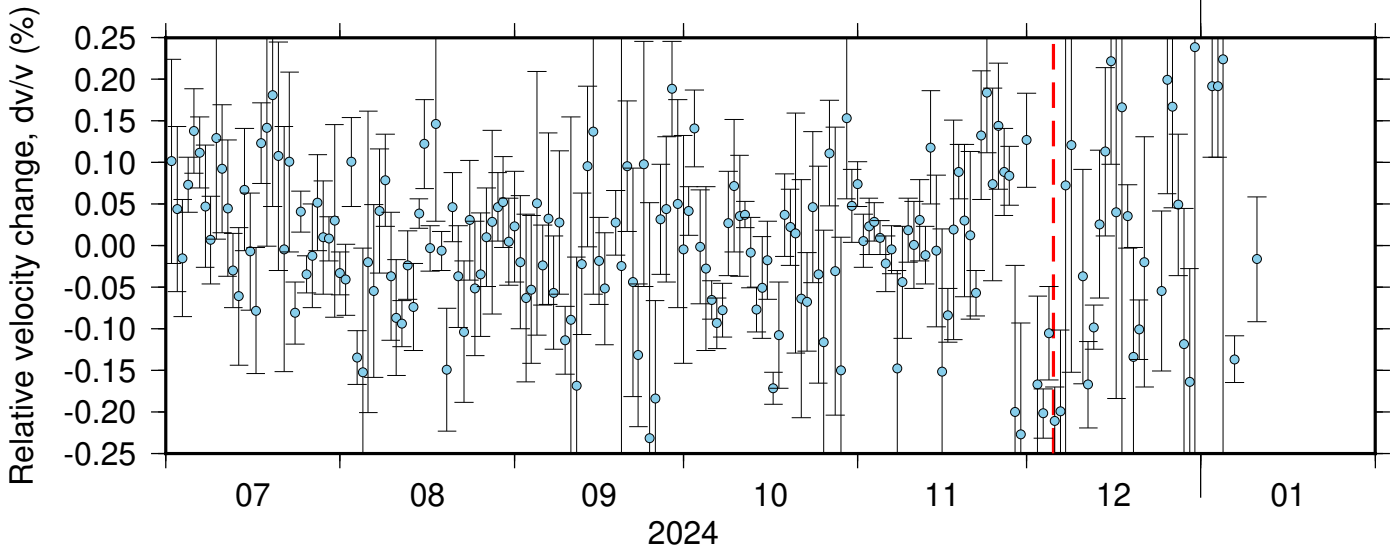
BK_PETL_NC_KMR ZRT 0.10-0.90Hz 011
