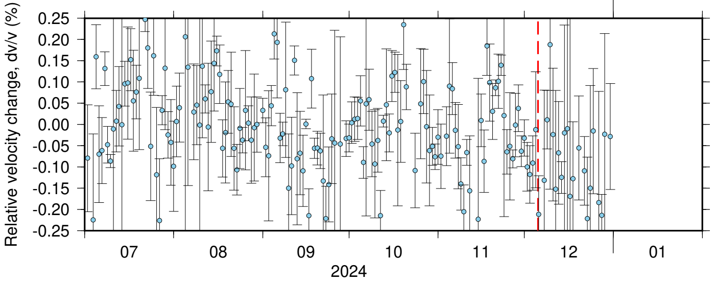
BK_RBOW_PB_B935 ZRT 0.10-0.90Hz 011
