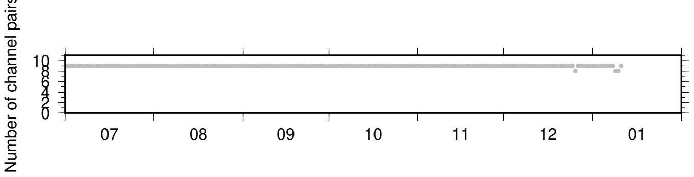
BK_BLAS_BK_SPRL ZRT 0.10-0.90Hz 011
