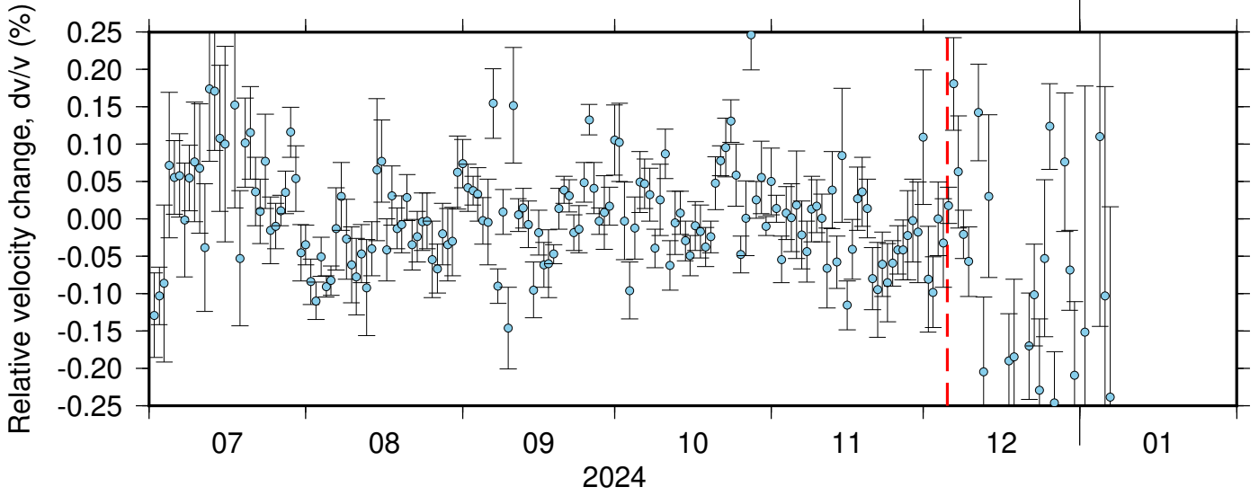
BK_PETL_NC_KMPB ZRT 0.10-0.90Hz 011
