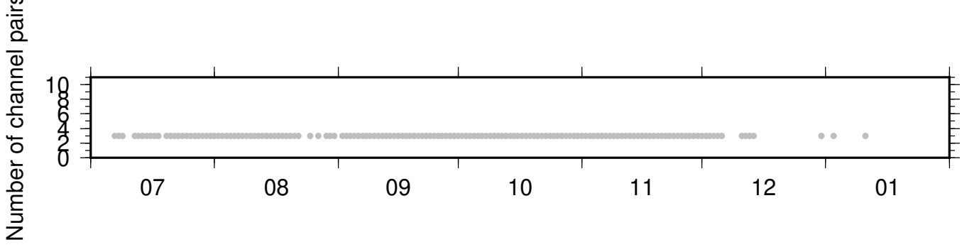
BK_BRIC_NC_KCR ZRT 0.10-0.90Hz 011
