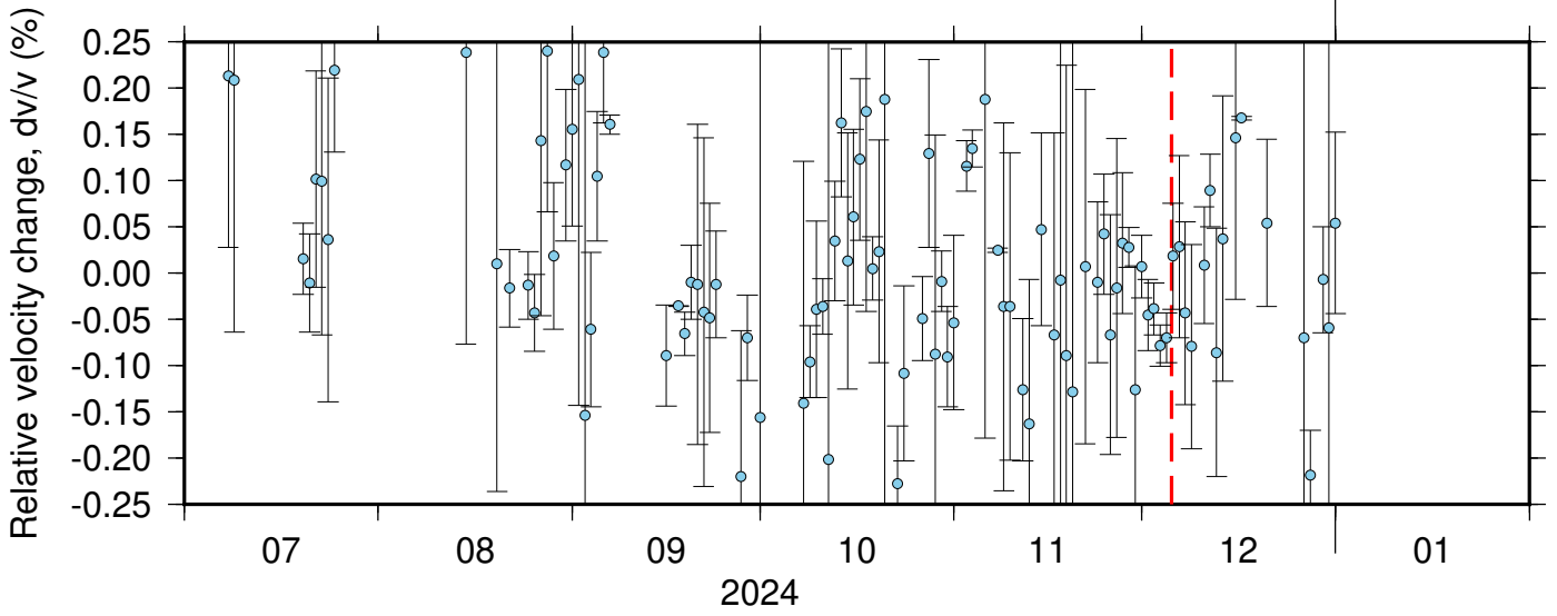
NC_KPR_PB_B935 ZRT 0.10-0.90Hz 011
