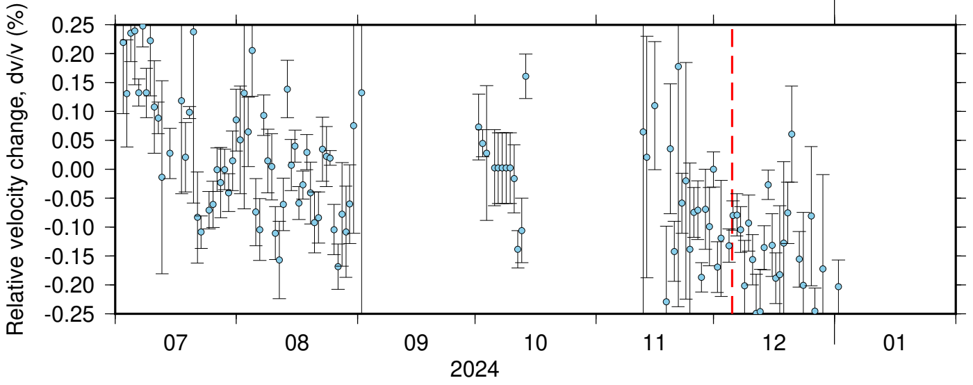
NC_KPR_PB_B046 ZRT 0.10-0.90Hz 011
