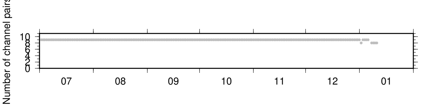
BK_GHOP_BK_PETL ZRT 0.10-0.90Hz 011
