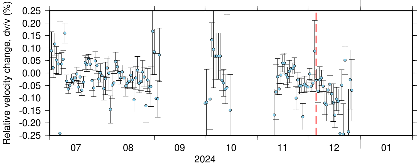
BK_GHOP_PB_B046 ZRT 0.10-0.90Hz 011
