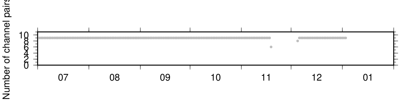
BK_PRDS_PB_B049 ZRT 0.10-0.90Hz 011
