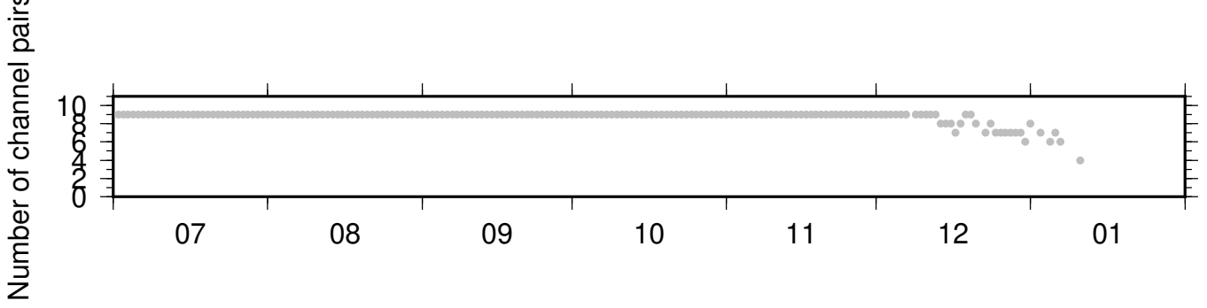
BK_JCC_NC_KCT ZRT 0.10-0.90Hz 011
