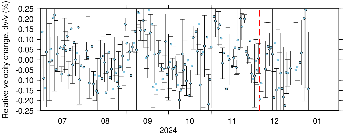
BK_GHOP_BK_JCC ZRT 0.10-0.90Hz 011
