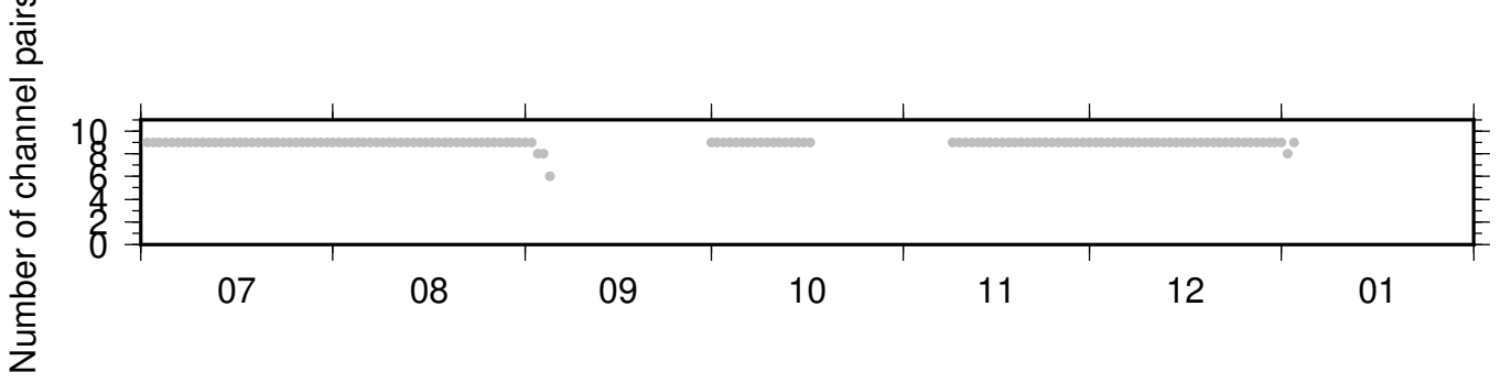
BK_GHOP_PB_B046 ZRT 0.10-0.90Hz 011
