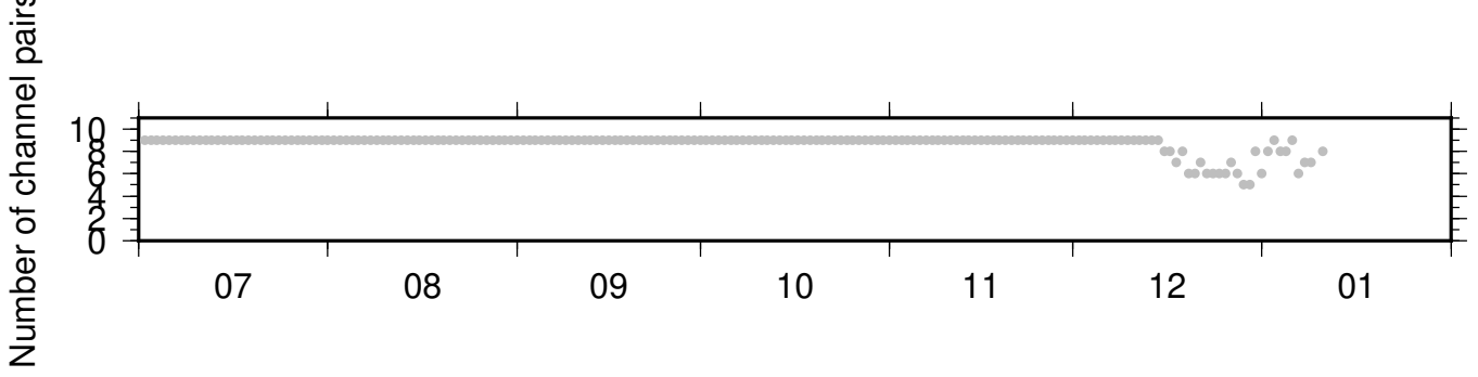
BK_RBOW_NC_KCT ZRT 0.10-0.90Hz 011
