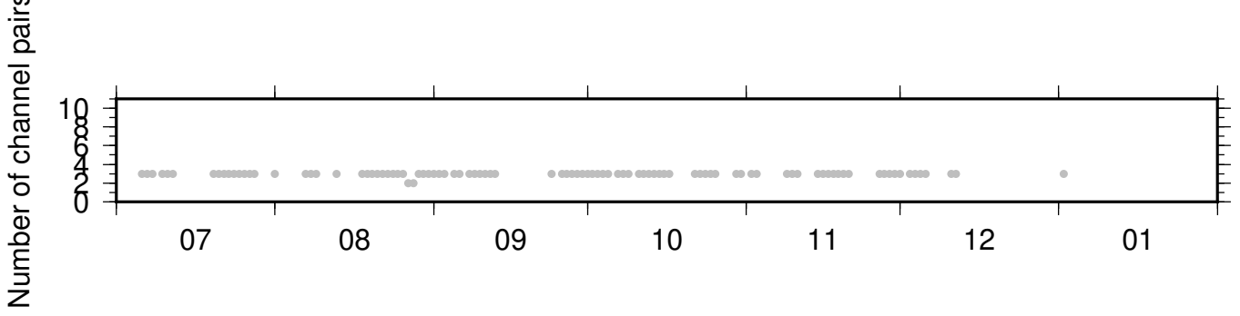
BK_JCC_NC_KBU ZRT 0.10-0.90Hz 011
