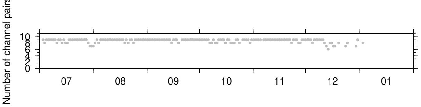
NC_KMPB_PB_B934 ZRT 0.10-0.90Hz 011
