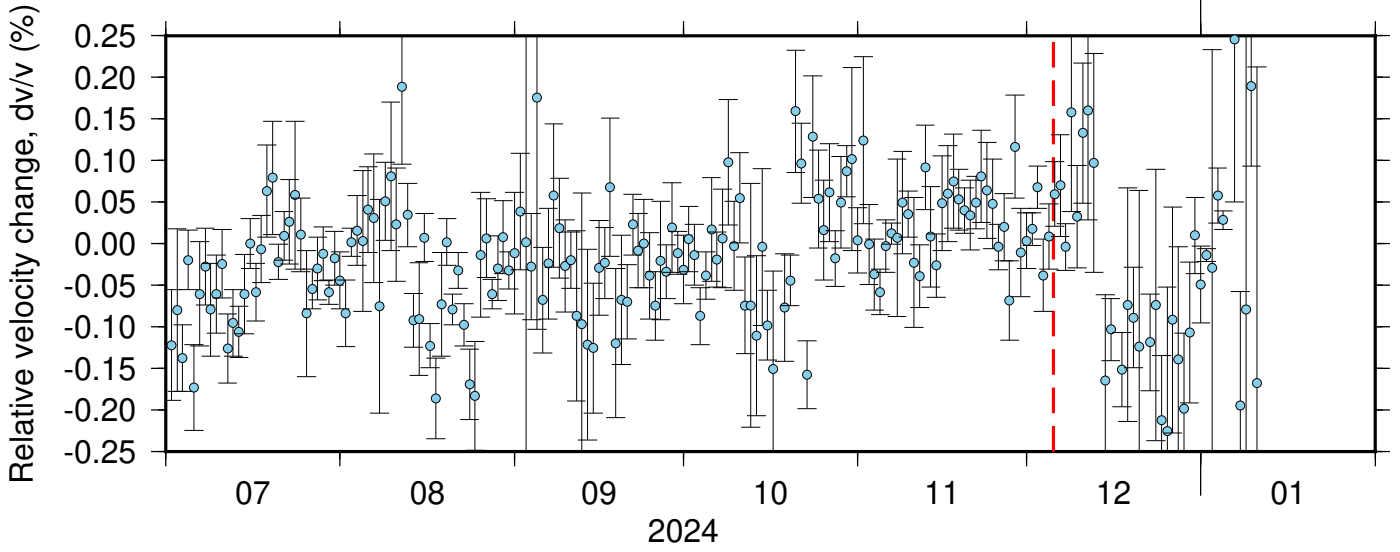
BK_BLAS_BK_SPRL ZRT 0.10-0.90Hz 011
