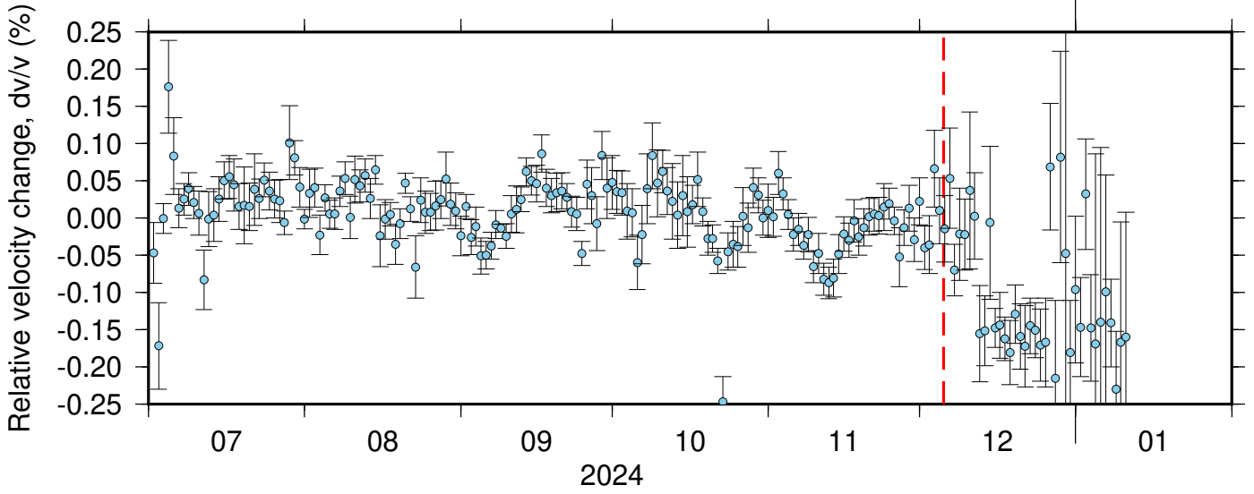
BK_PRDS_BK_RBOW ZRT 0.10-0.90Hz 011
