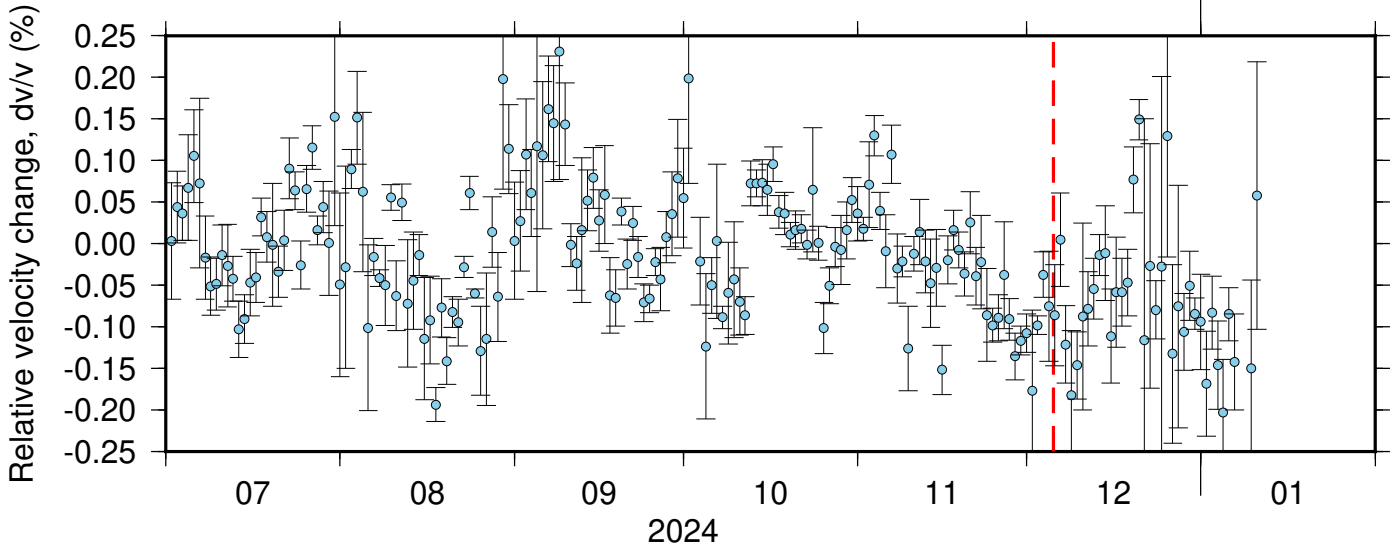
BK_PRDS_NC_KBU ZRT 0.10-0.90Hz 011
