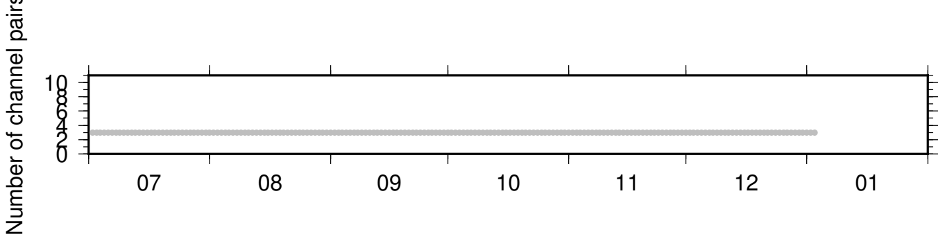
NC_KPR_PB_B047 ZRT 0.10-0.90Hz 011
