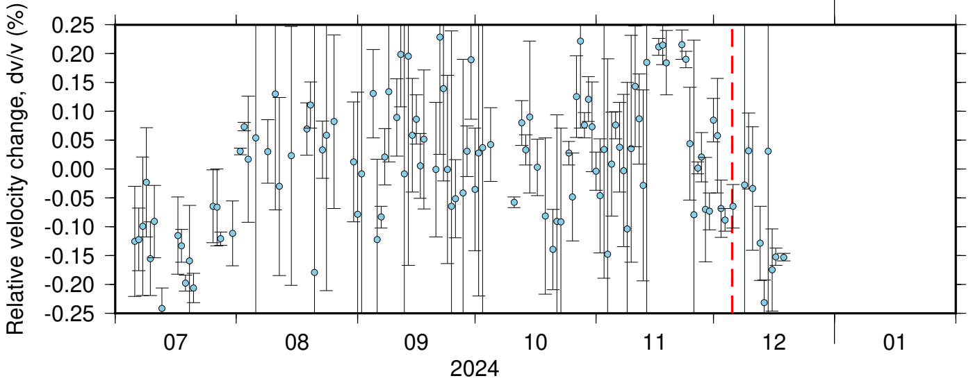
NC_KPR_PB_B934 ZRT 0.10-0.90Hz 011
