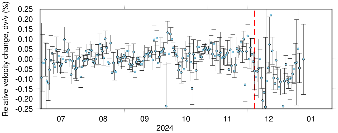
BK_RBOW_NC_KMR ZRT 0.10-0.90Hz 011
