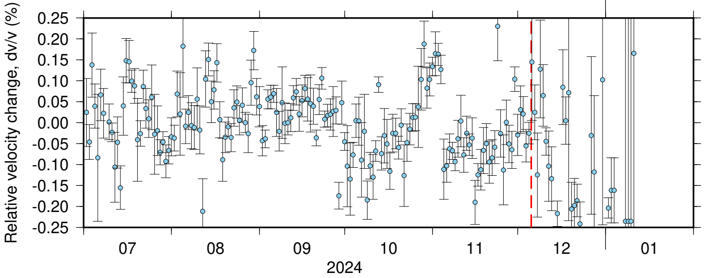
BK_GHOP_BK_PETL ZRT 0.10-0.90Hz 011
