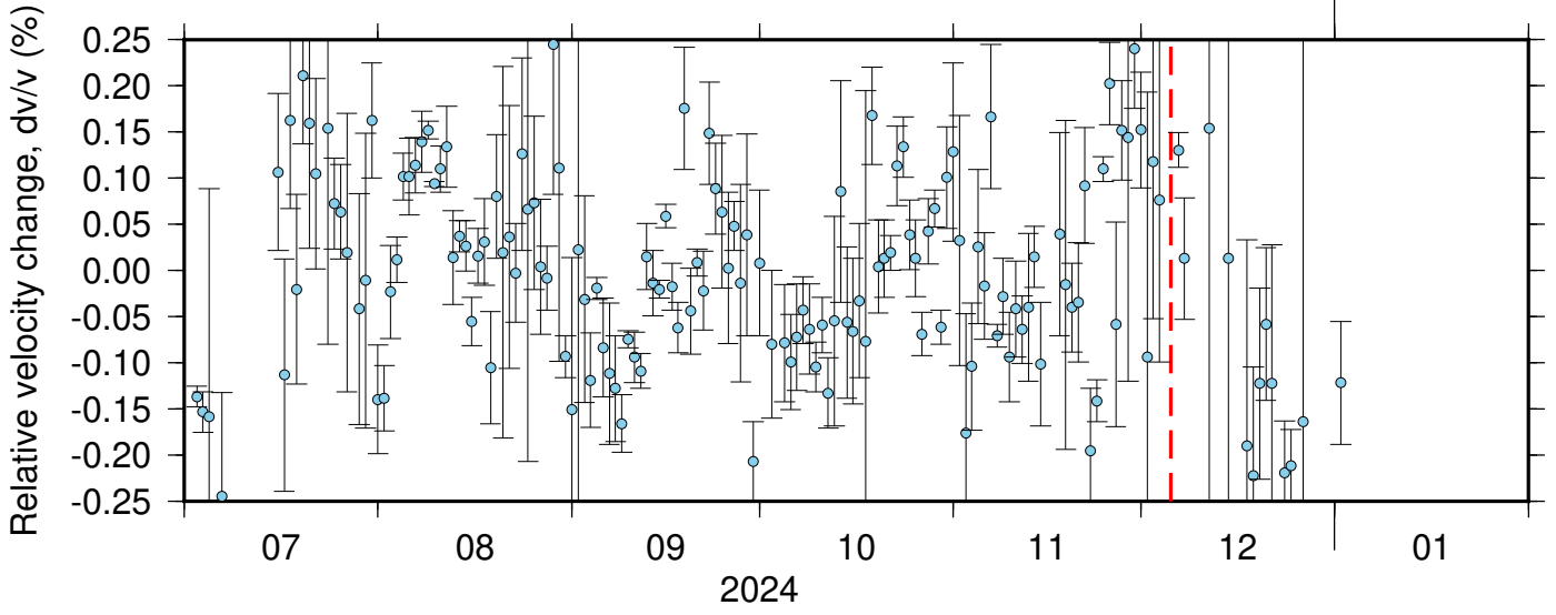
NC_KCR_NC_KMPB ZRT 0.10-0.90Hz 011
