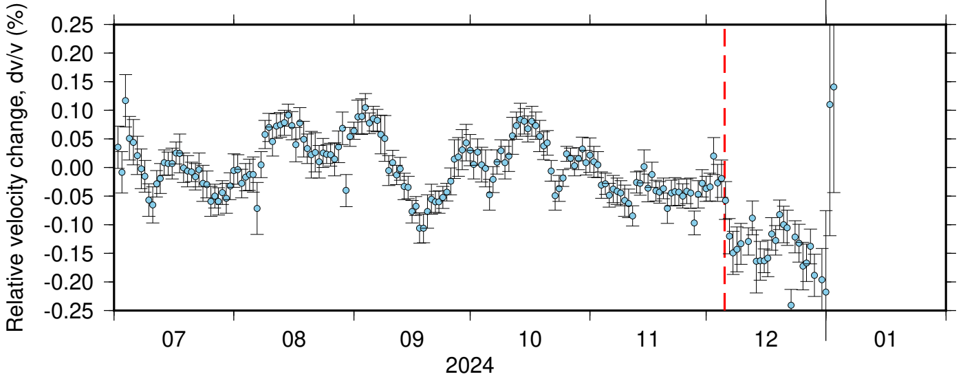
BK_GHOP_PB_B047 ZRT 0.10-0.90Hz 011
