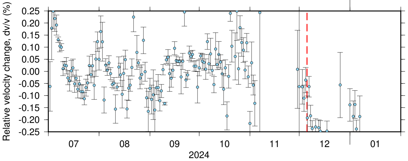
BK_PRDS_NC_KSM ZRT 0.10-0.90Hz 011
