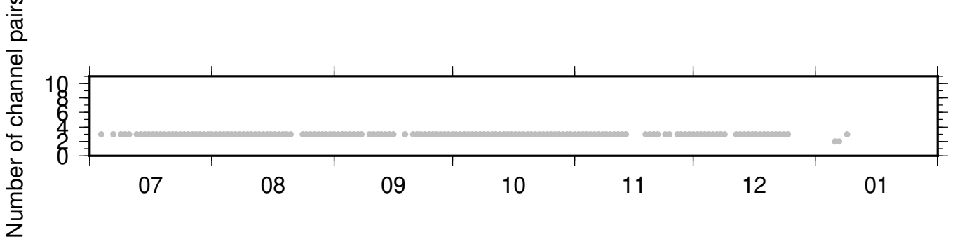
BK_HAYF_NC_KBU ZRT 0.10-0.90Hz 011
