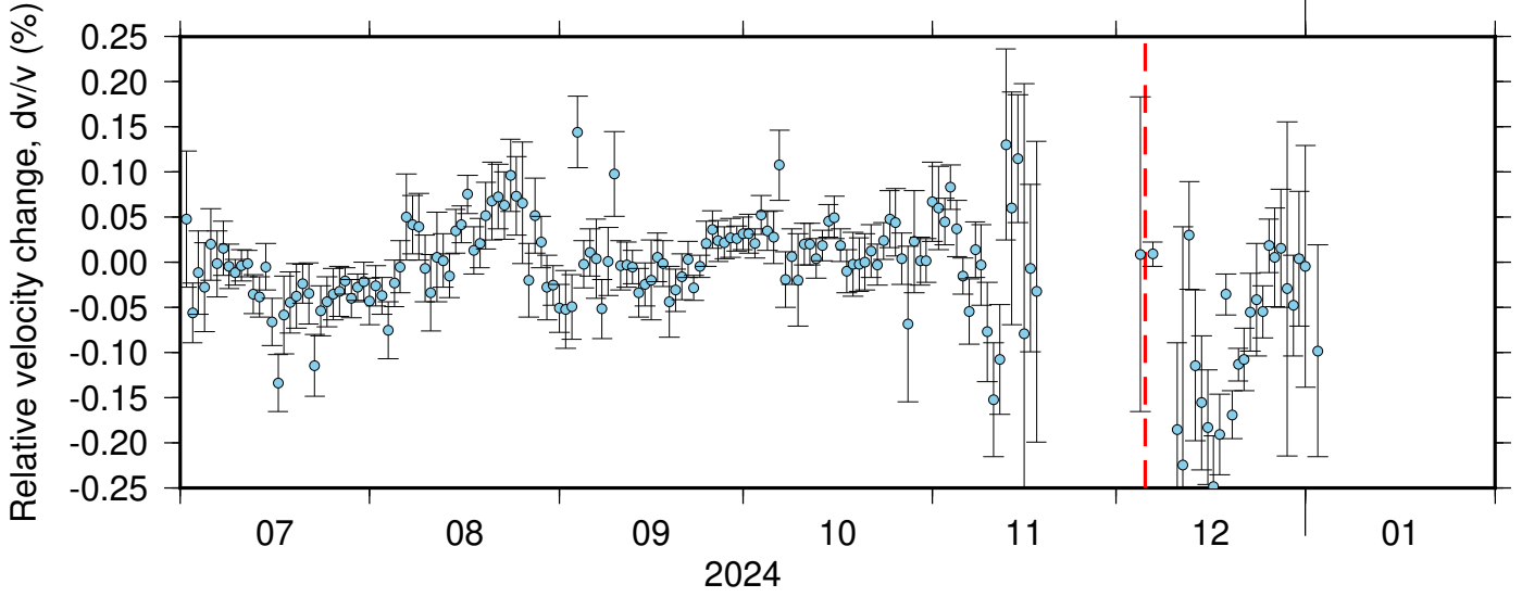
BK_RBOW_PB_B049 ZRT 0.10-0.90Hz 011
