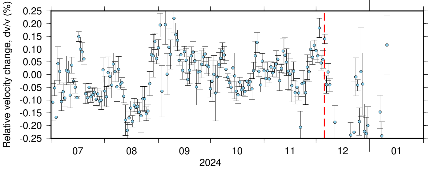
BK_PRDS_NC_KPR ZRT 0.10-0.90Hz 011
