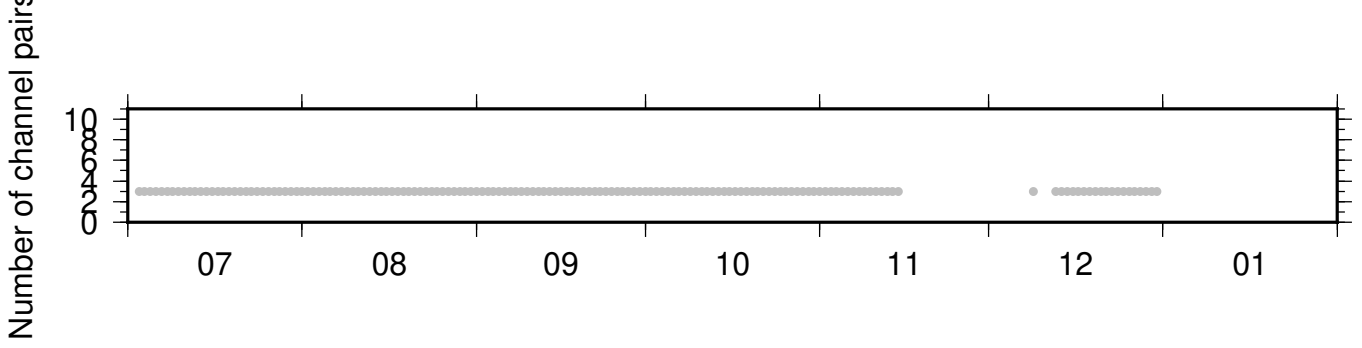
NC_KCR_PB_B049 ZRT 0.10-0.90Hz 011
