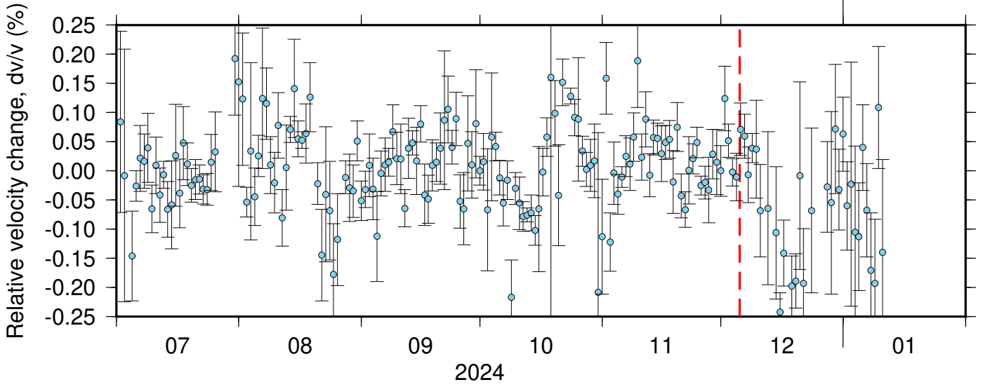
BK_SPRL_NC_KMPB ZRT 0.10-0.90Hz 011
