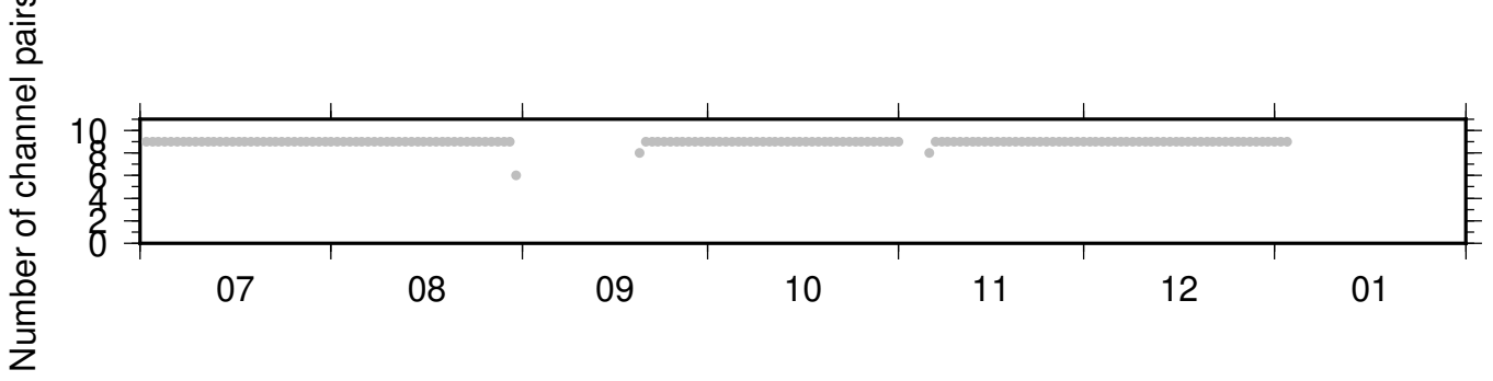
BK_GHOP_PB_B045 ZRT 0.10-0.90Hz 011
