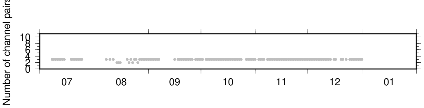
NC_KPR_PB_B935 ZRT 0.10-0.90Hz 011
