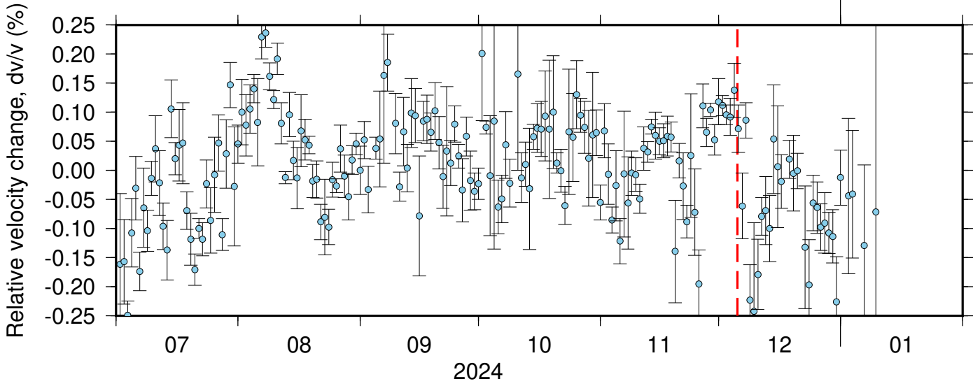
BK_SPRL_NC_KBU ZRT 0.10-0.90Hz 011
