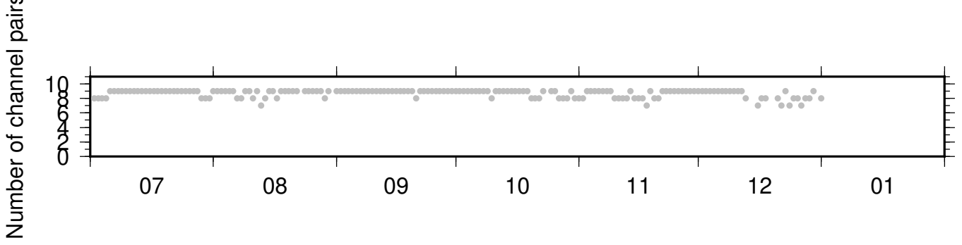
BK_RBOW_PB_B934 ZRT 0.10-0.90Hz 011
