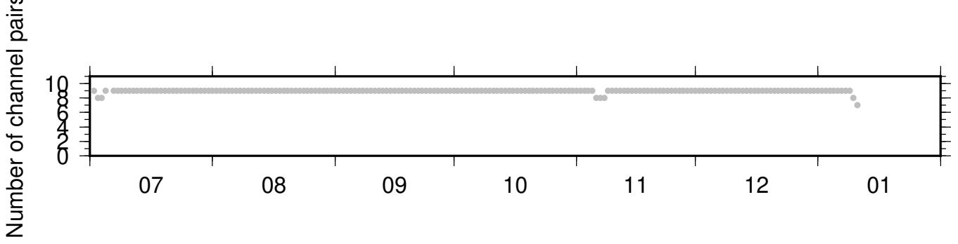
BK_GHOP_BK_JCC ZRT 0.10-0.90Hz 011
