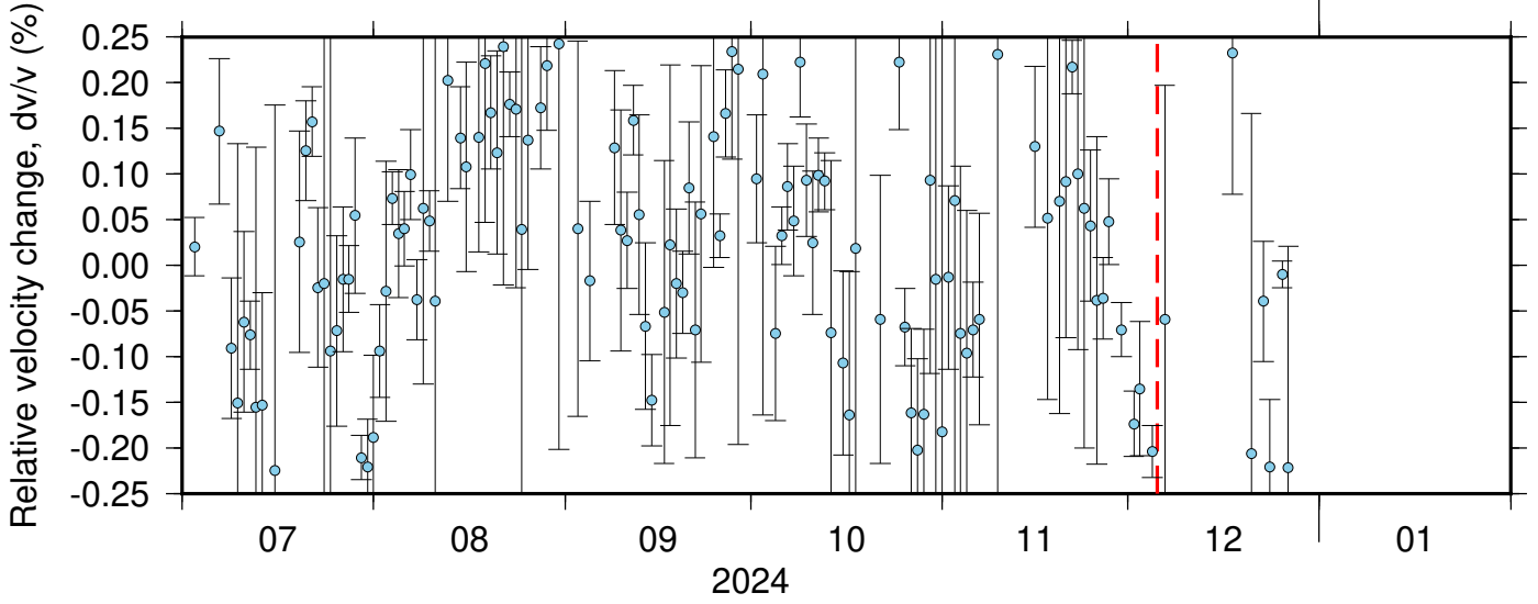
BK_PRDS_NC_KCR ZRT 0.10-0.90Hz 011
