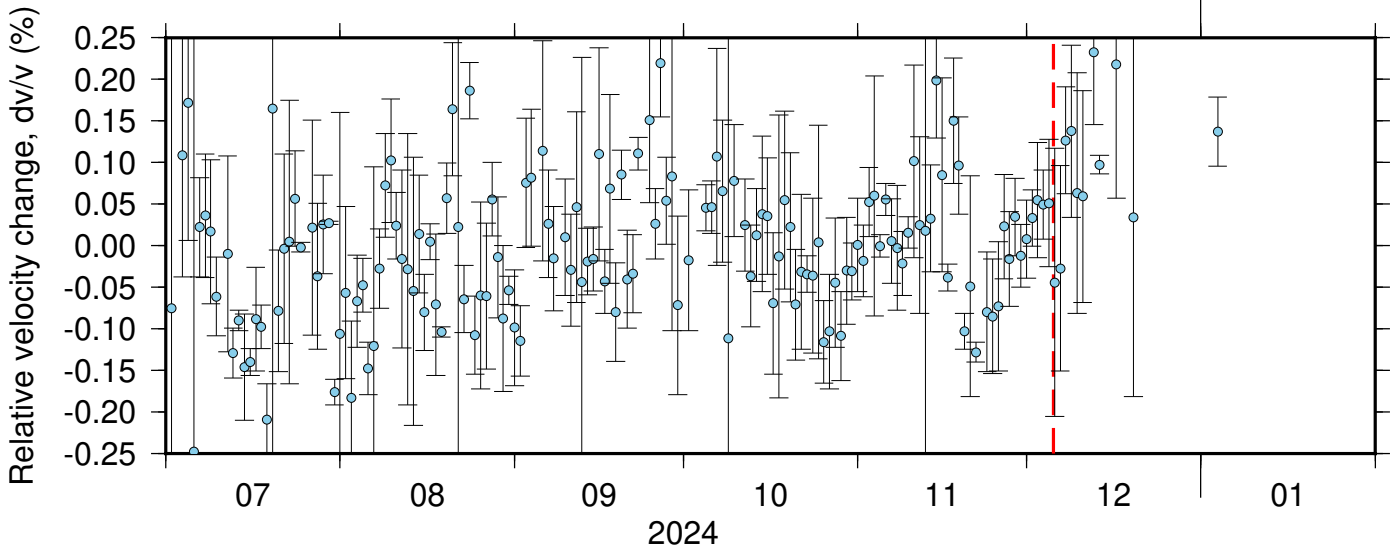
BK_SPRL_NC_KCT ZRT 0.10-0.90Hz 011
