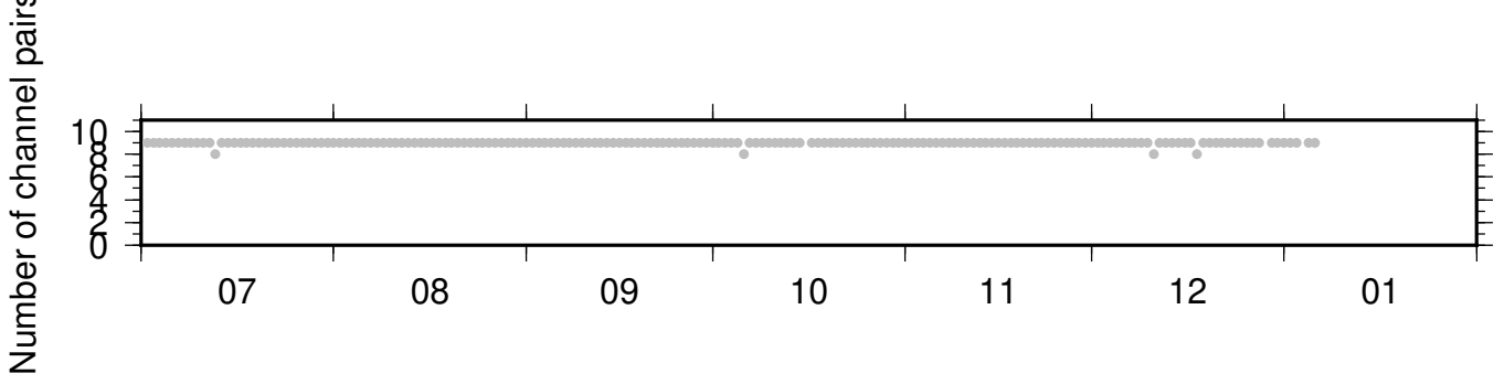
BK_HAYF_NC_KMPB ZRT 0.10-0.90Hz 011
