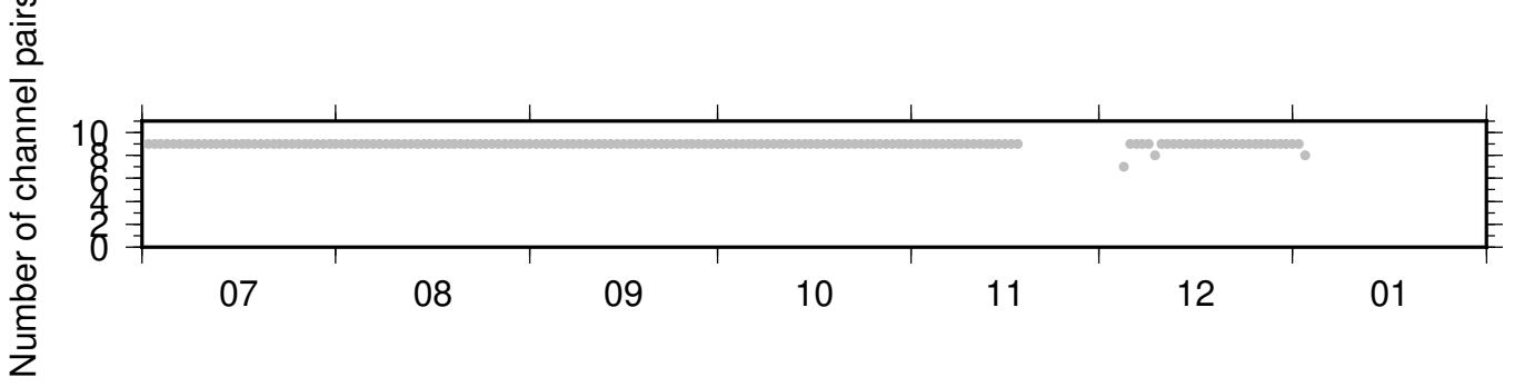
BK_RBOW_PB_B049 ZRT 0.10-0.90Hz 011
