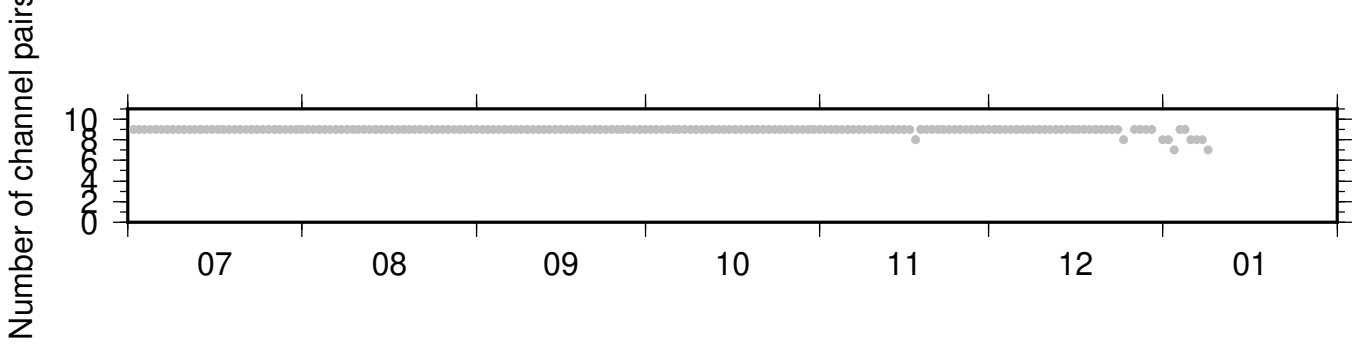
BK_HAYF_BK_SPRL ZRT 0.10-0.90Hz 011
