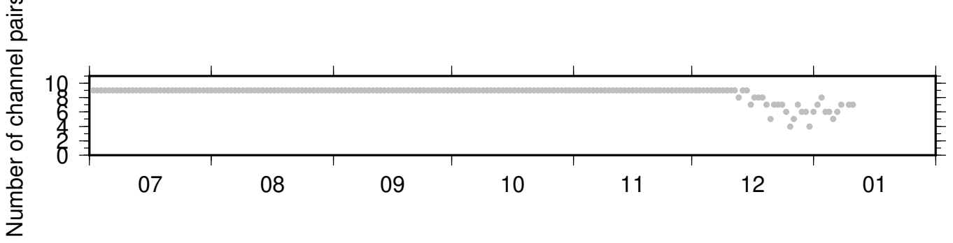
BK_GHOP_NC_KCT ZRT 0.10-0.90Hz 011
