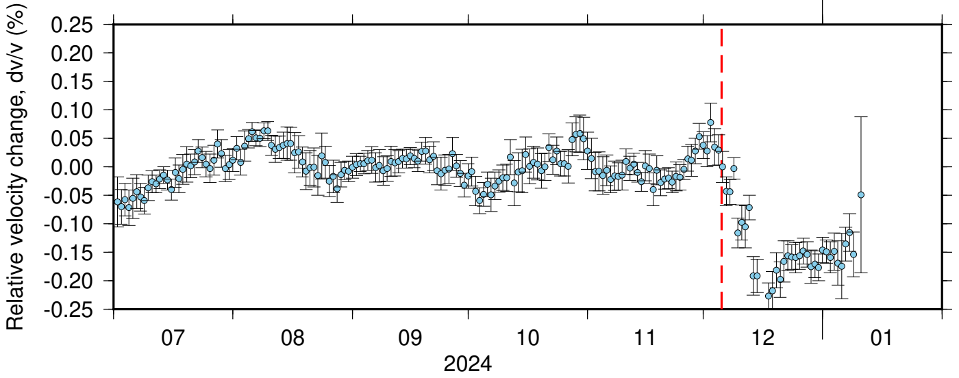
BK_GHOP_BK_RBOW ZRT 0.10-0.90Hz 011
