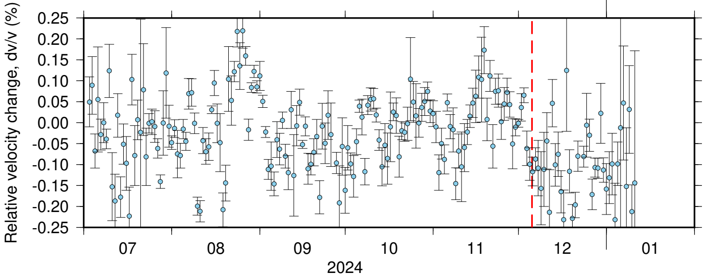
BK_RBOW_NC_KPR ZRT 0.10-0.90Hz 011
