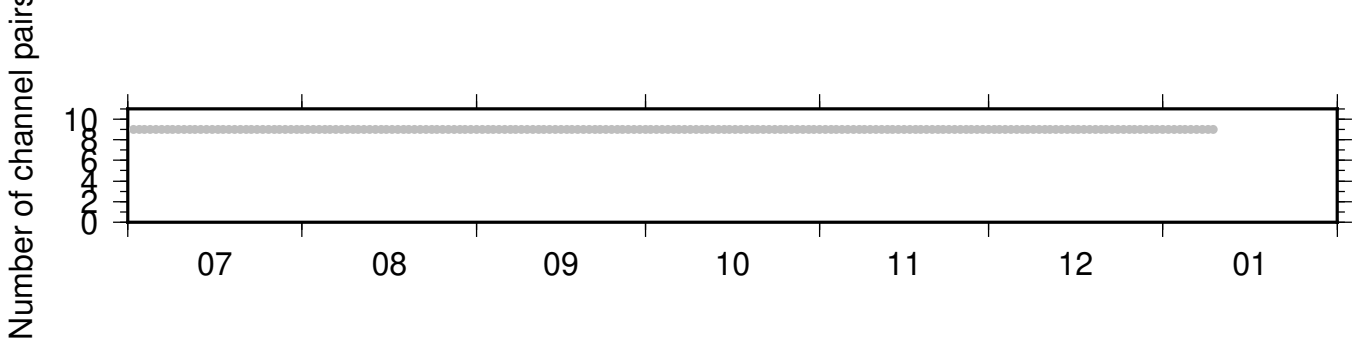
BK_BLAS_NC_KMR ZRT 0.10-0.90Hz 011
