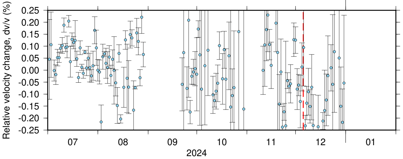
NC_KPR_PB_B045 ZRT 0.10-0.90Hz 011
