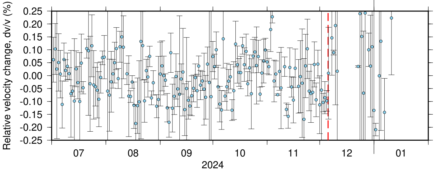
NC_KCT_NC_KMR ZRT 0.10-0.90Hz 011
