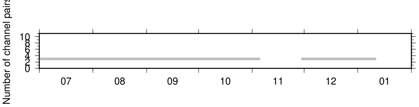
BK_GHOP_NC_KSM ZRT 0.10-0.90Hz 011
