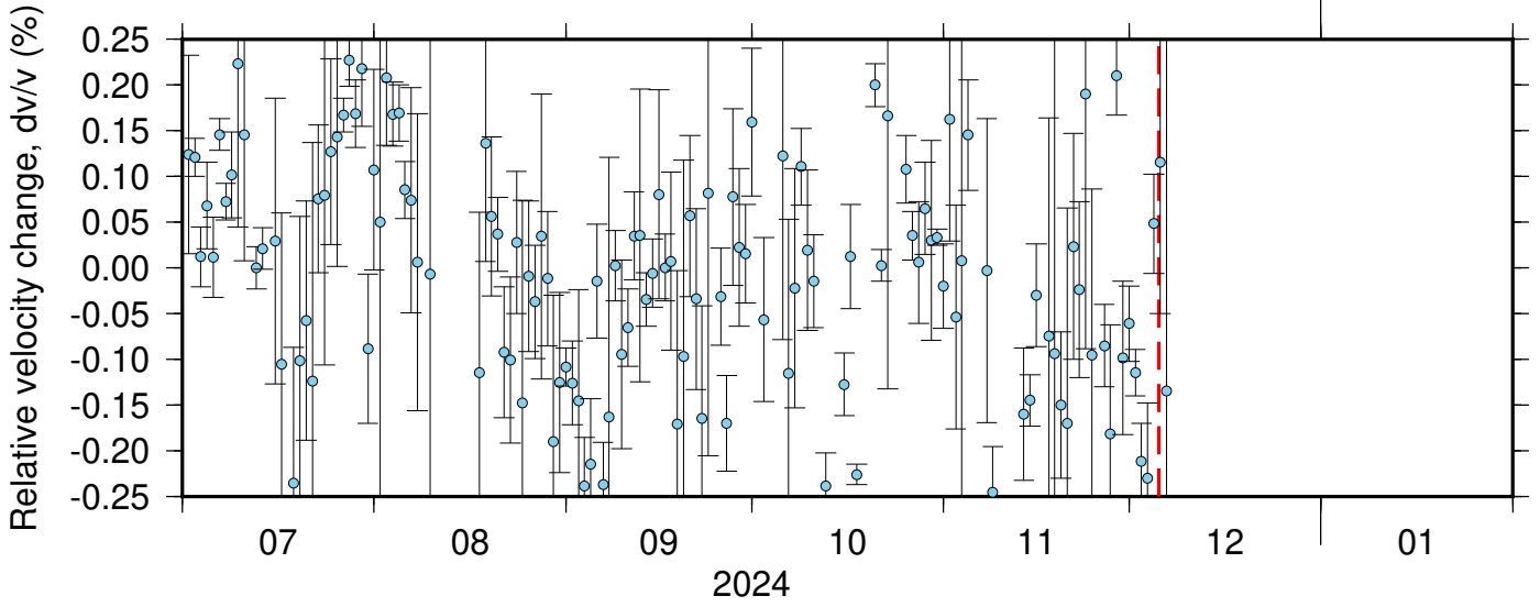
BK_PETL_NC_KBU ZRT 0.10-0.90Hz 011
