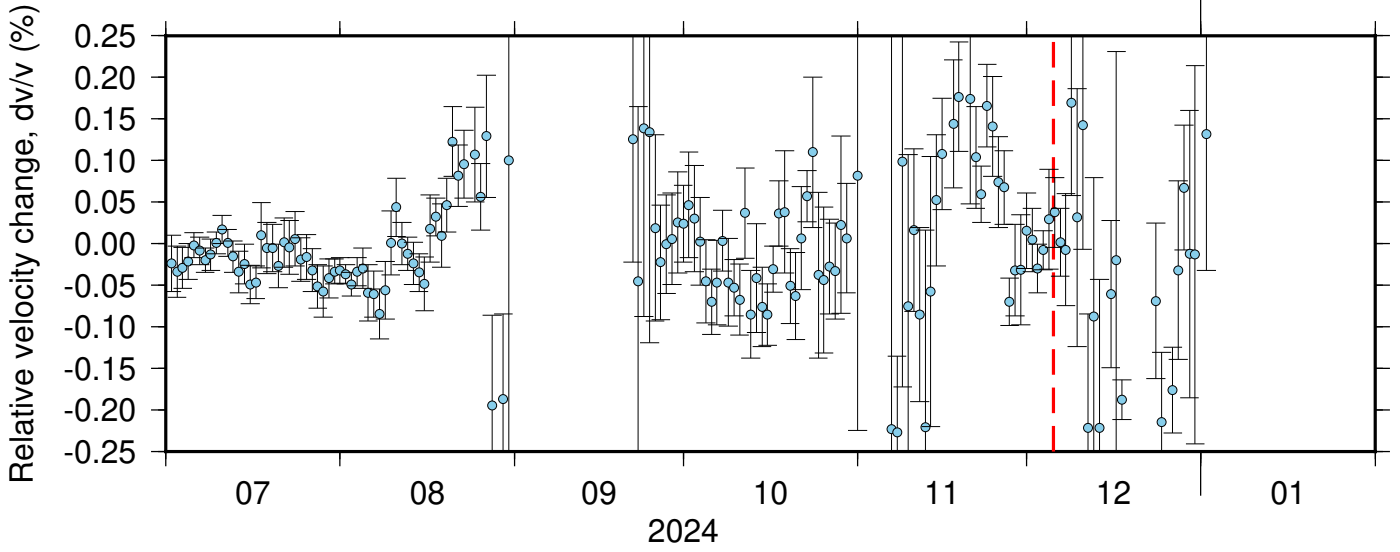
BK_RBOW_PB_B045 ZRT 0.10-0.90Hz 011
