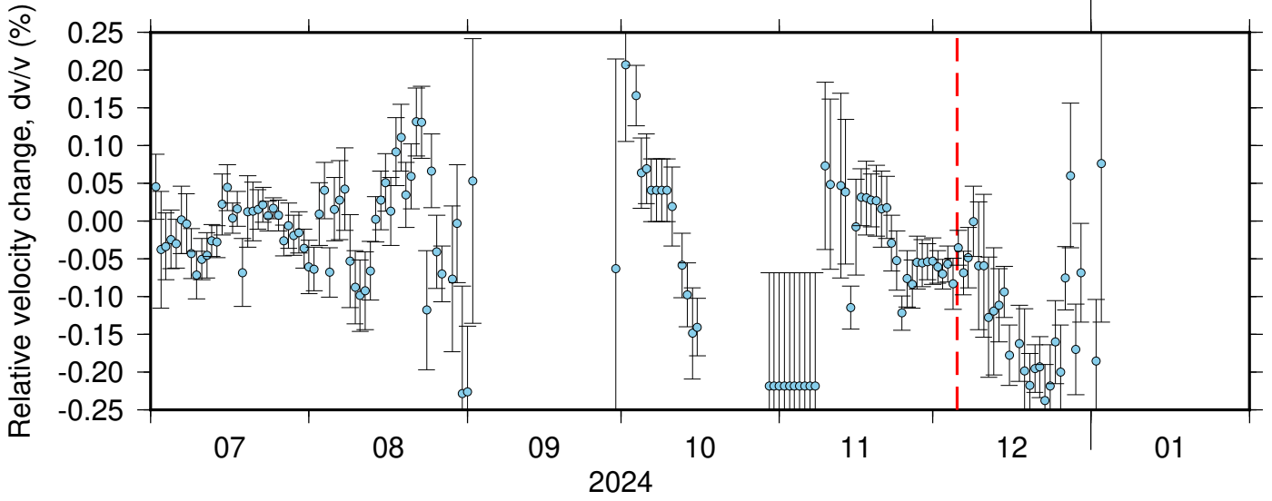
BK_RBOW_PB_B046 ZRT 0.10-0.90Hz 011
