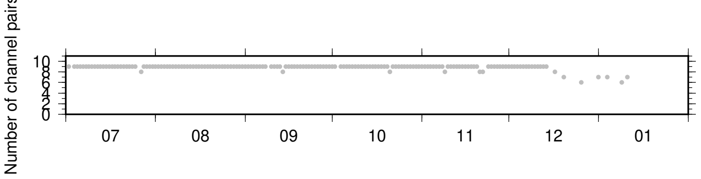
BK_SPRL_NC_KCT ZRT 0.10-0.90Hz 011
