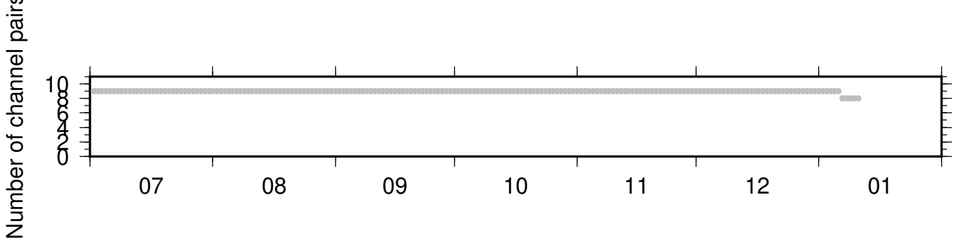
BK_SPRL_NC_KMPB ZRT 0.10-0.90Hz 011
