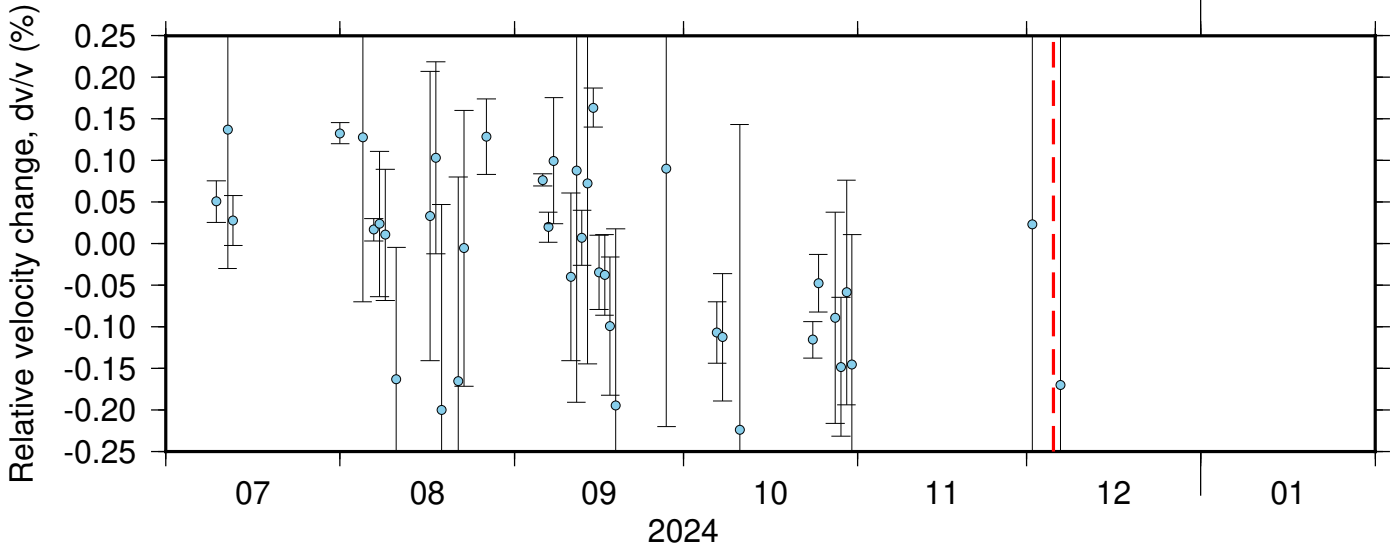
BK_JCC_NC_KSM ZRT 0.10-0.90Hz 011
