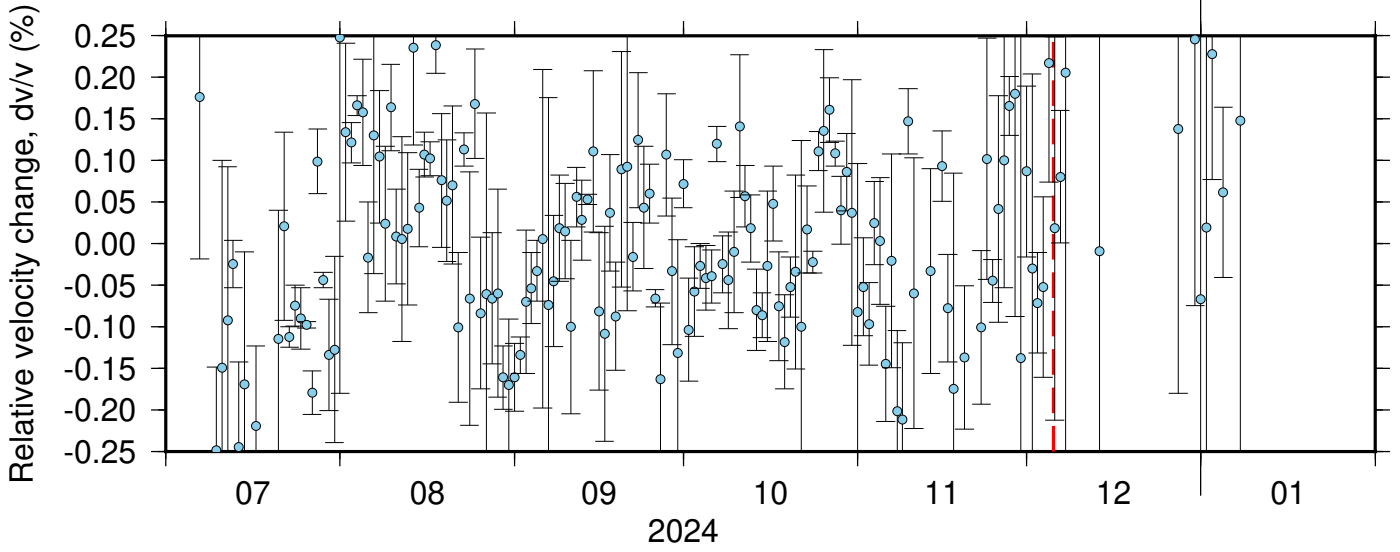
BK_BLAS_NC_KCR ZRT 0.10-0.90Hz 011
