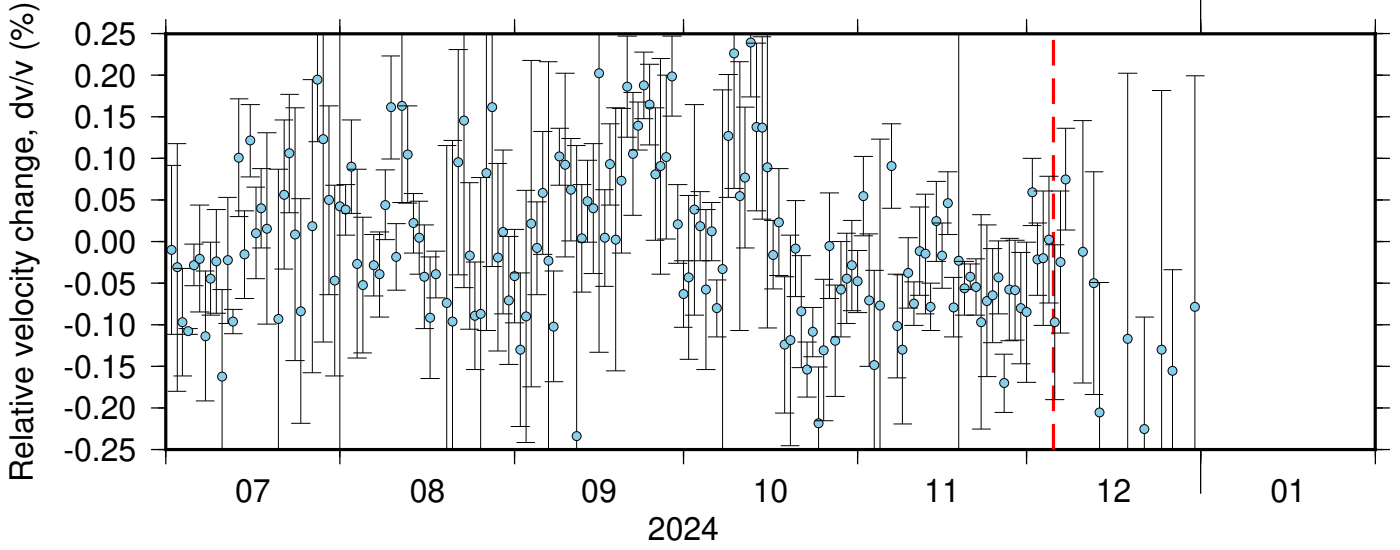
NC_KMPB_PB_B935 ZRT 0.10-0.90Hz 011
