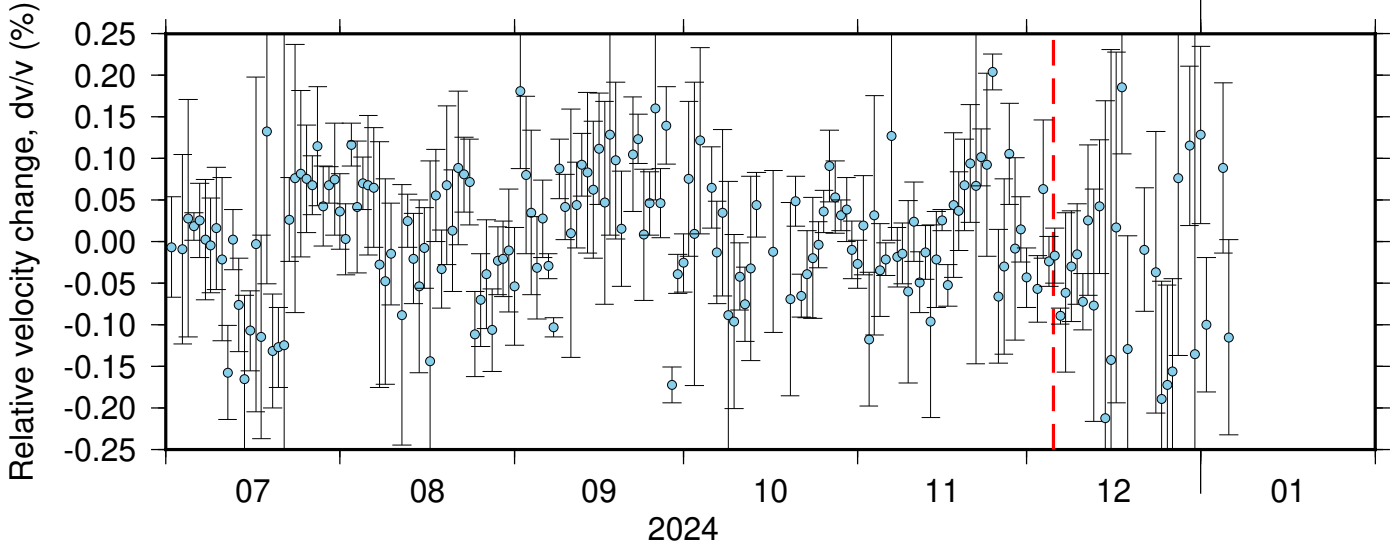
BK_HAYF_NC_KMPB ZRT 0.10-0.90Hz 011
