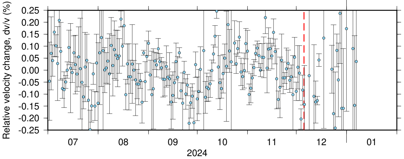
BK_JCC_NC_KCT ZRT 0.10-0.90Hz 011
