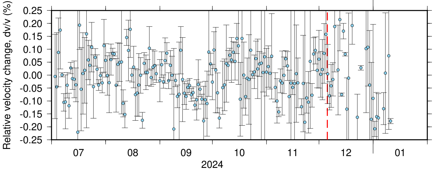
BK_GHOP_BK_HAYF ZRT 0.10-0.90Hz 011
