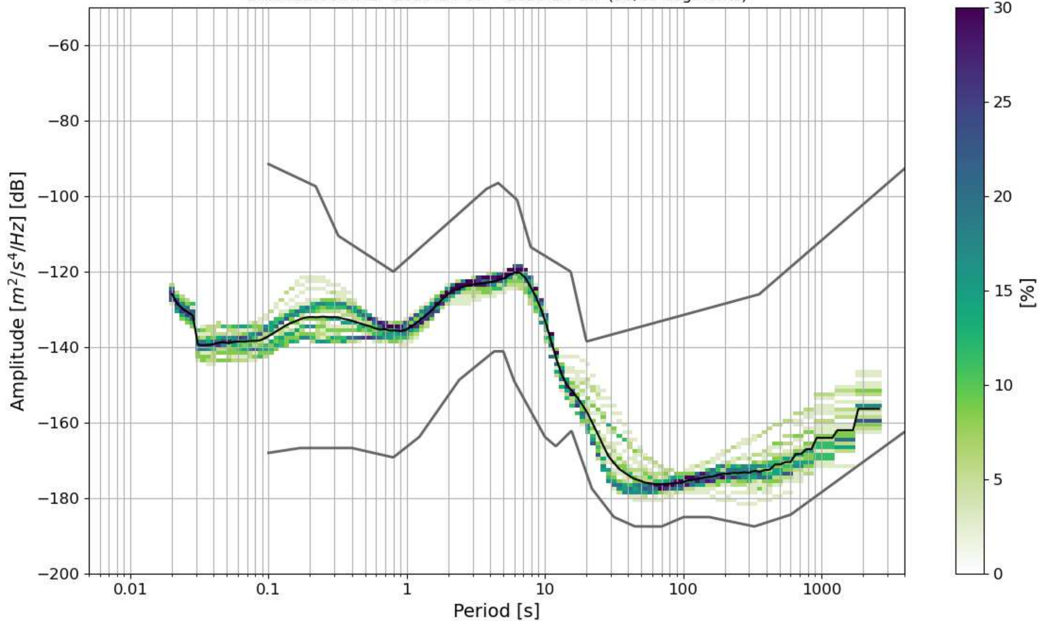
BK.BK02.00.HHZ 2025-04-08 -- 2025-04-10 (35/35 segments)
