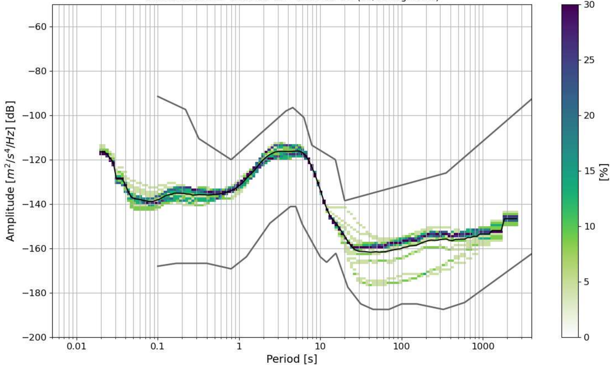
BK.BK30.00.HHZ 2025-03-15 -- 2025-03-16 (23/23 segments)
