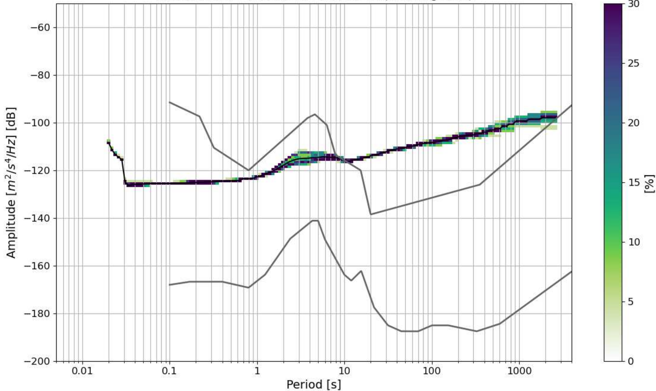
BK.BK02.00.HNZ 2025-03-15 -- 2025-03-16 (23/23 segments)
