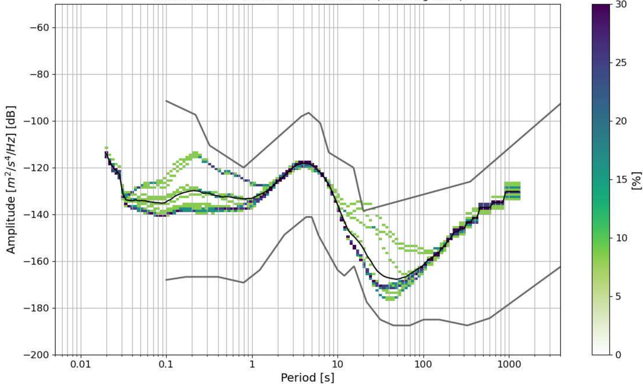
BK.BK84.01.HHZ 2025-03-12 -- 2025-03-12 (12/12 segments)
