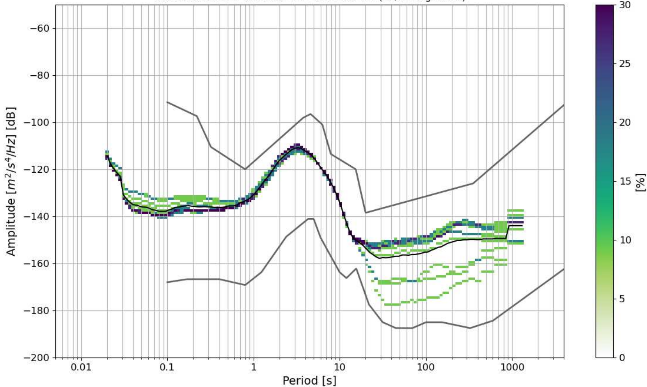
BK.BK30.00.HHZ 2025-03-13 -- 2025-03-13 (11/11 segments)
