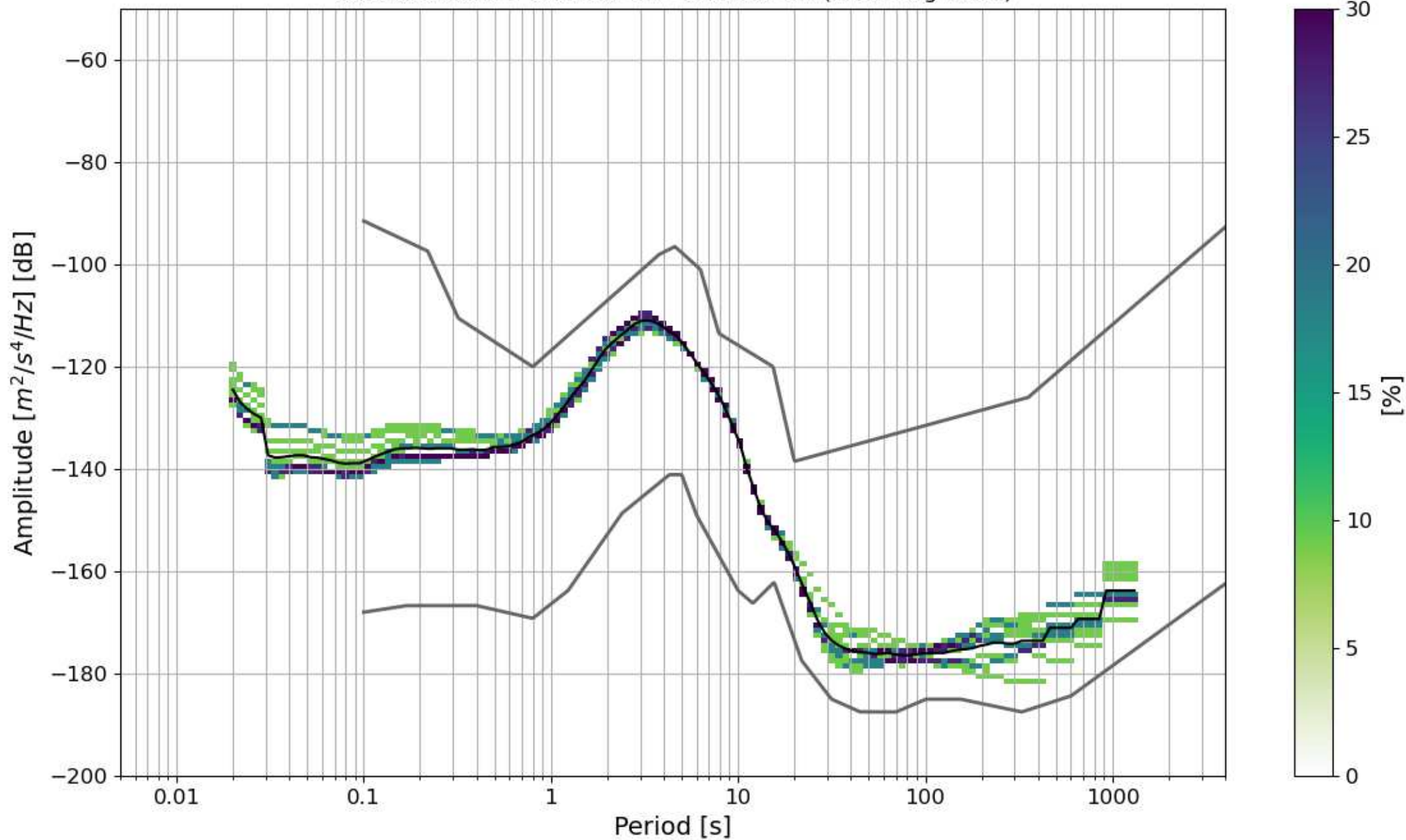
BK.BK02.00.HHZ 2025-03-13 -- 2025-03-13 (11/11 segments)
