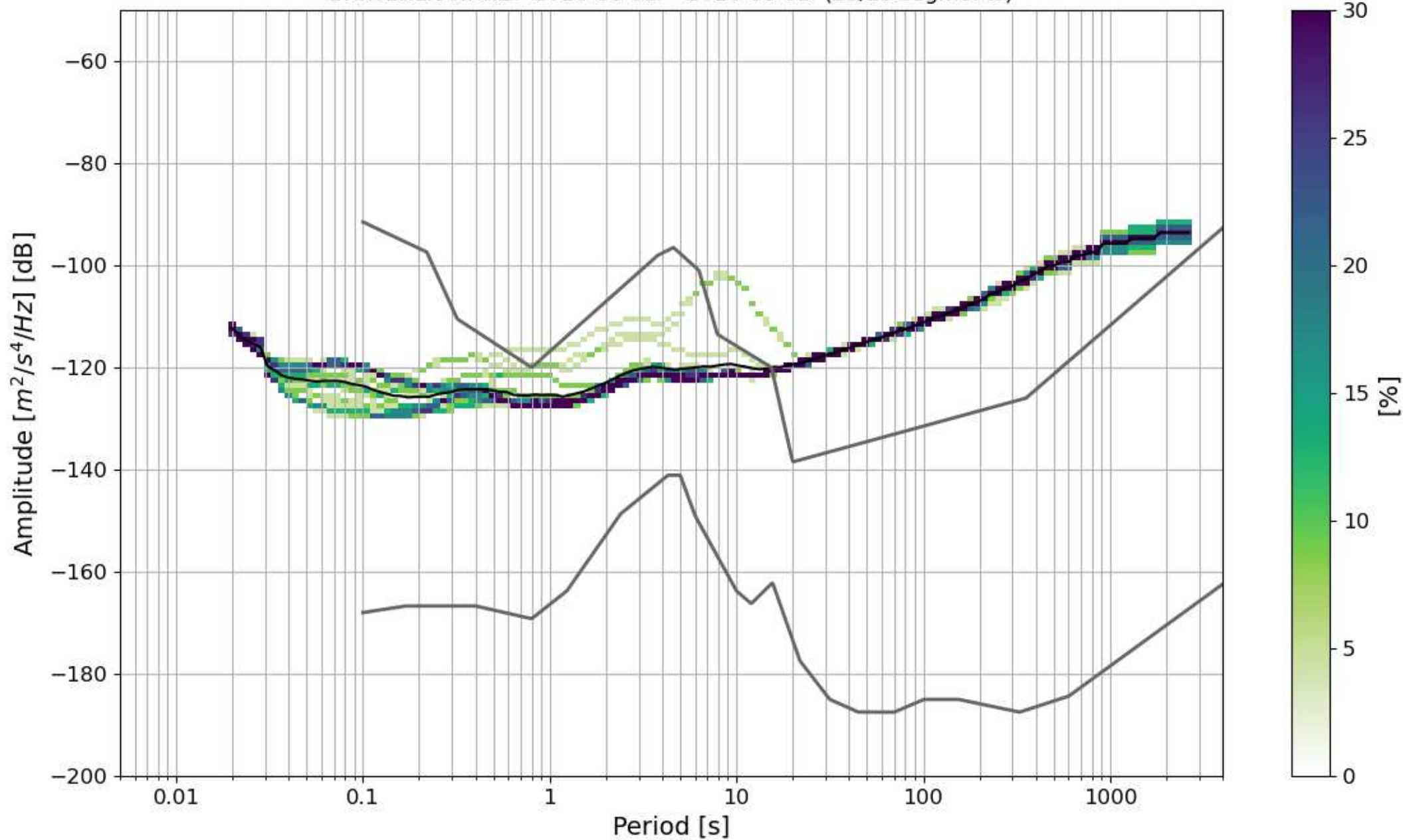
BK.WENL.00.HNZ 2026-06-02 -- 2026-06-03 (23/23 segments)
